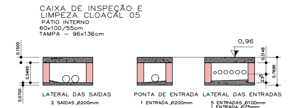
DETALHE 03 CAIXAS DE INSPEÇÃO ESC. - 1:50
