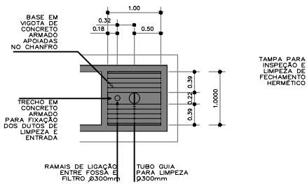
DETALHE 05 PLANTA BAIXA PARCIAL FUNDO FALSO DO FILTRO ANAERÓBIO ESC. - 1:50
