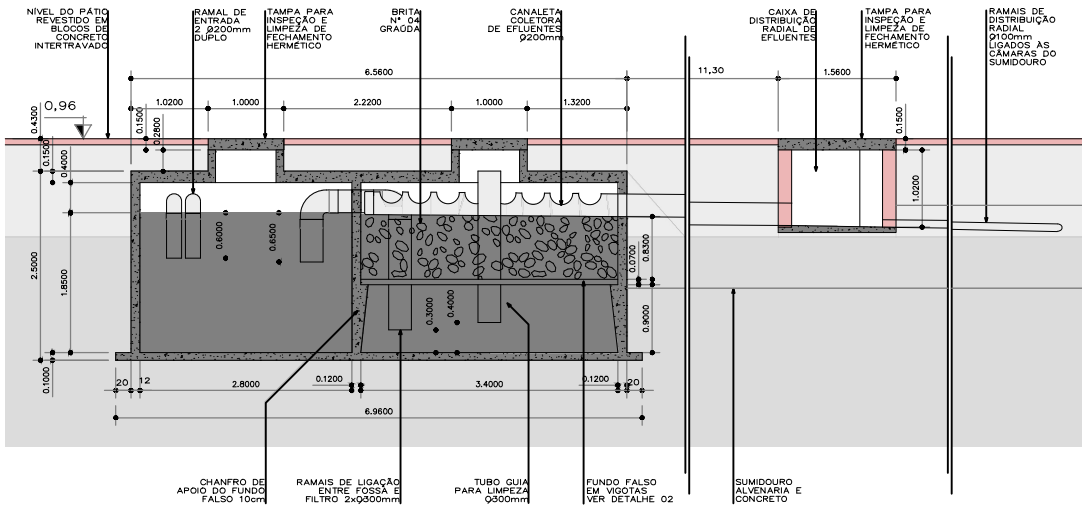
DETALHE 01 CORTE DO SISTEMA DE TRATAMENTO DE ESGOTOS FOSSA SÉPTICA, FILTRO ANAERÓBIO E SUMIDOURO SANITÁRIOS BLOCOS 02 E 04 ESC. - 1:50
