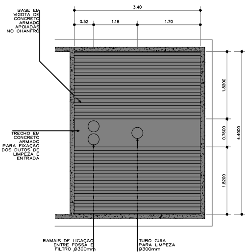
DETALHE 02 PLANTA BAIXA PARCIAL FUNDO FALSO DO FILTRO ANAERÓBIO ESC. - 1:50
