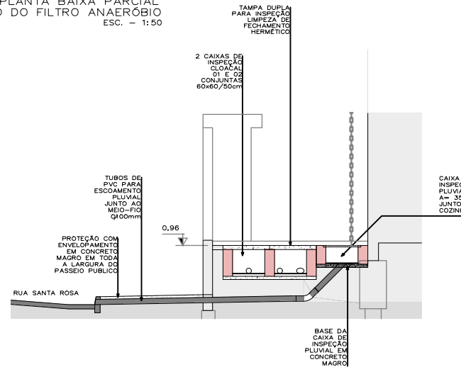
DETALHE 06 CORTE CAIXAS DE INSPEÇÃO CLOACAL E PLUVIAL ESC. - 1:50
