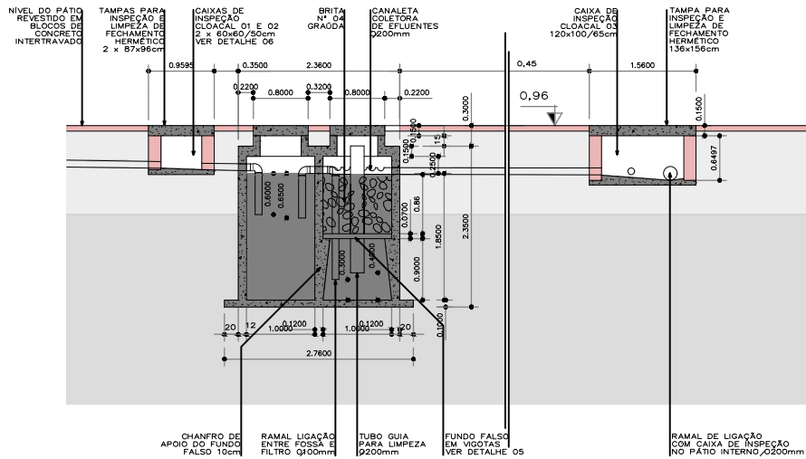
DETALHE 04 CORTE DO SISTEMA DE TRATAMENTO DE ESGOTOS FOSSA SÉPTICA, FILTRO ANAERÓBIO E SUMIDOURO SANITÁRIO, COZINHA E LAVANDERIA DO SERVIÇO ESC. - 1:50
