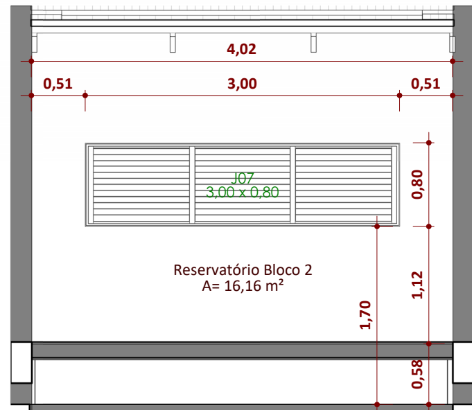
Elevação 1 - a ESCALA 1:50
