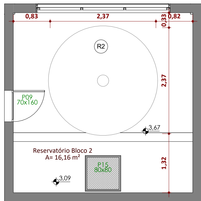
Ampliação Reservatório Bloco 2 ESCALA 1:50
