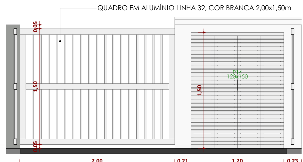
Elevação 4 - c ESCALA 1:25
