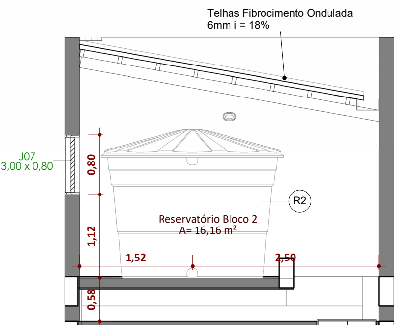
Elevação 1 - b ESCALA 1:50
