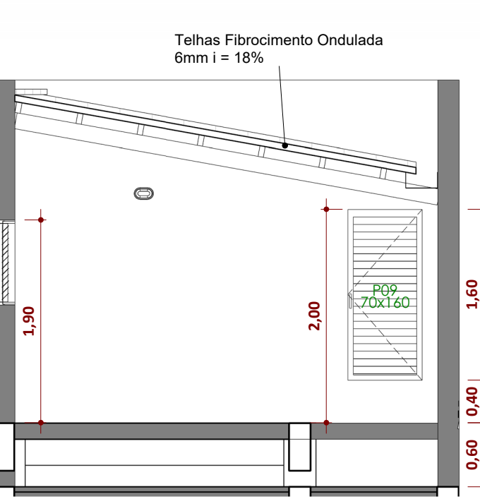
Elevação 3 - d ESCALA 1:50
