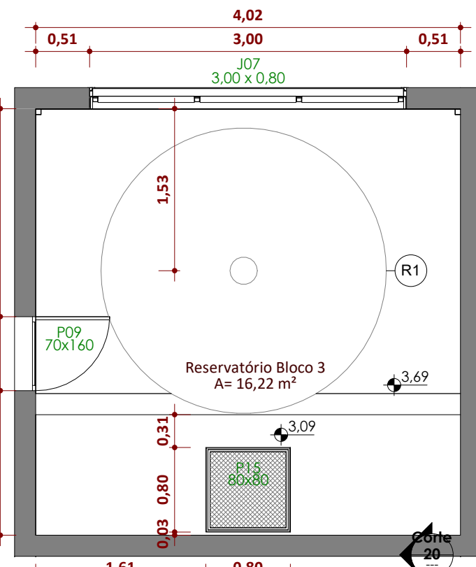
Ampliação Reservatório Bloco 3 ESCALA 1:50
