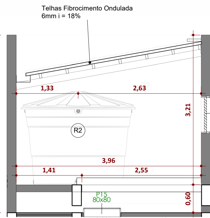
Elevação 3 - b ESCALA 1:50
