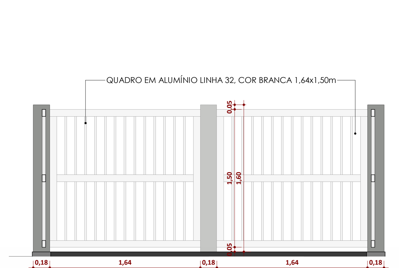
Elevação 4 - a ESCALA 1:25
