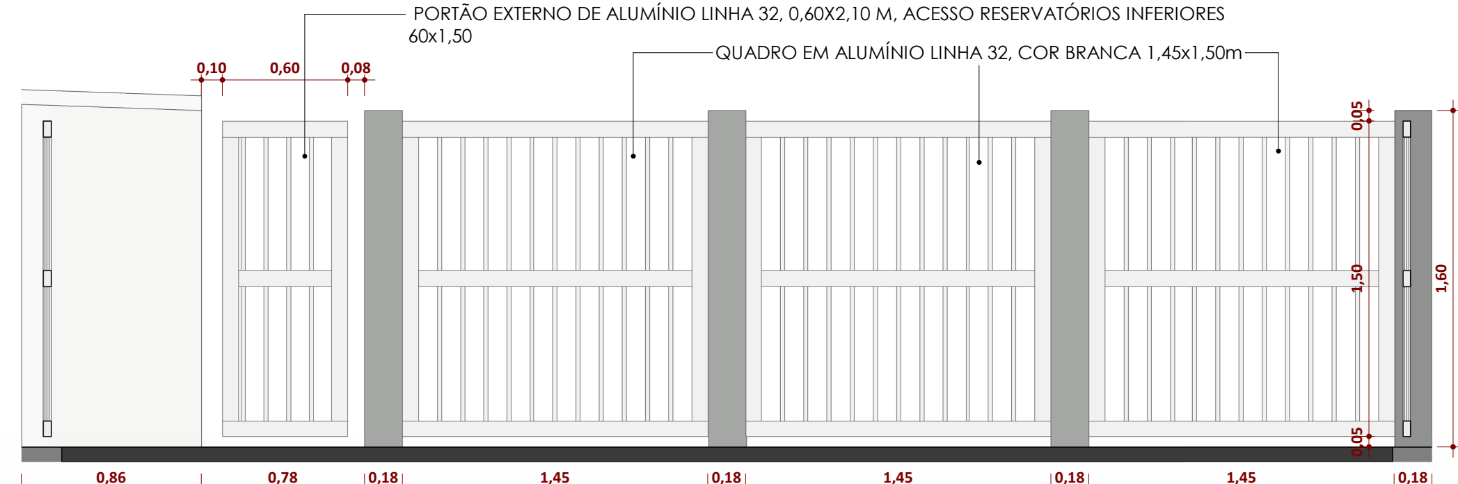
Elevação 4 - b ESCALA 1:25
