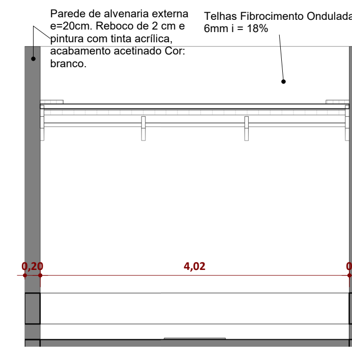
Elevação 2 - c ESCALA 1:50
