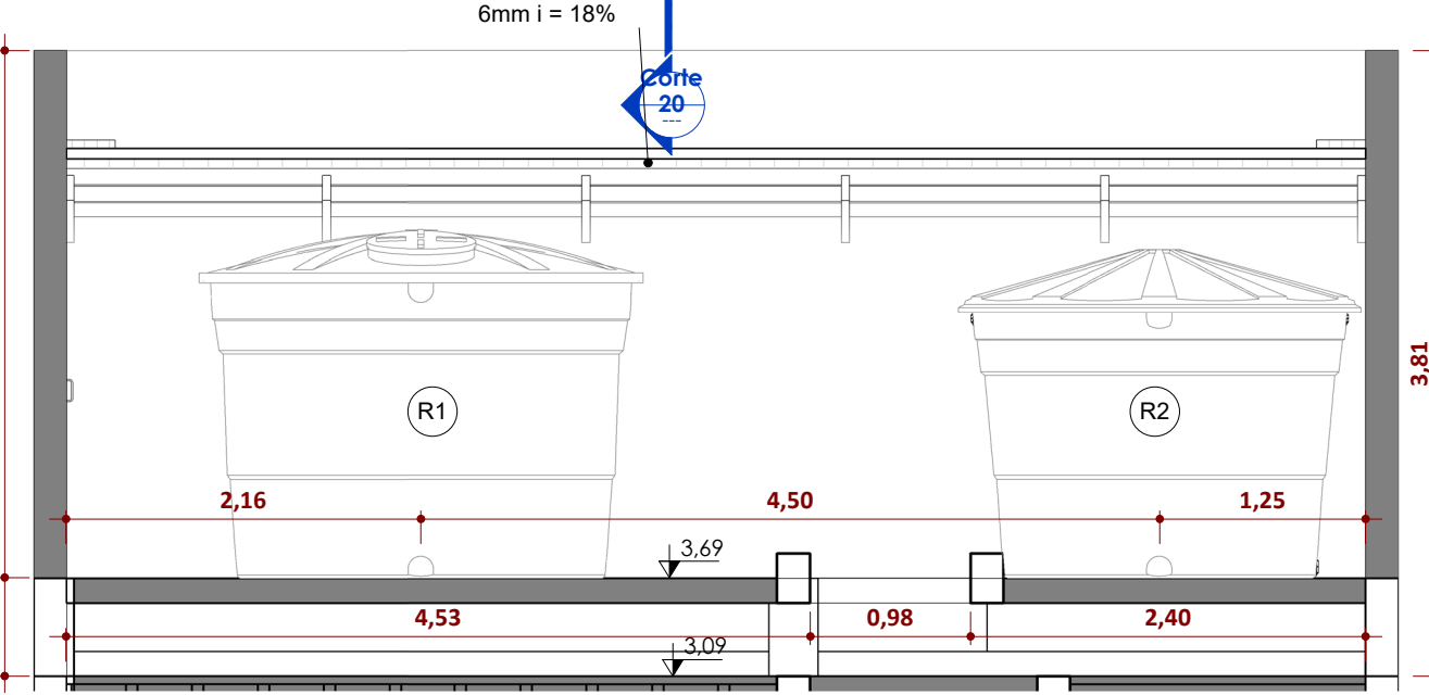
Elevação 3 - a ESCALA 1:50
