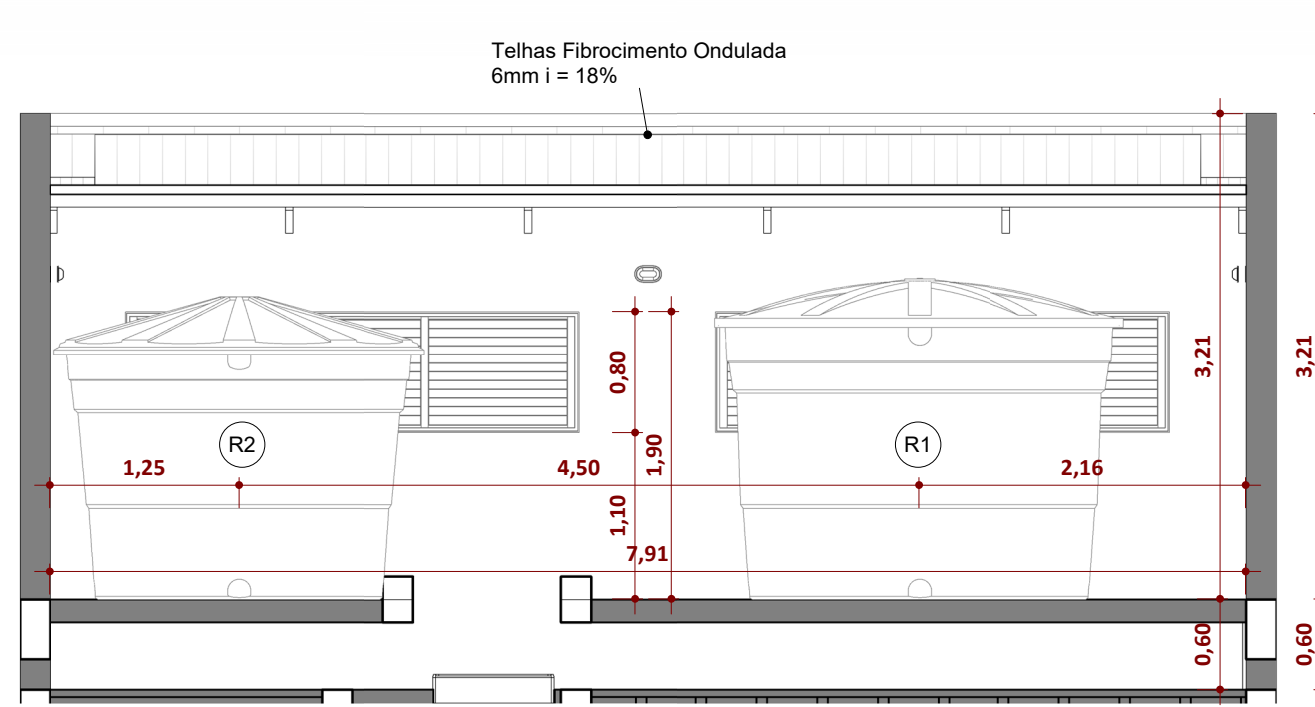
Elevação 3 - c ESCALA 1:50
