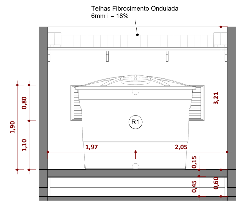
Elevação 2 - a ESCALA 1:50
