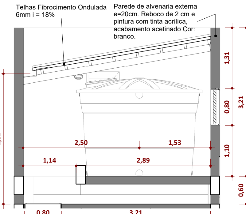
Elevação 2 - d ESCALA 1:50
