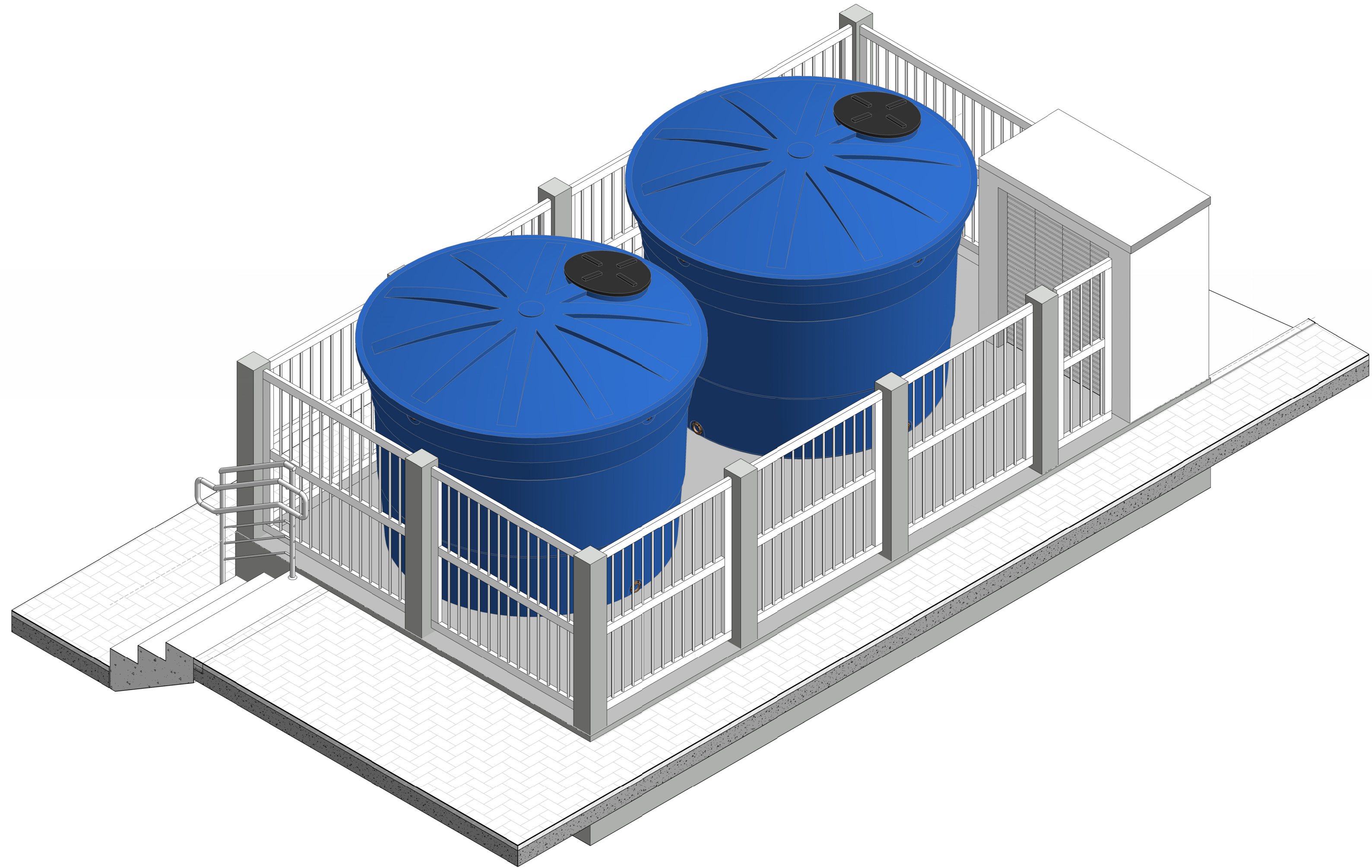
Reservatório Externo - Bloco 5 - Perspectiva ESCALA 1:25
