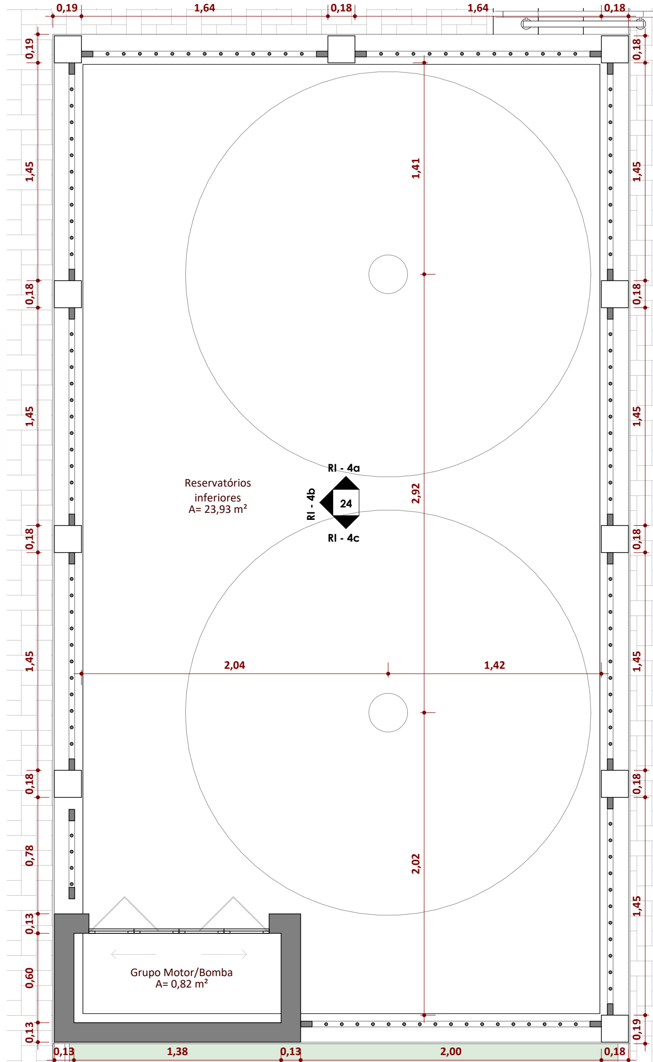
Ampliação Reservatório Externo - Bloco 5 ESCALA 1:25
