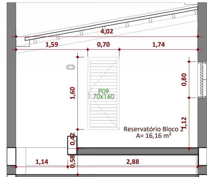
Elevação 1 - d ESCALA 1:50
