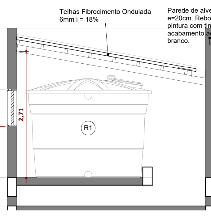
Elevação 2 - b ESCALA 1:50
