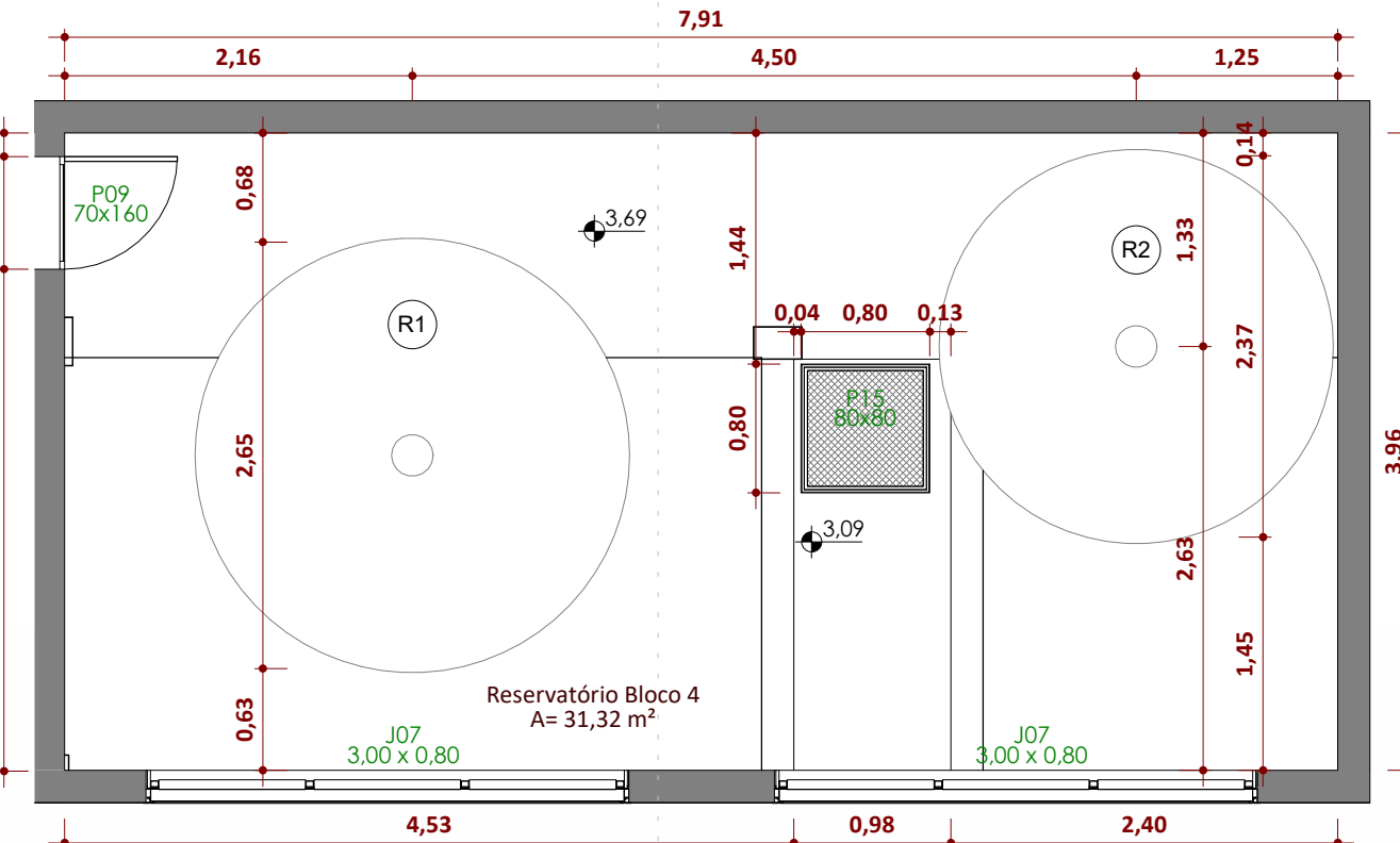
Ampliação Reservatório Bloco 4 ESCALA 1:50
