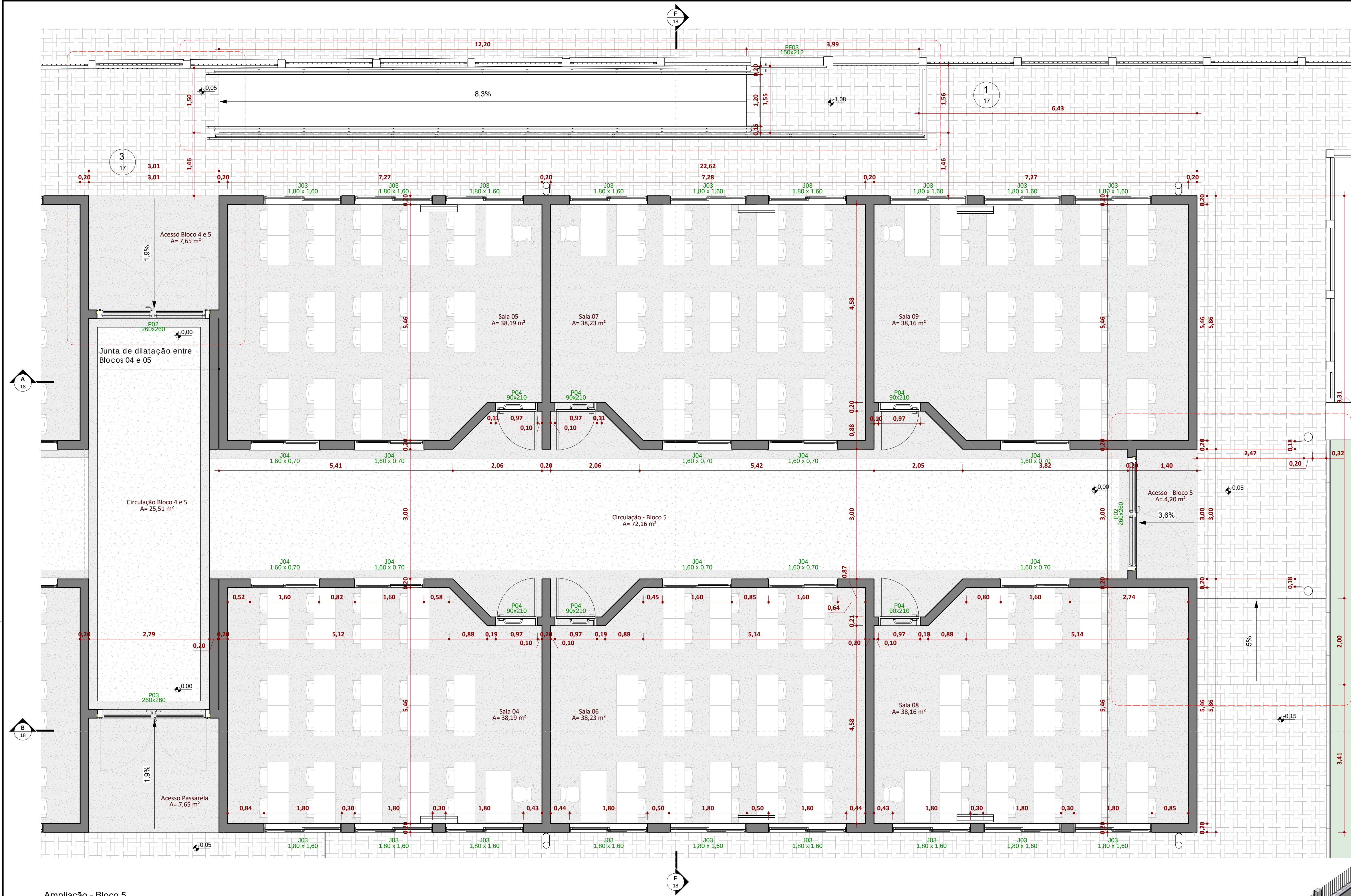
Ampliação - Bloco 5 ESCALA 1:50
