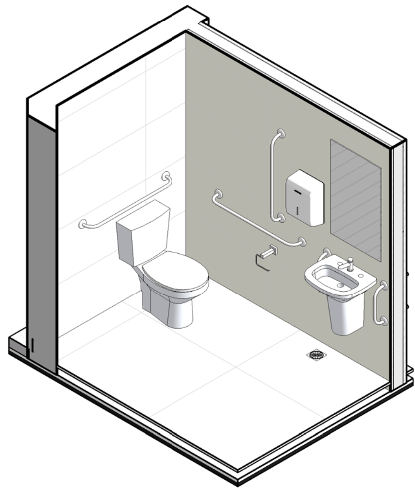
Bloco 2 - Perspectiva Sanitário Masculino Professores PCD ESCALA
