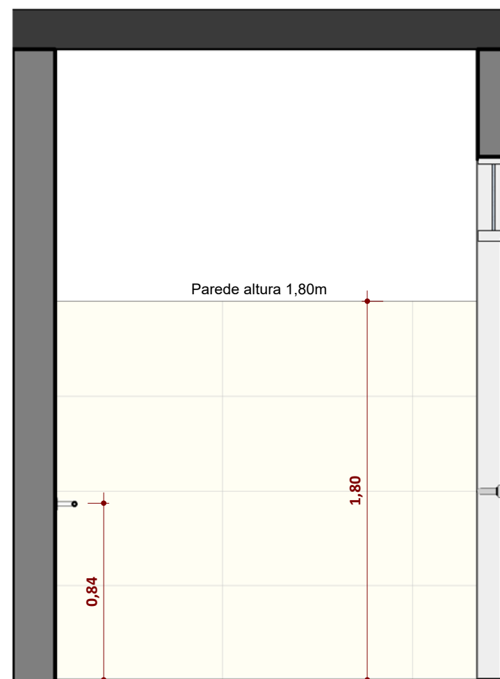
Bloco 2 - Sanitário PCD Masc. - Elevação 9.2 d ESCALA 1:25
