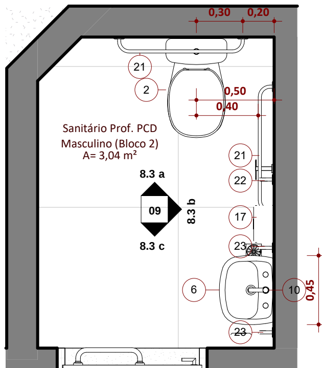
Ampliação - Bloco 2 - 9.3 - Sanitário PCD Masculino Prof. ESCALA 1:25
