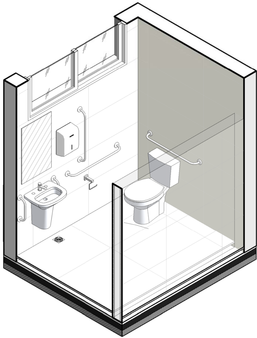
Bloco 2 - Perspectiva Sanitário Masculino PCD ESCALA
