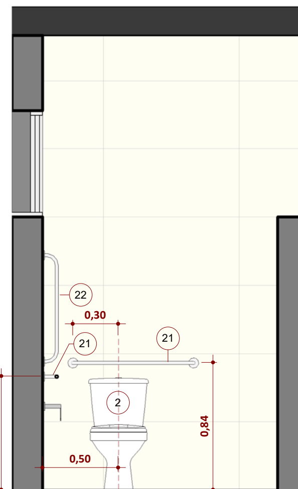
Bloco 2 - Sanitário PCD Masc. - Elevação 9.2 c ESCALA 1:25
