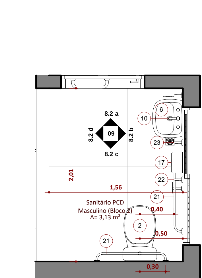
Ampliação - Bloco 2 - 9.2 Sanitário PCD Masculino ESCALA 1:25
