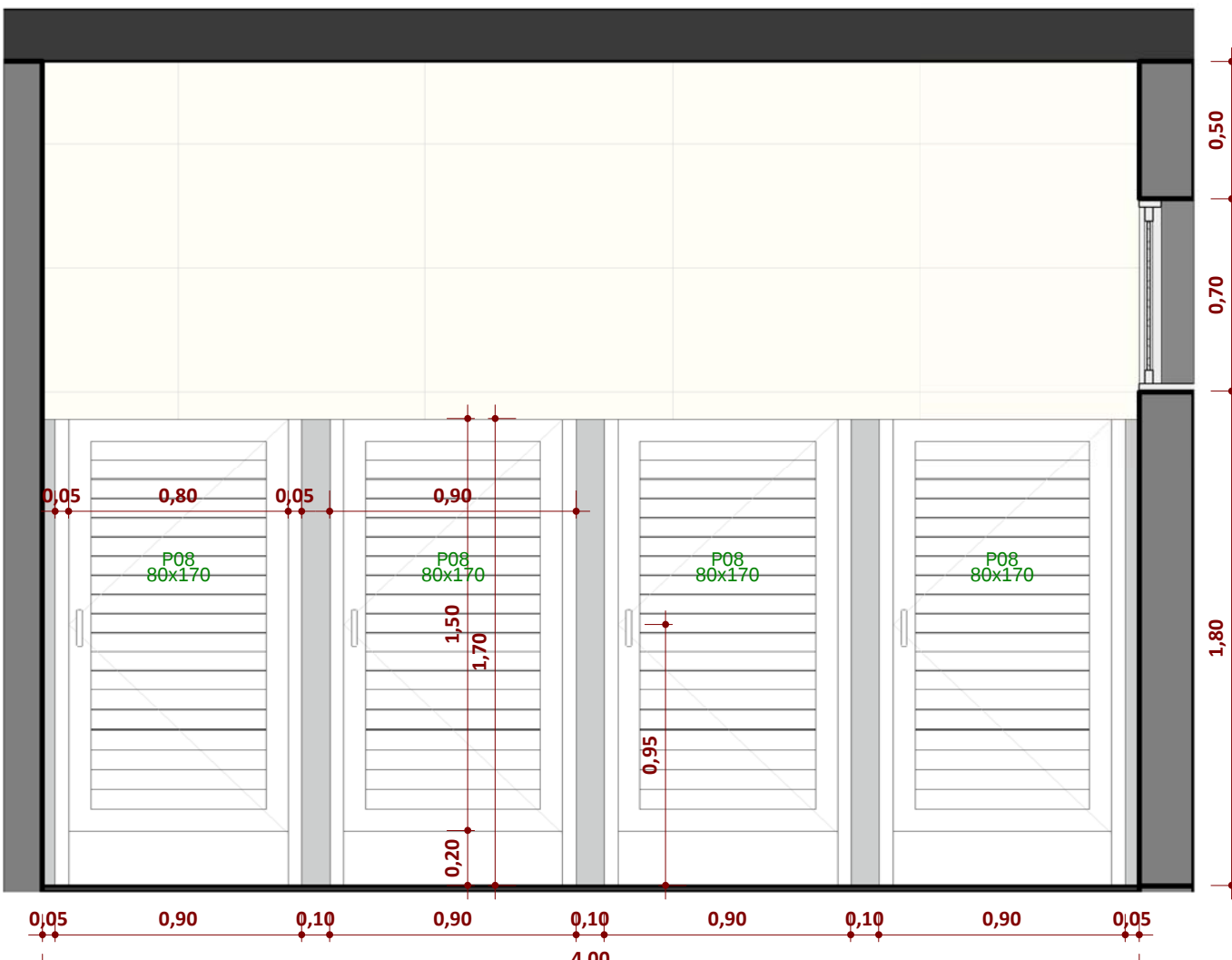
Bloco 2 - Sanitário Masculino - Elevação 9.1 c ESCALA 1:25
