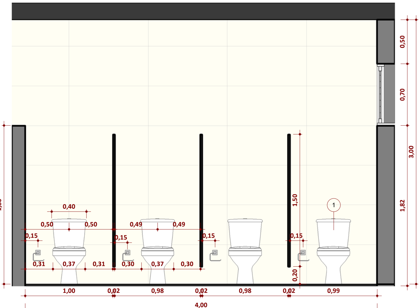
Bloco 2 - Sanitário Masculino - Corte 9.1 C1 ESCALA 1:25
