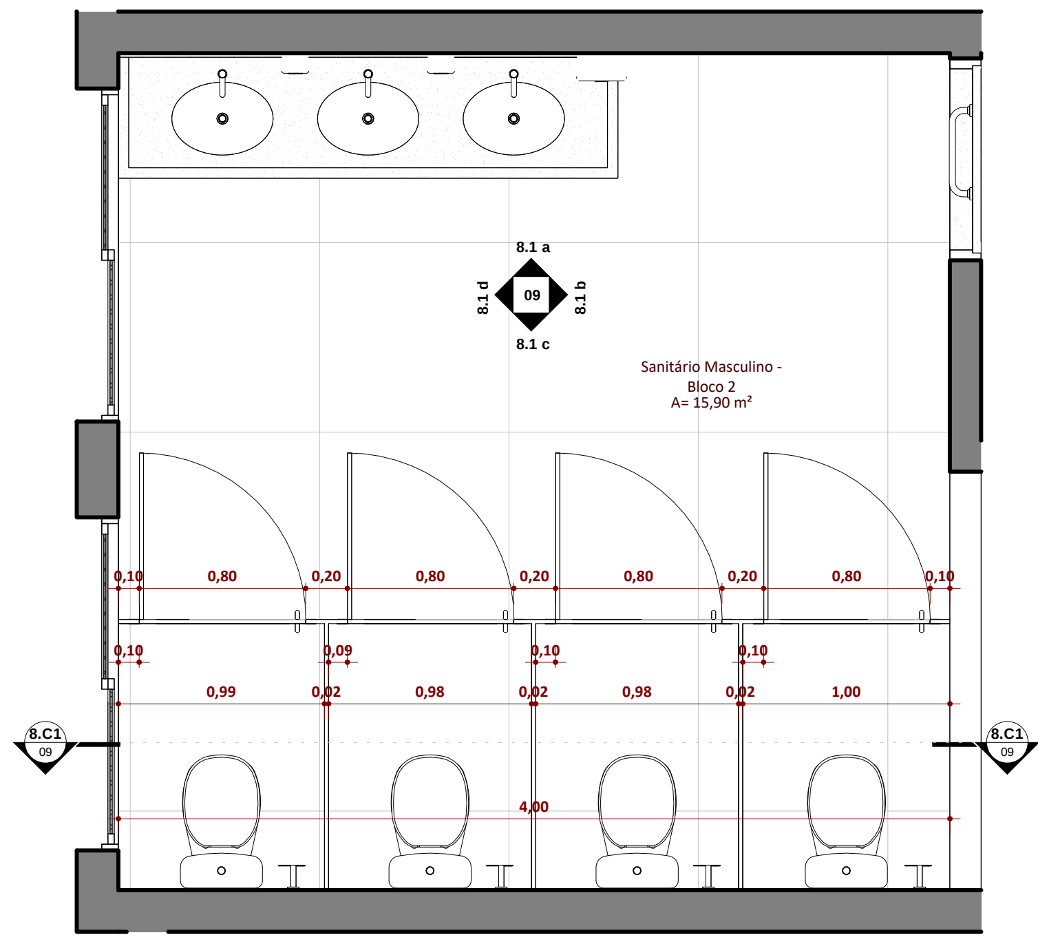
Ampliação - Bloco 2 - 9.1 Sanitário Masculino ESCALA 1:25
