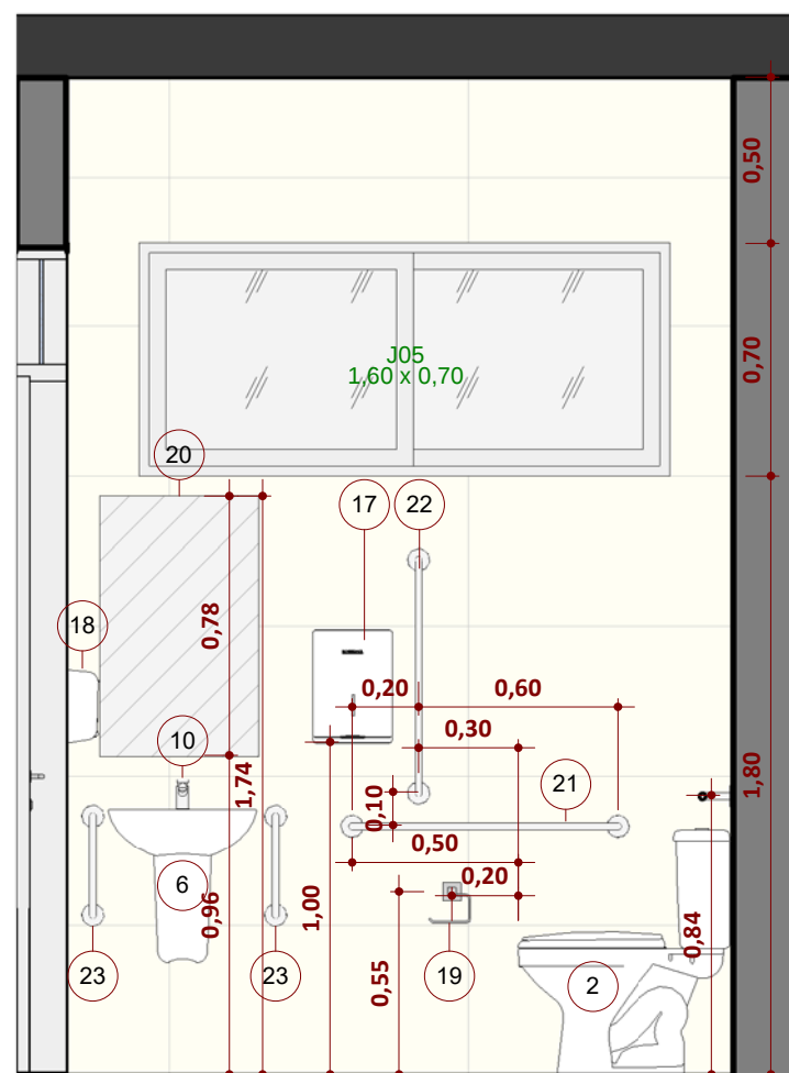
Bloco 2 - Sanitário PCD Masc. - Elevação 9.2 b ESCALA 1:25
