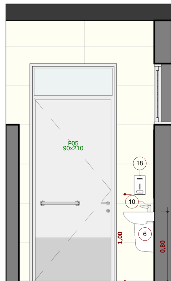
Bloco 2 - Sanitário PCD Masc. - Elevação 9.2 a ESCALA 1:25
