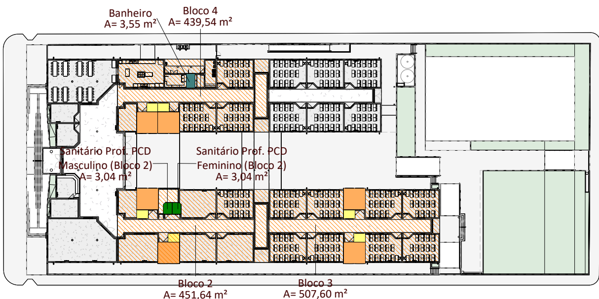
Bloco 2, 3 e 4 - Detalhe Sanitários ESCALA 1:750
