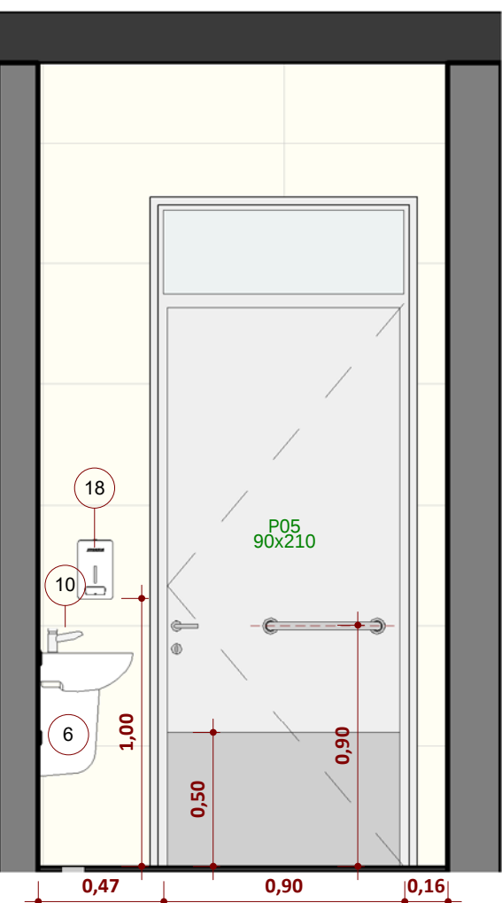
Bloco 2 - Sanitário PCD Masc. Prof. - Elevação 9.3 c ESCALA 1:25
