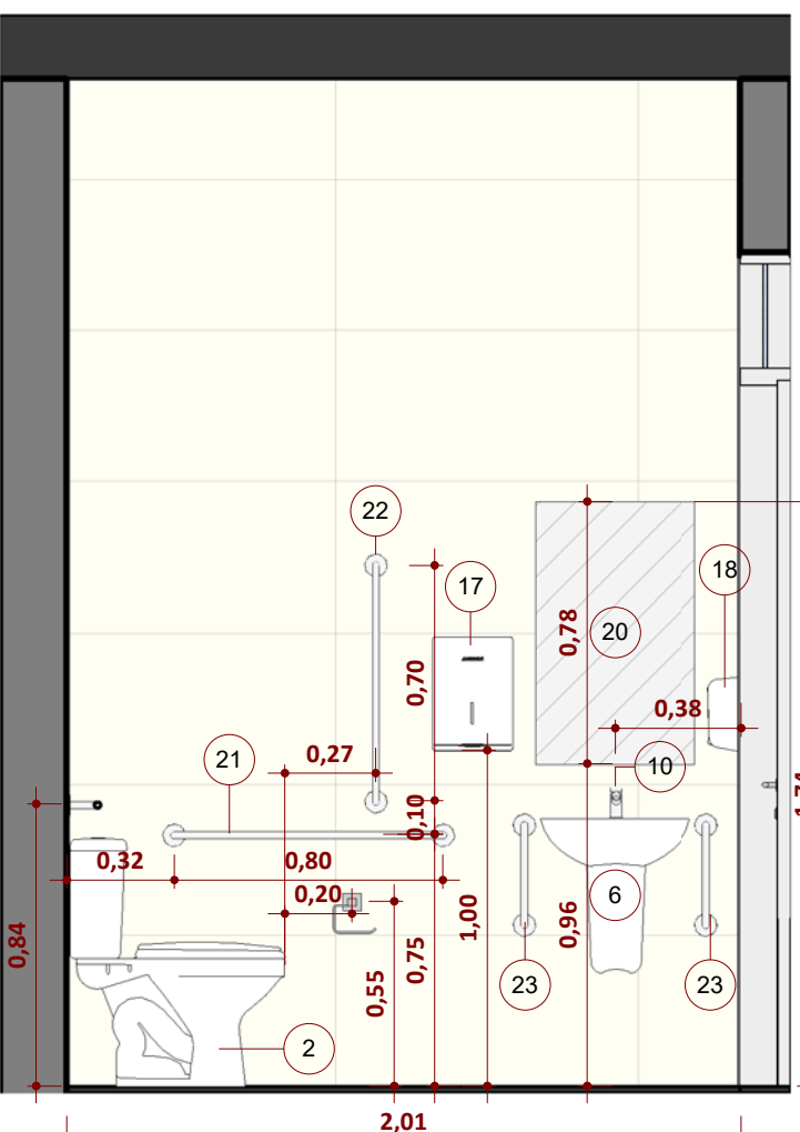
Bloco 2 - Sanitário PCD Masc. Prof. - Elevação 9.3 b ESCALA 1:25
