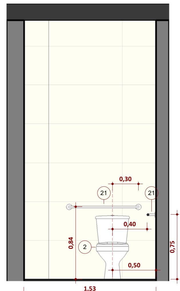
Bloco 2 - Sanitário PCD Masc. Prof. - Elevação 9.3 a ESCALA 1:25
