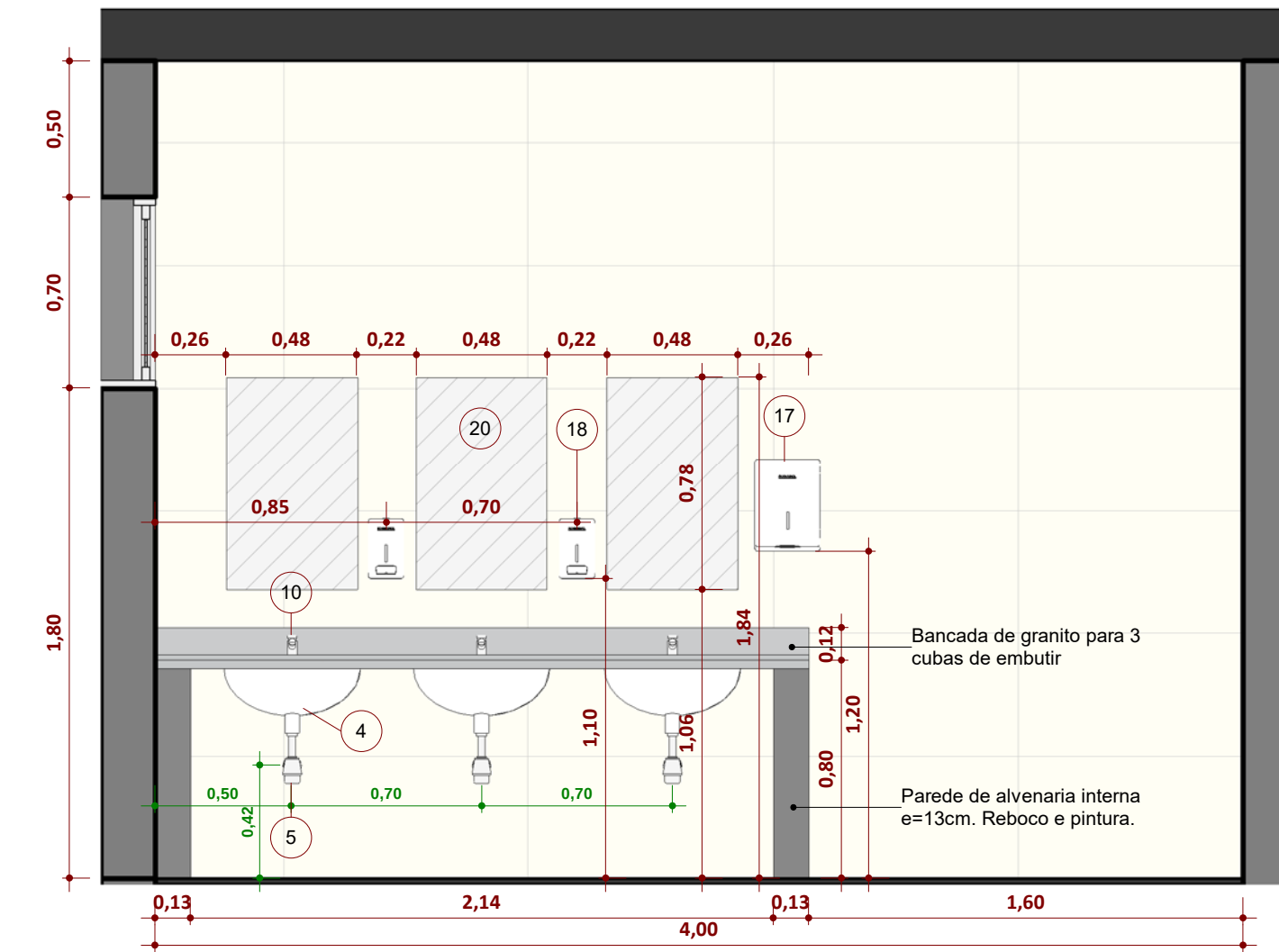
Bloco 2 - Sanitário Masculino - Elevação 9.1 a ESCALA 1:25
