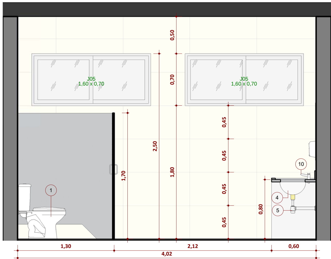
Bloco 2 - Sanitário Masculino - Elevação 9.1 d ESCALA 1:25
