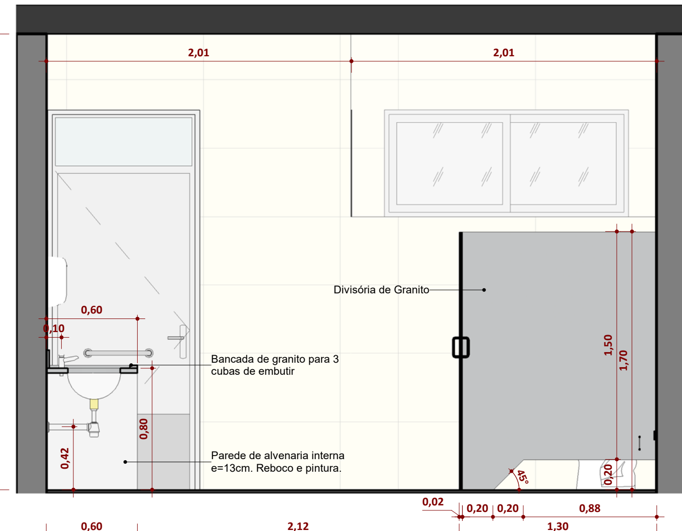
Bloco 2 - Sanitário Masculino - Elevação 9.1 b ESCALA 1:25
