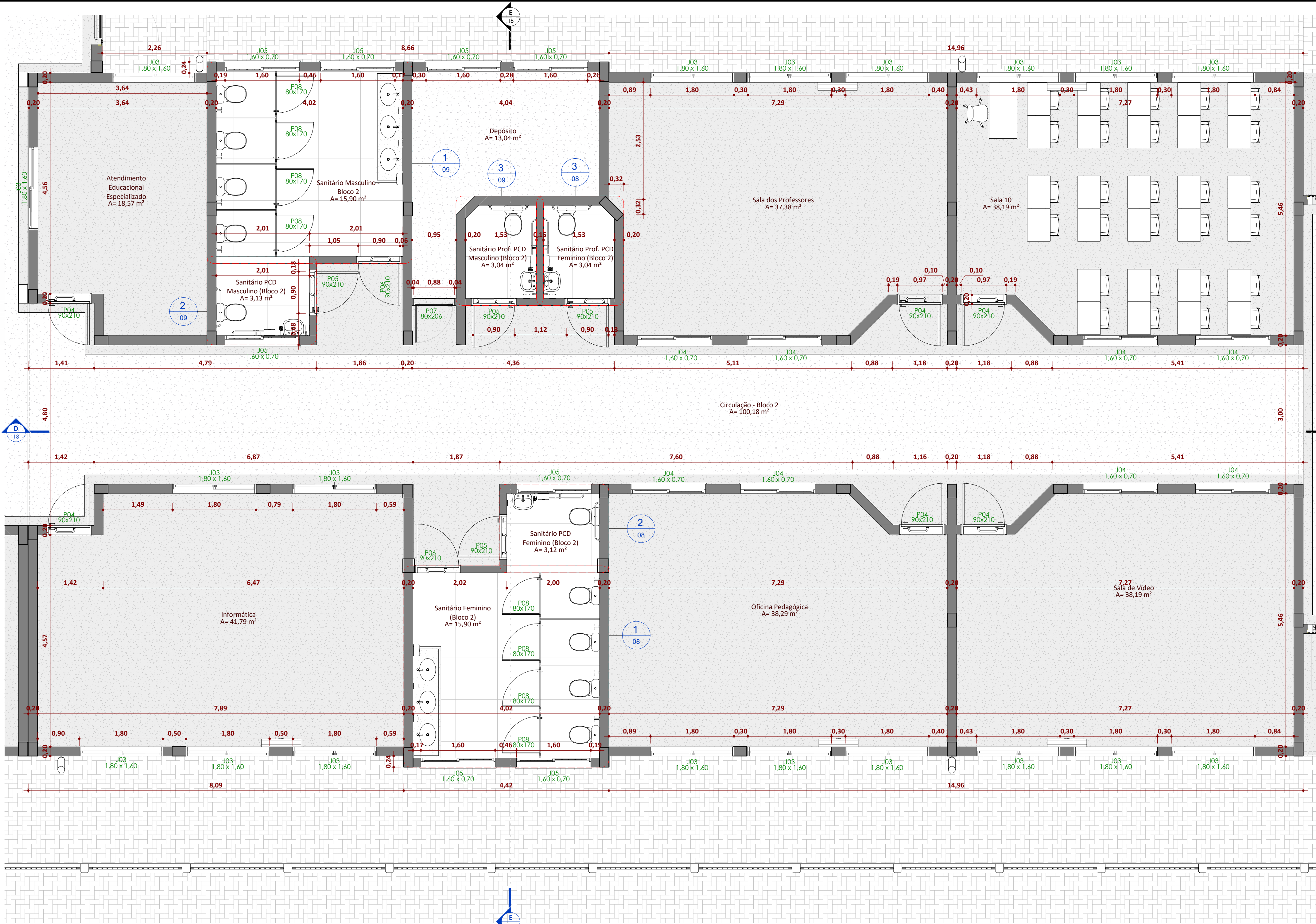
Ampliação - Bloco 2 ESCALA 1 : 50
