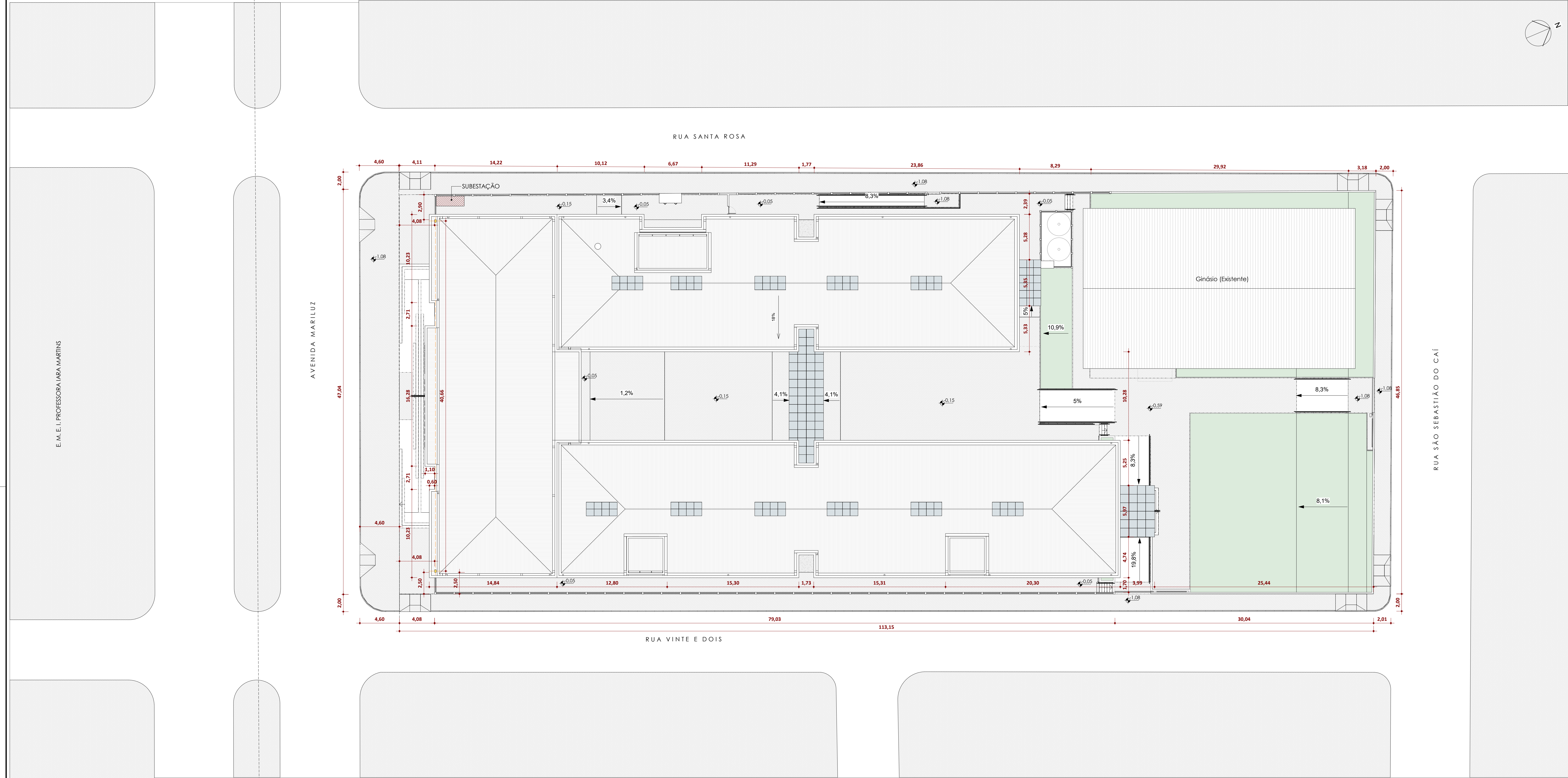
Planta de Implantação ESCALA 1:200
