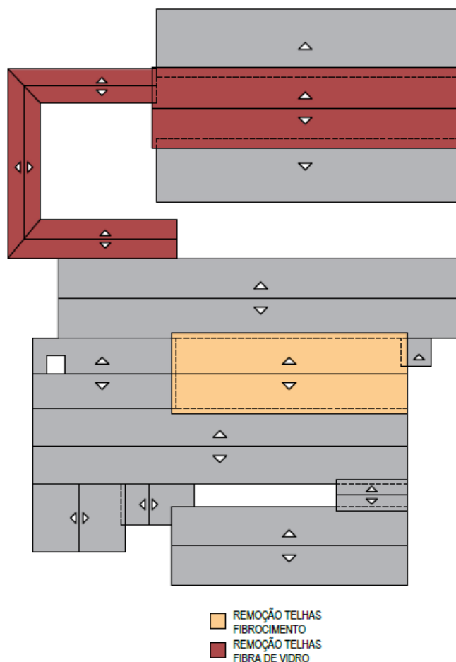
Croqui demolições da cobertura
