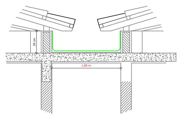
POSIÇÃO DA CALHA ENTRE DOIS TELHADOS
