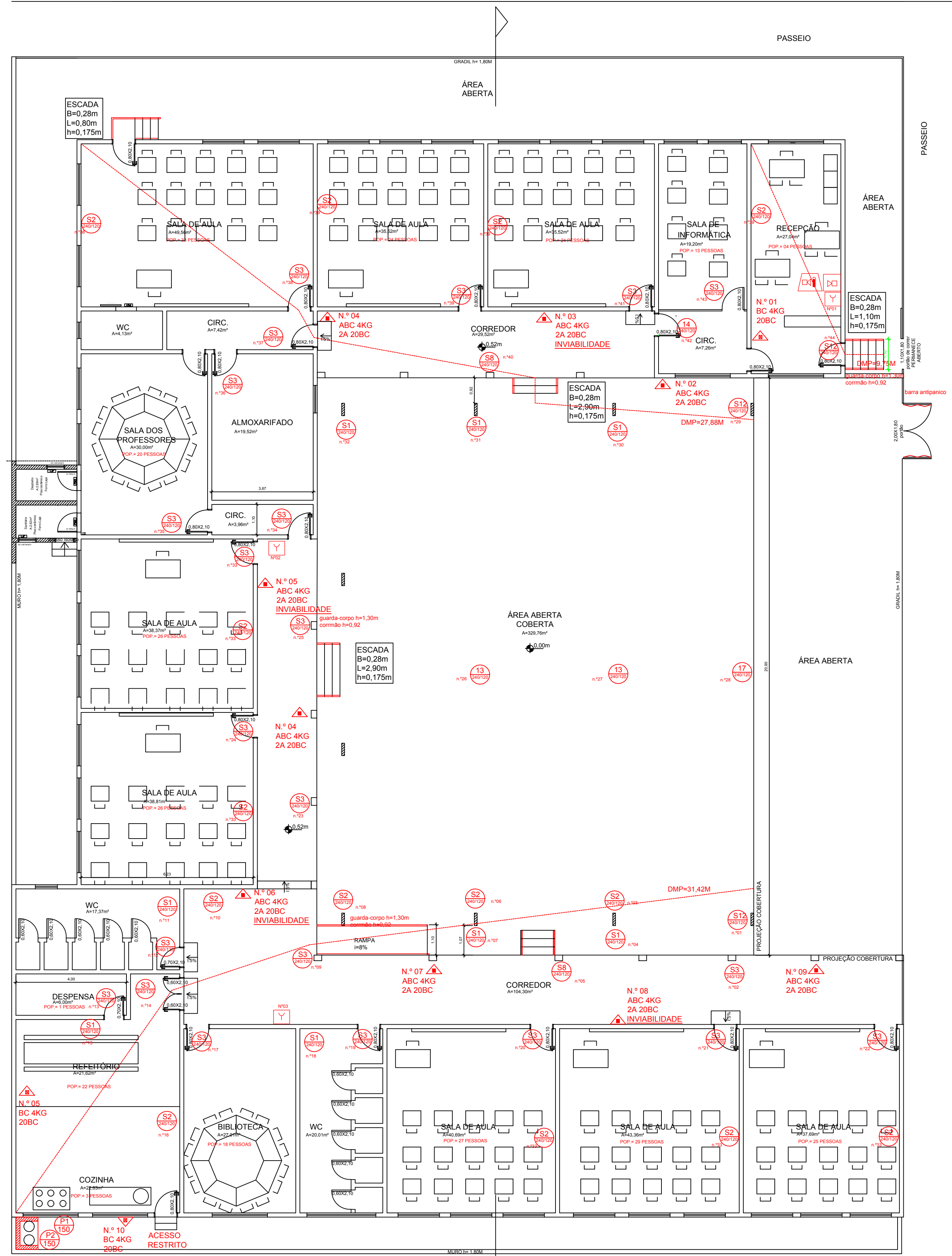
PLANTA BAIXA A=1.063,00M² ESC: 1/100
