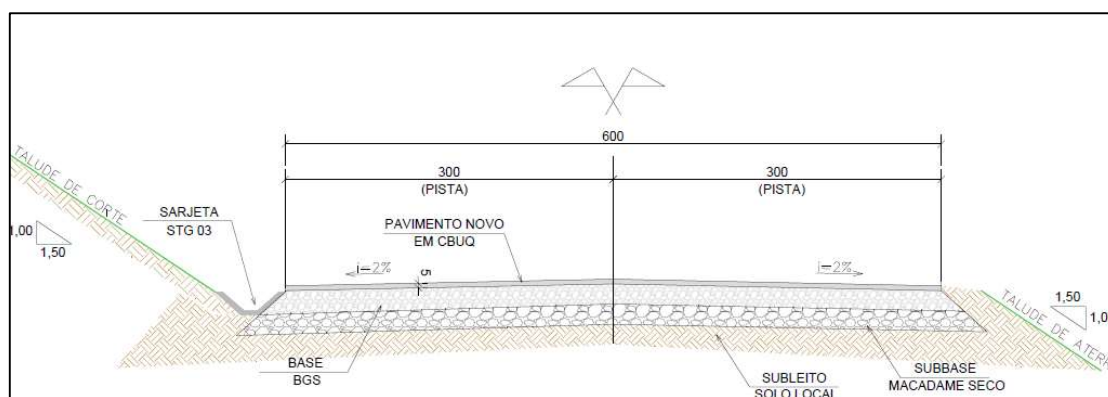
Figura 1 – Seção tipo com plataforma de rolamento de 6,00 metros.
