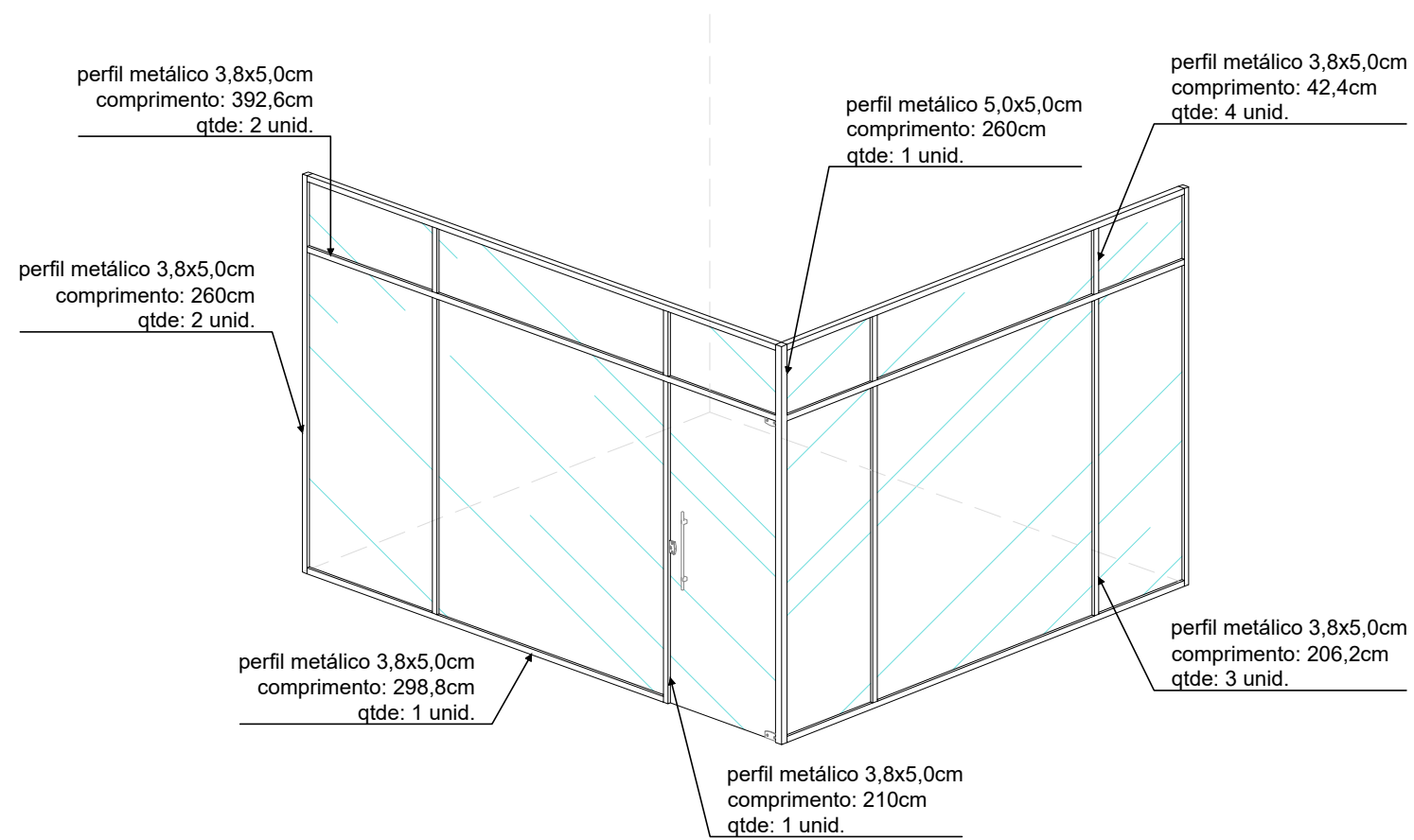
PERSPECTIVA ISOMÉTRICA
