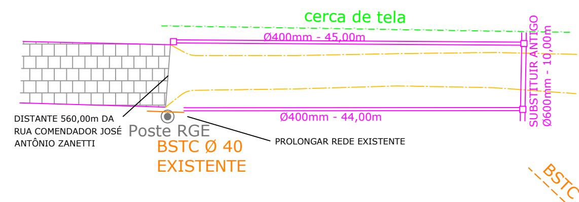
QUANTITATIVOS DRENAGEM RUA EXP. JOÃO BATISTA ALBERTON
