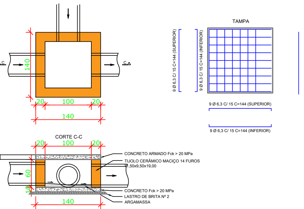
CAIXA DE LIGAÇÃO E PASSAGEM (CLP)
