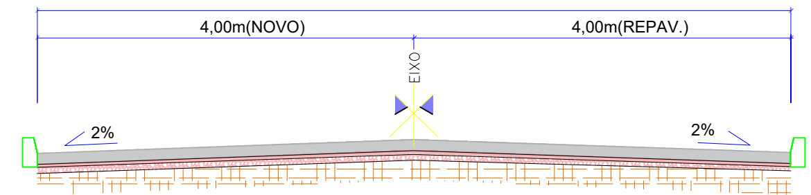
SEÇÃO TIPO PAVIMENTAÇÃO - 8,00M
