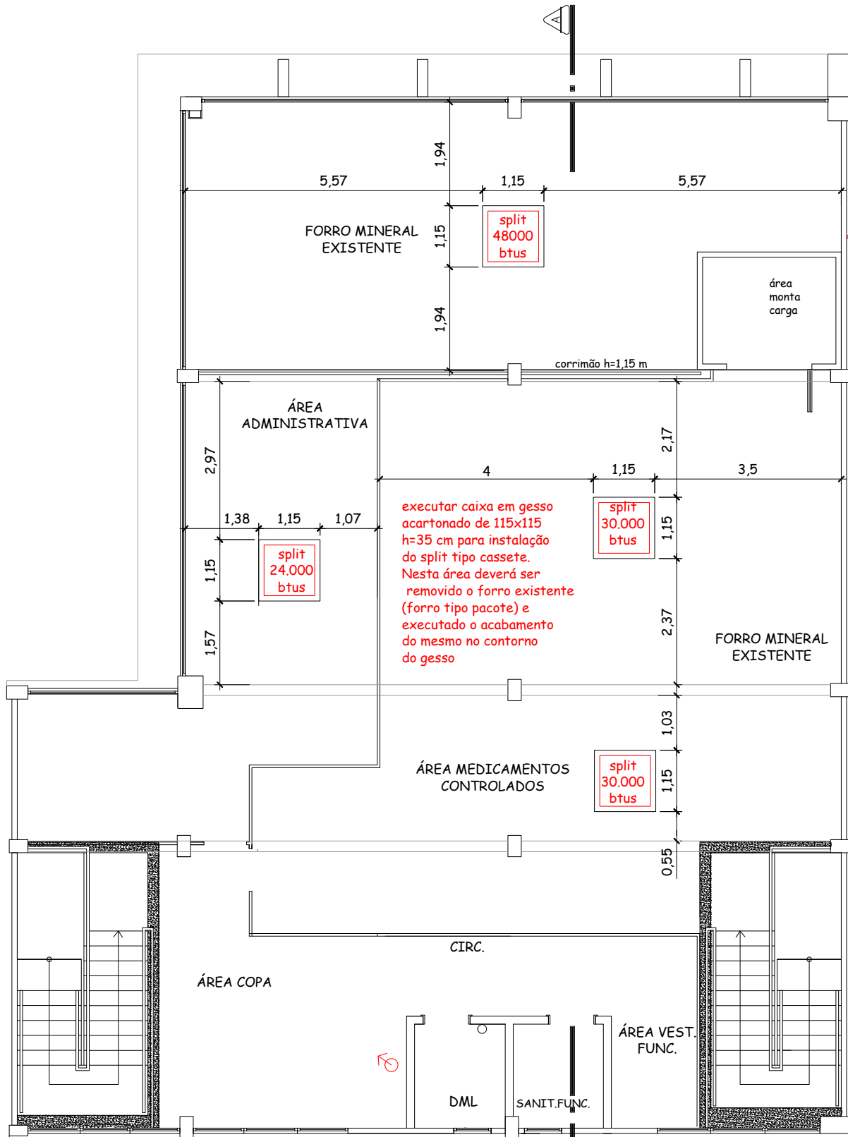
PLANTA BAIXA FORRO MEZANINO - ÁREA CAIXAS EM GESSO ACARTONADO PARA SPLITS esc:1/100
