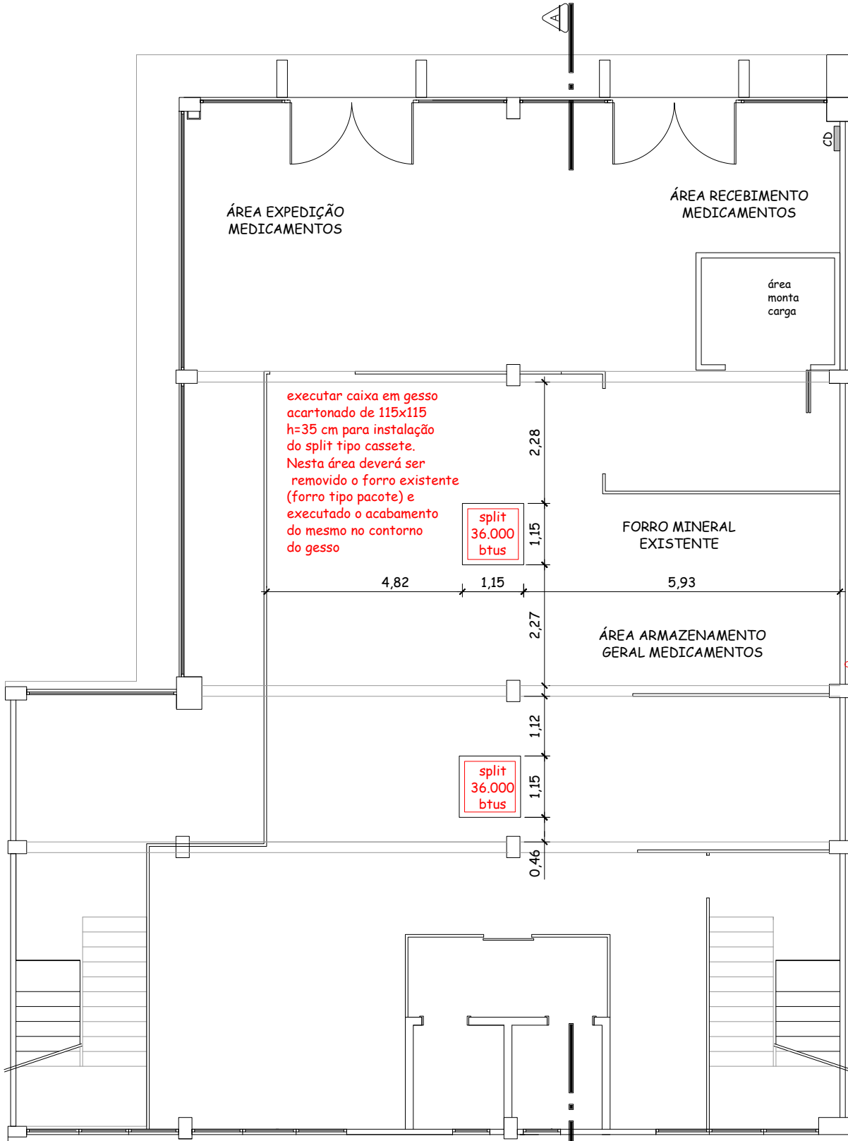
PLANTA BAIXA FORRO TÉRREO - ÁREA CAIXAS EM GESSO ACARTONADO PARA SPLITS esc:1/100
