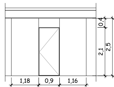
VISTA 08 esc:1/100
