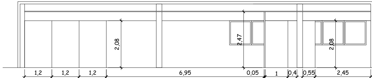
CORTE AA'
