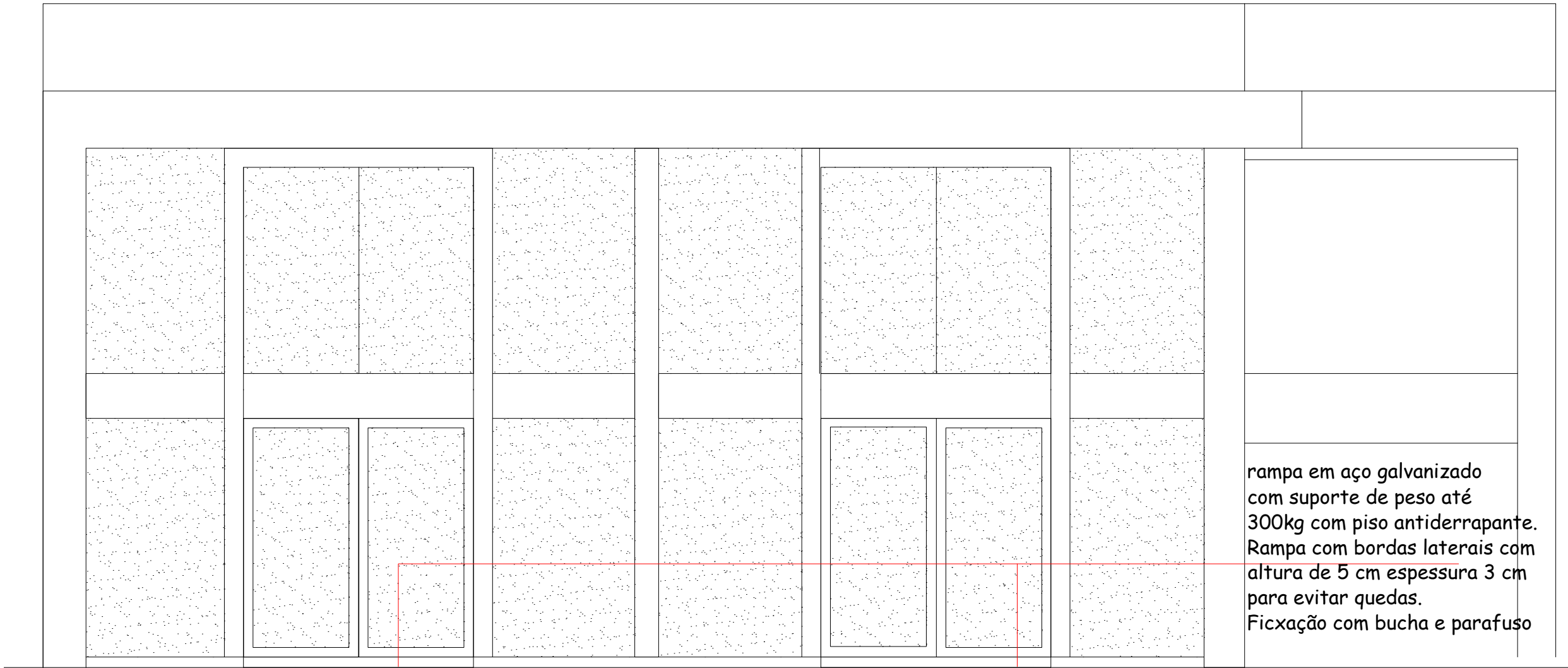
VISTA 01- rampa acesso esc:1/50
