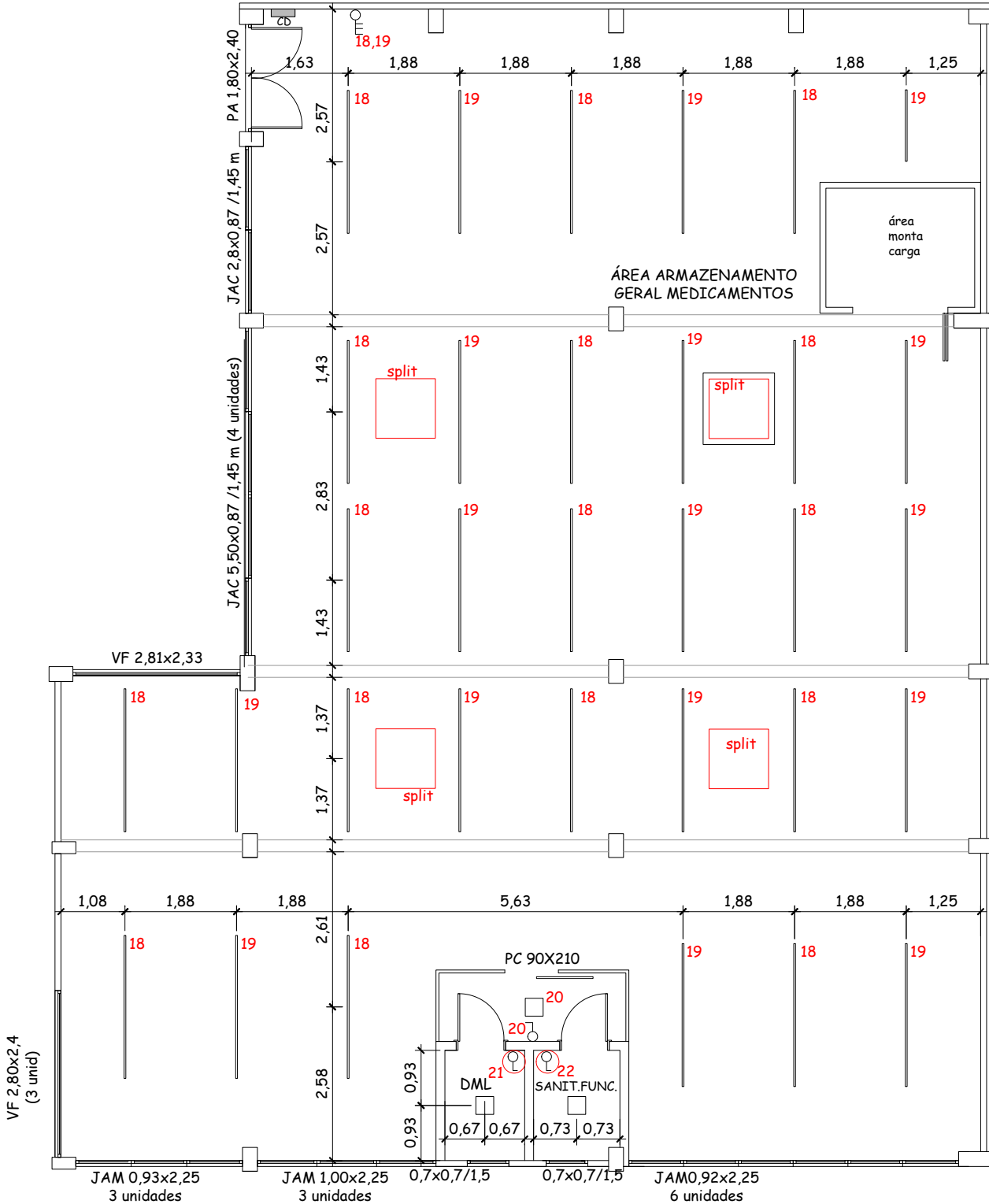
PLANTA SUBSOLO - PONTOS ILUMINAÇÃO esc:1/100
