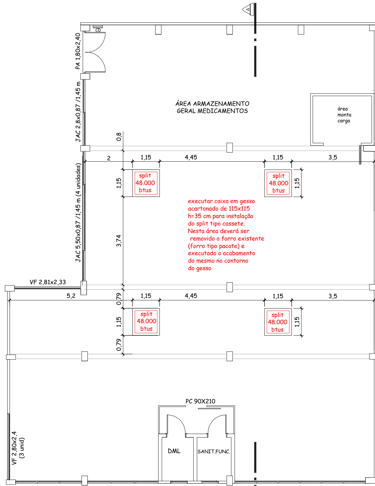
PLANTA BAIXA FORRO SUBSOLO - ÁREA CAIXAS EM GESSO ACARTONADO PARA SPLITS esc:1/100
