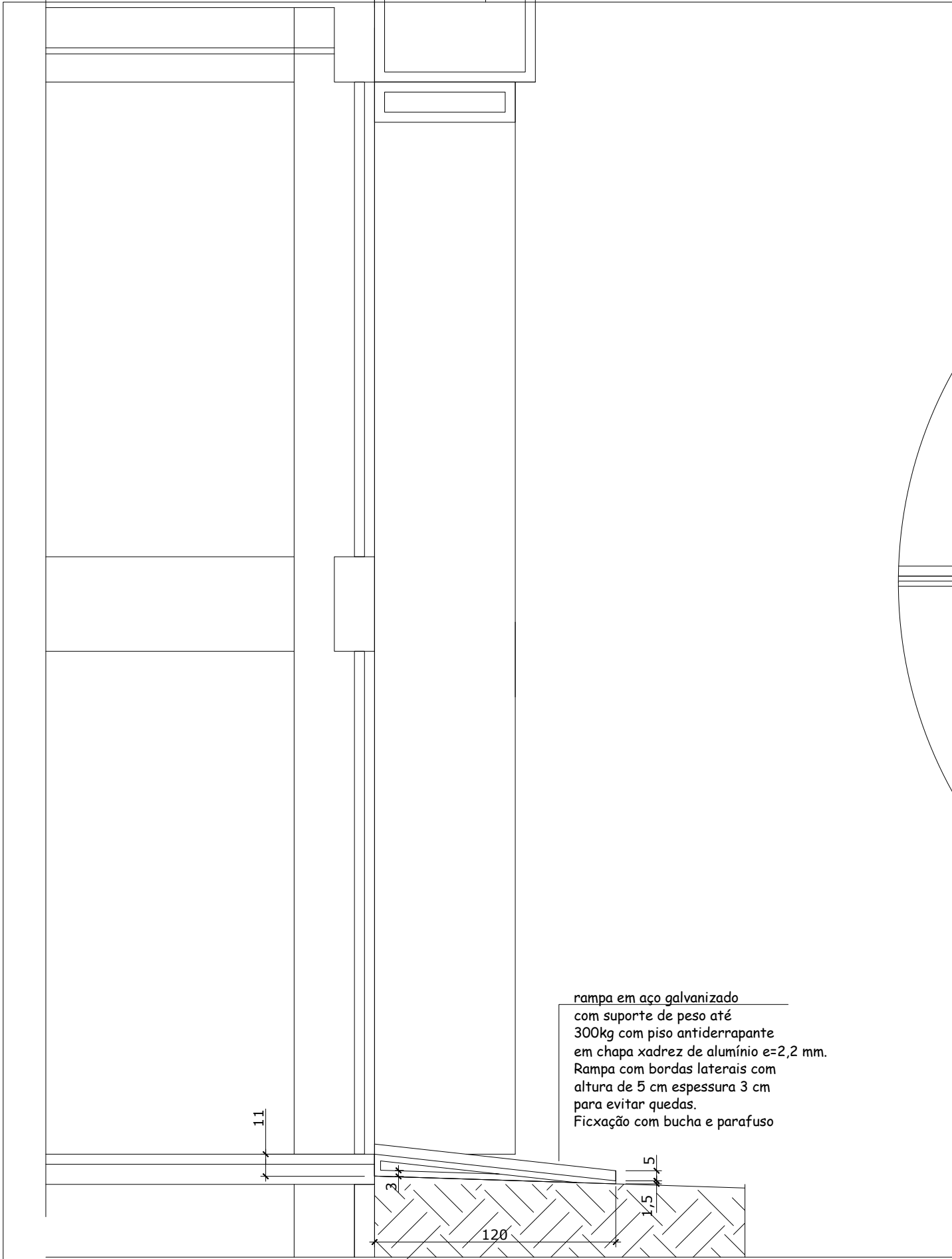
DET. RAMPA ACESSO - corte esquemático ESCALA 1/25
