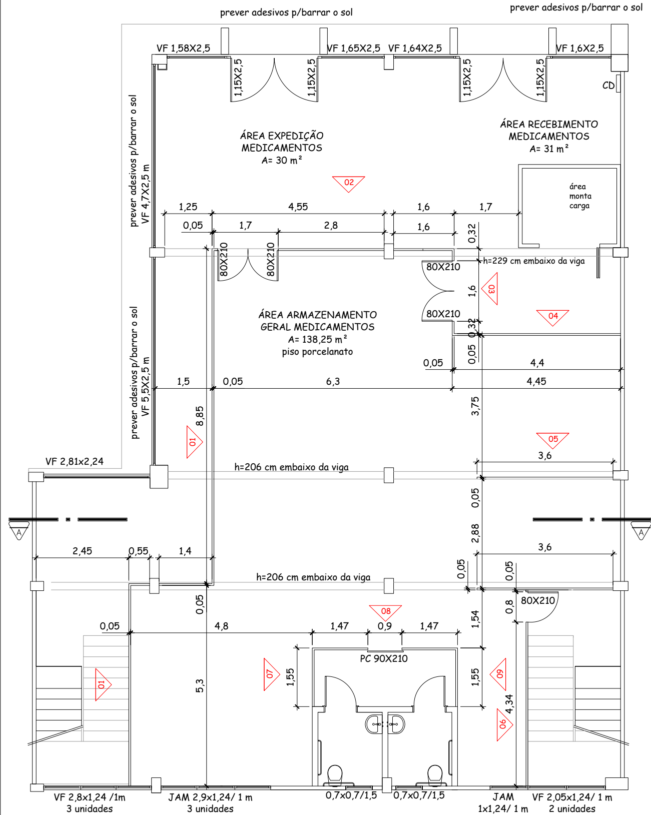
PLANTA BAIXA TÉRREO - divisórias PVC esc:1/100
