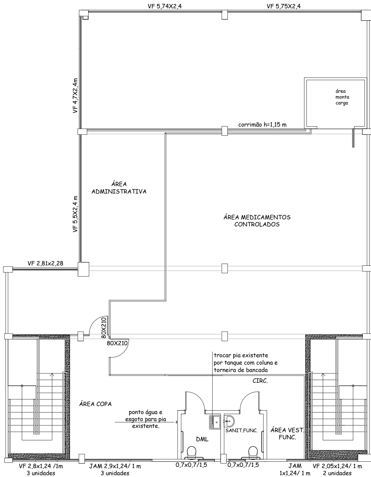
PLANTA PONTOS HIDRÁULICOS - MEZANINO esc:1/100
