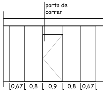
VISTA 08
