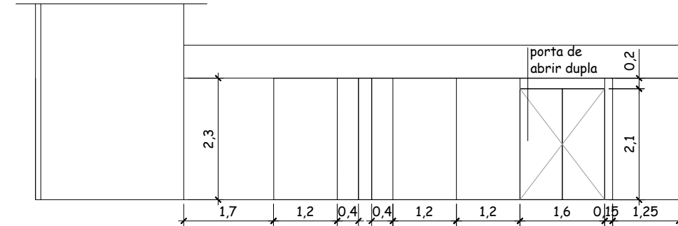
VISTA 02
