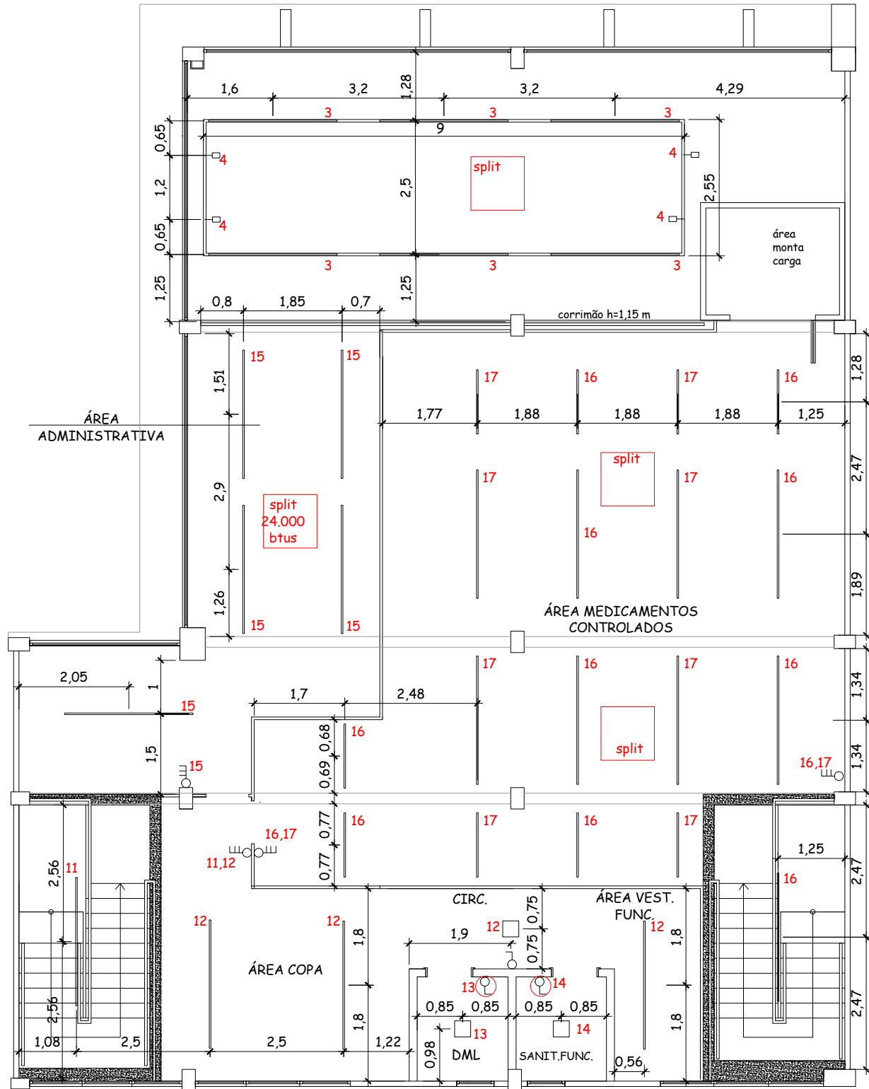
PLANTA BAIXA MEZANINO -PONTOS ILUMINAÇÃO esc:1/100
