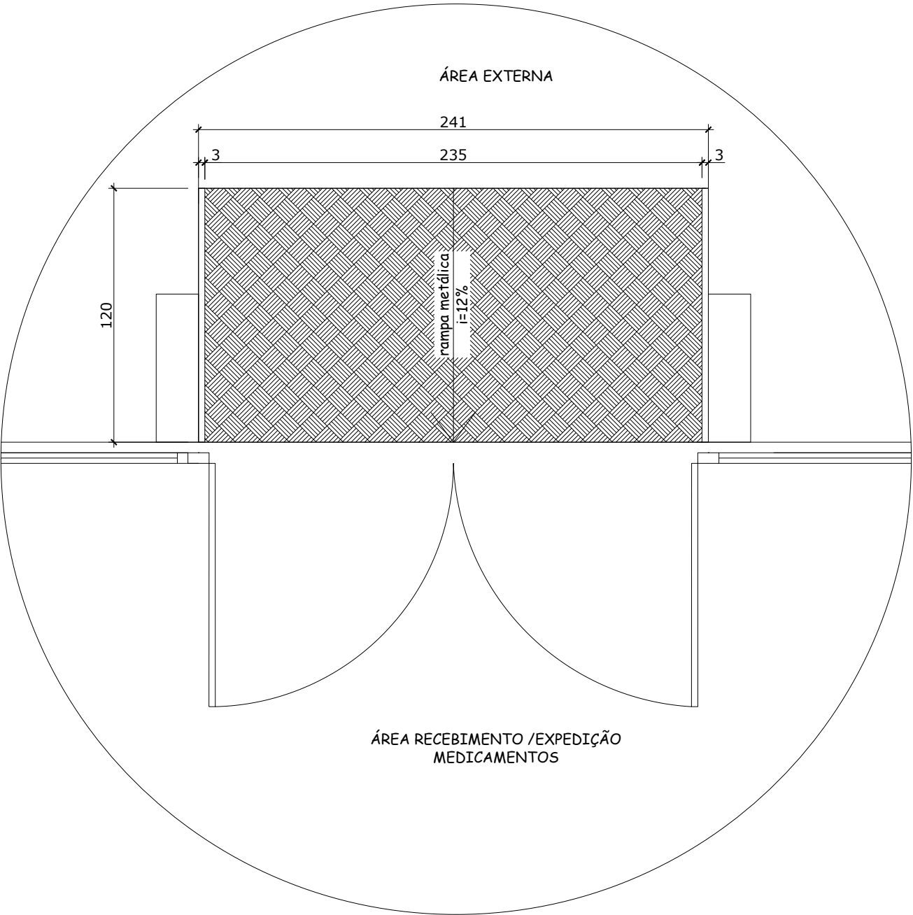
DET. RAMPA ACESSO - planta baixa ESCALA 1/25
