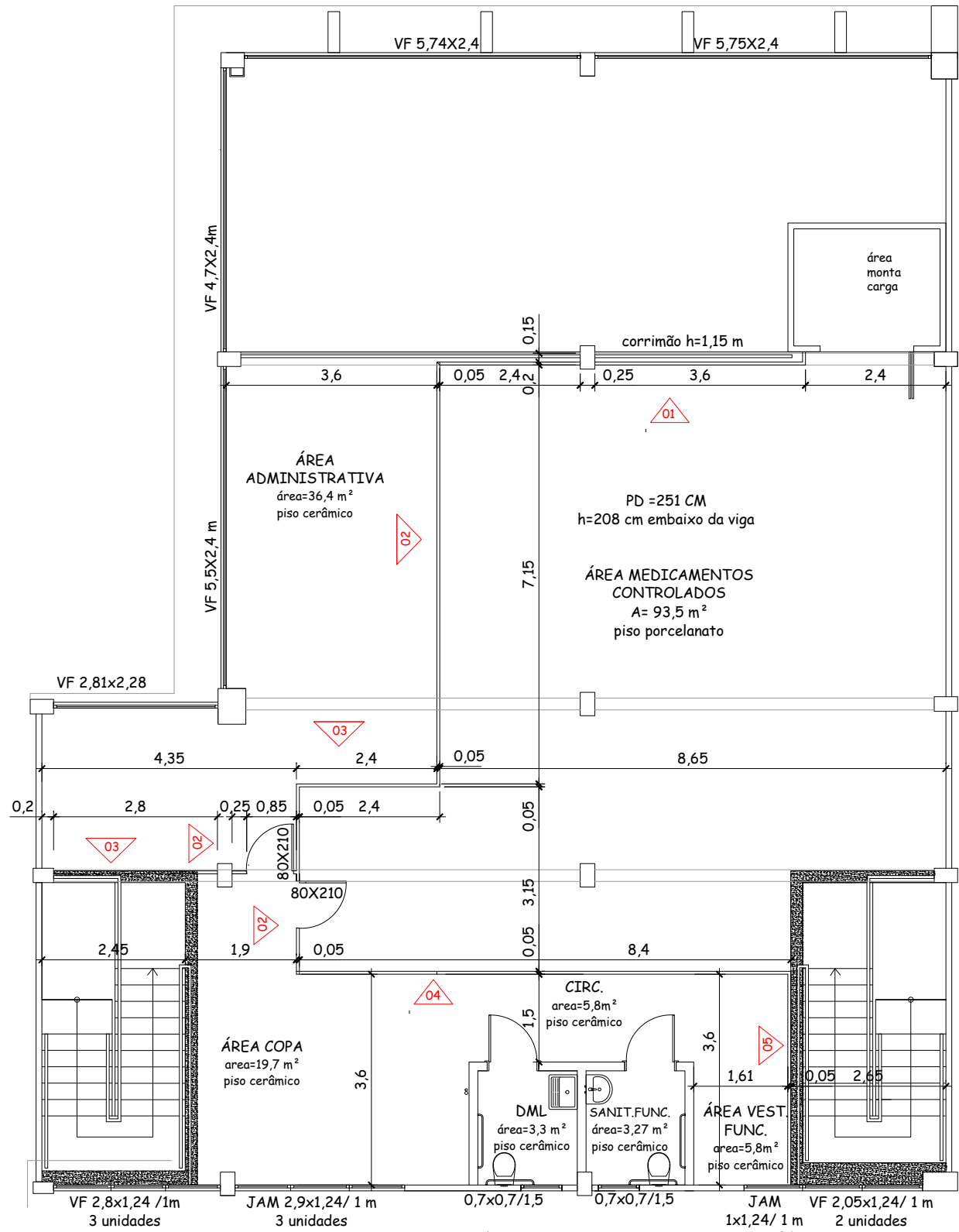
PLANTA BAIXA - MEZANINO esc:1/100
