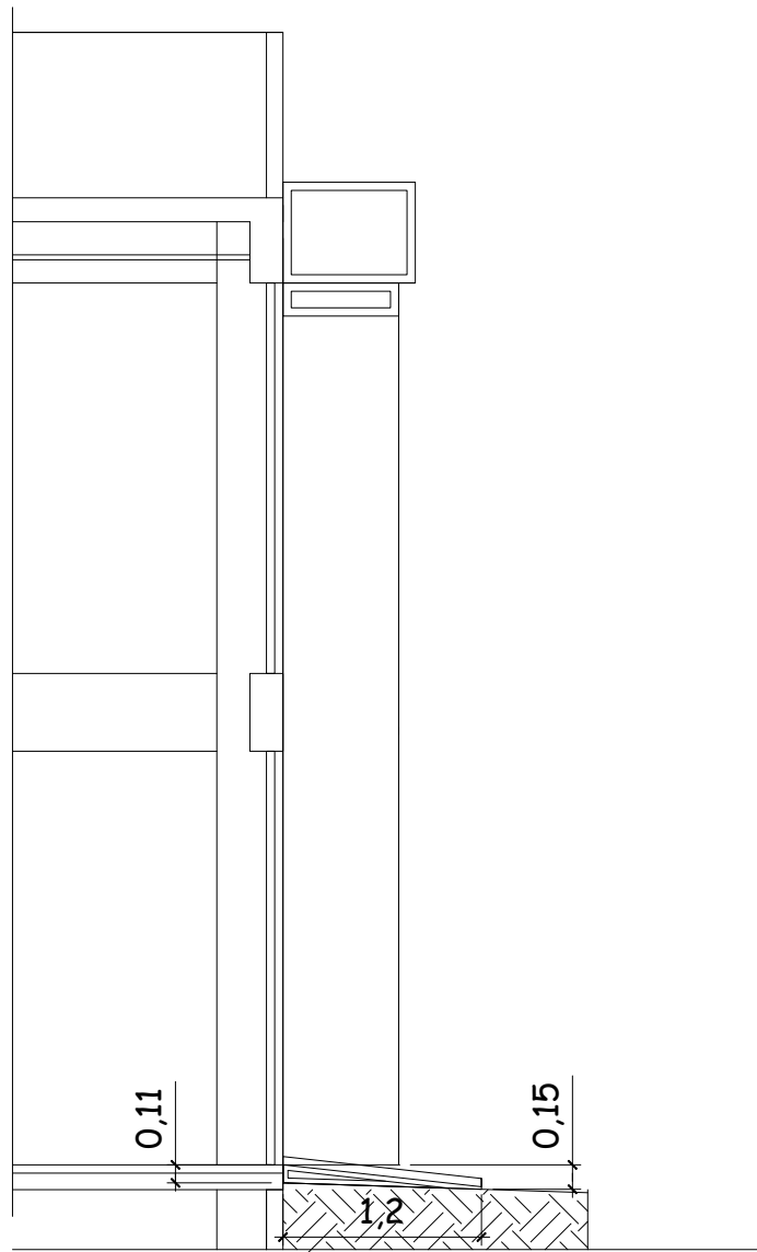
CORTE BB' - rampa acesso esc:1/50
