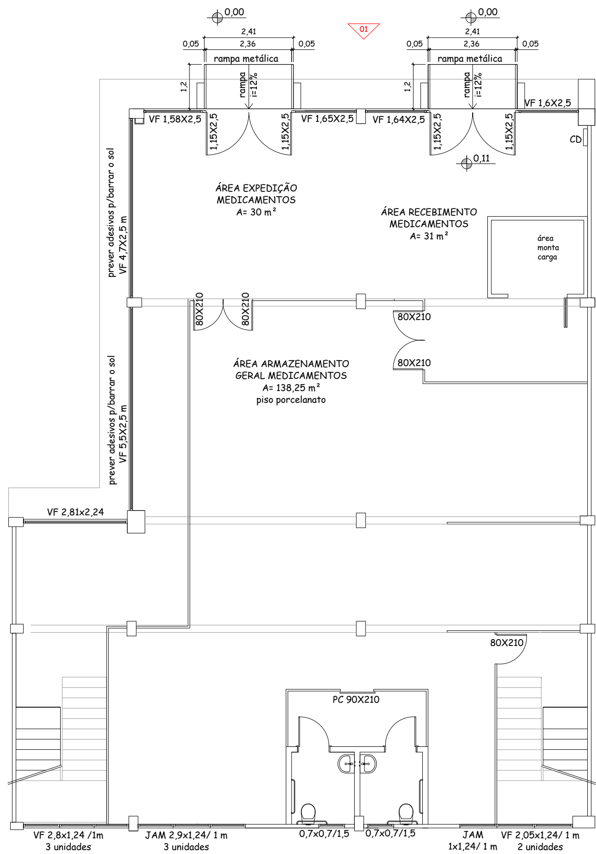
PLANTA BAIXA TÉRREO - det.rampa acesso esc:1/100
