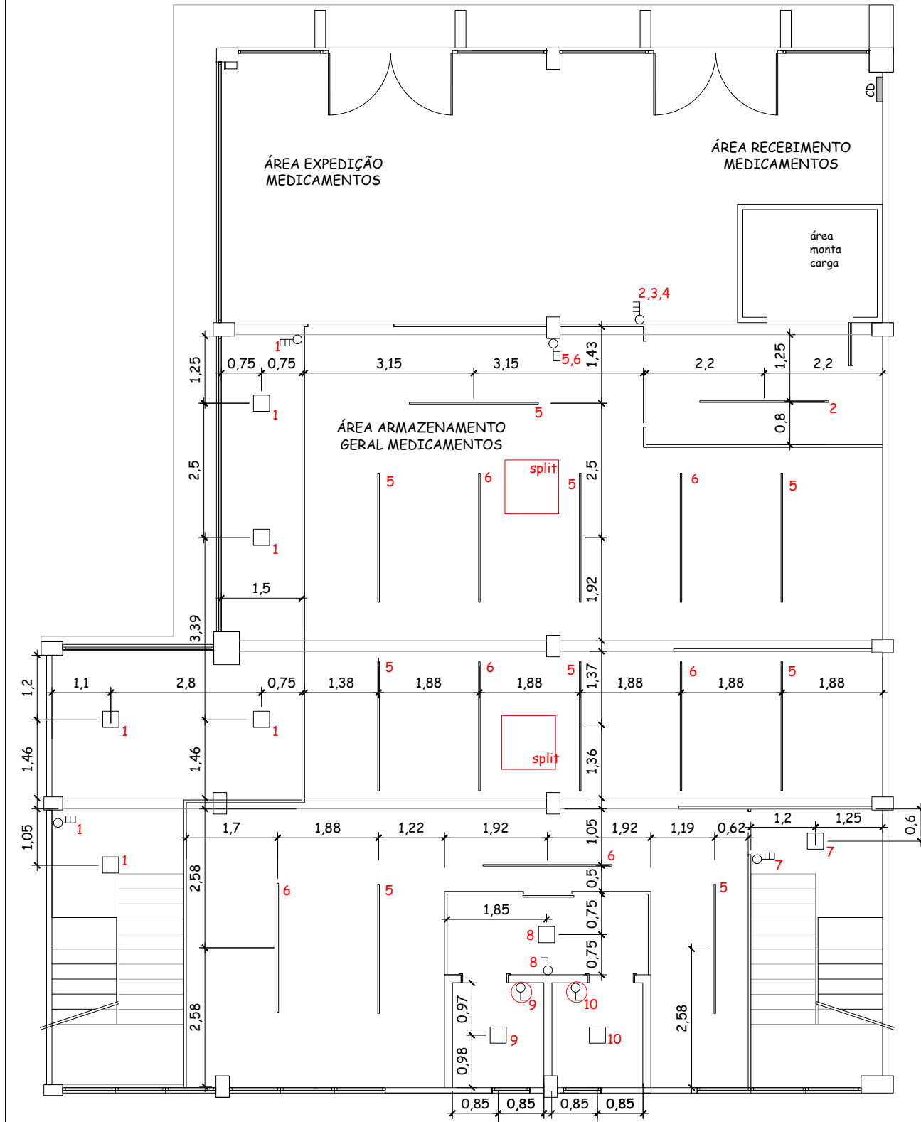
PLANTA BAIXA TÉRREO - PONTOS ILUMINAÇÃO esc:1/100
