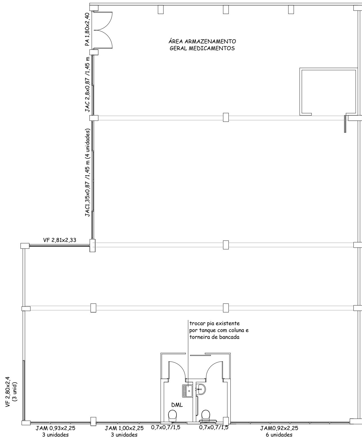
PLANTA PONTOS HIDRÁULICOS -SUBSOLO esc:1/100
