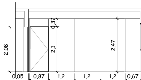
VISTA 06
