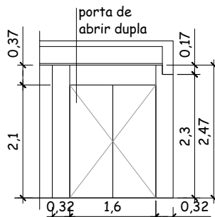
VISTA 03
