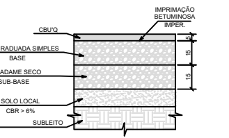
DETALHE 1 - PAVIMENTO ASFÁLTICO
