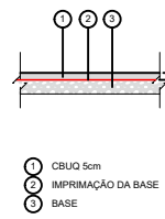
DETALHE - PISTA
