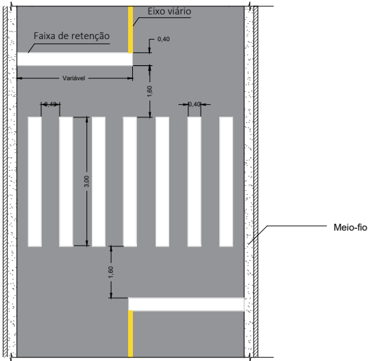
DETALHAMENTO 1 FAIXA DE PEDESTRE
