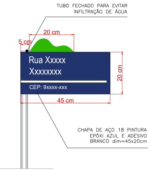
DETALHE PLACAS DE IDENTIFICAÇÃO DAS RUAS
