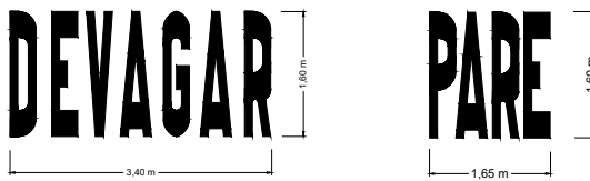
DETALHE DA SINALIZAÇÃO HORIZONTAL EM TEXTO
