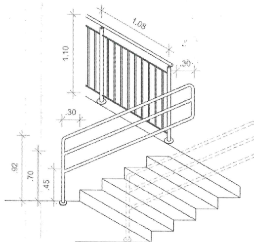
Detalhe da escada, guarda-corpo e corrimãos
