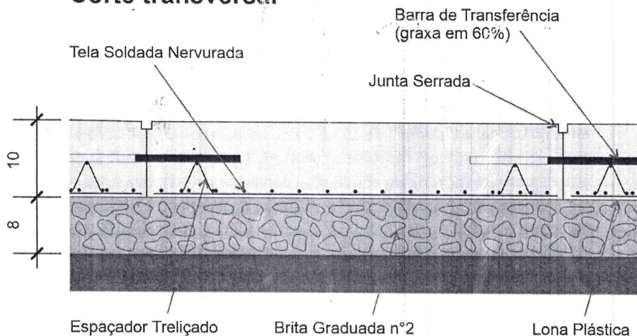
Posicionamento das barras, espaçadores e telas
