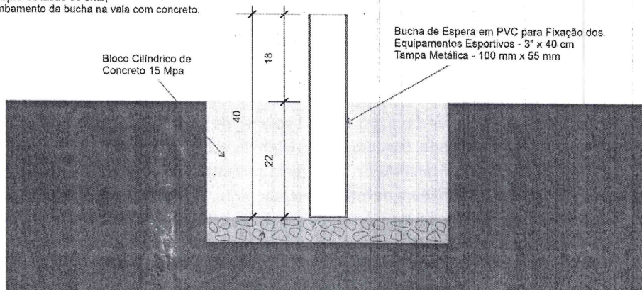
Detalhe da fundação das Buchas dos Equipamentos Esportivos
