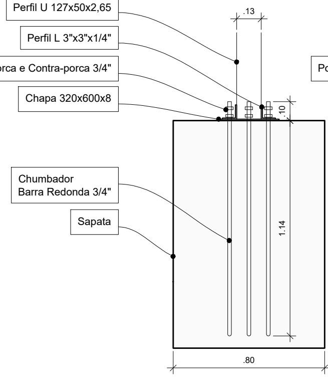
DETALHES DA BASE DOS PILARES DO OITÃO SAPATAS Nº 11 A 14
