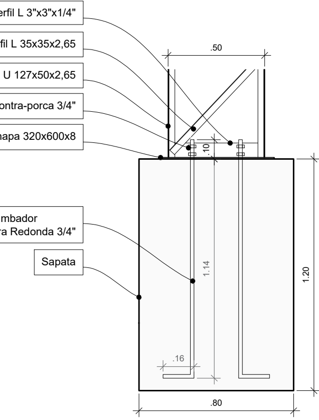
DETALHES DA BASE DOS PILARES DO OITÃO SAPATAS Nº 11 A 14
