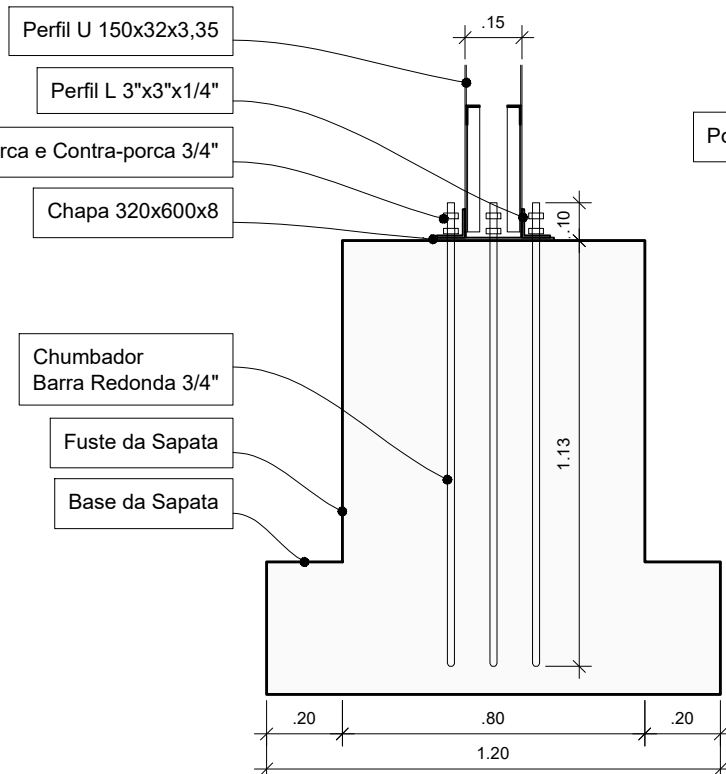
DETALHES DA BASE DOS PILARES PRINCIPAIS SAPATAS Nº 06 A 10
