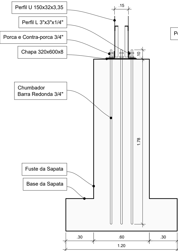
DETALHES DA BASE DOS PILARES PRINCIPAIS SAPATAS Nº 01 A 05
