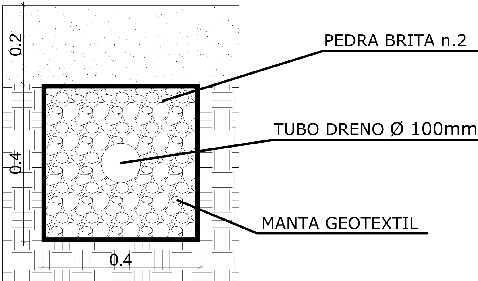
DET. DRENAGEM RAMIFICAÇÃO
