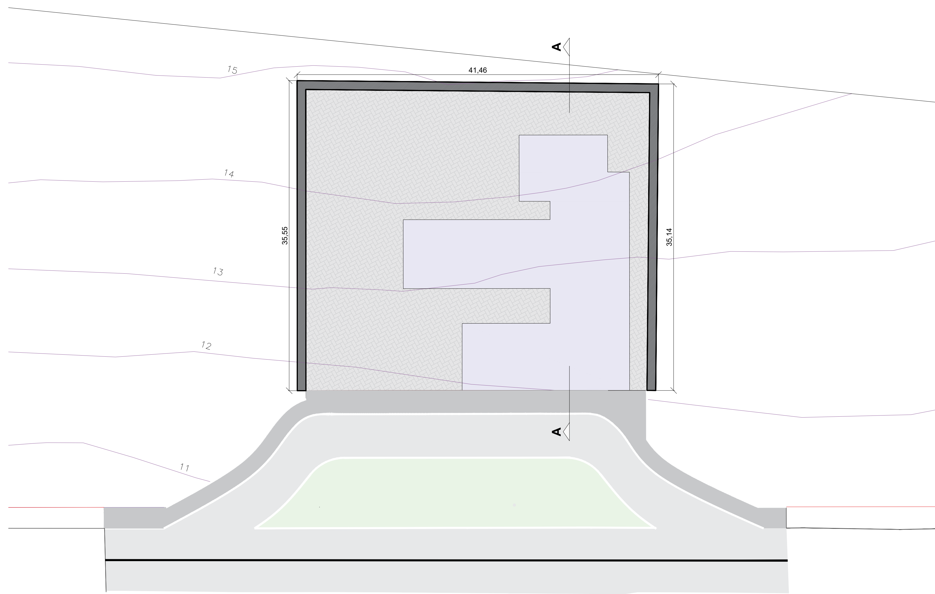
IMPLANTAÇÃO UBS PORTE 1 - BAIRRO MORRETES
