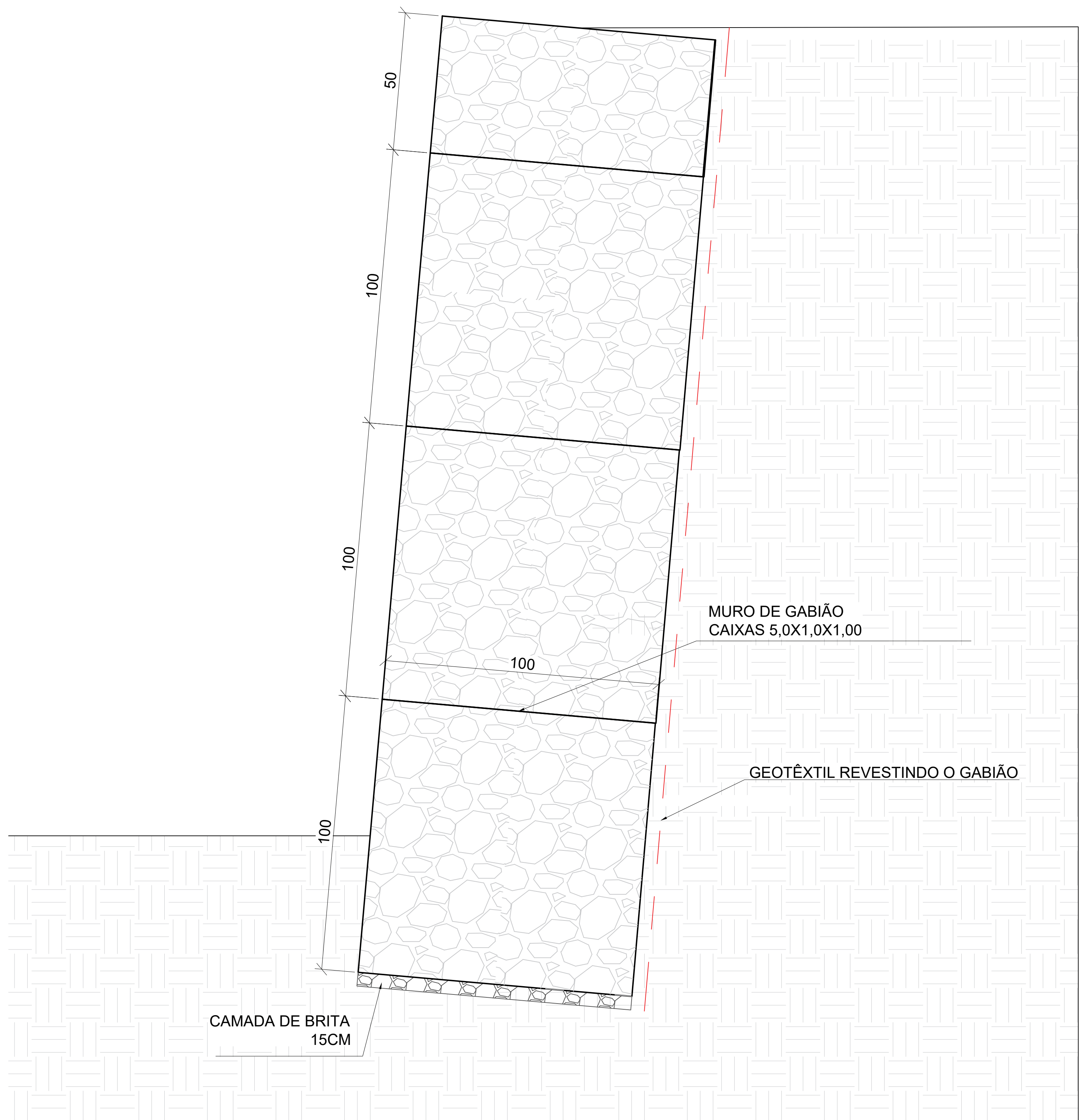
DETALHAMENTO MURO DE GABIÃO - BAIRRO MORRETES
