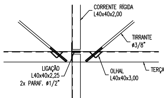
DETALHE DO TRAVAMENTO DAS TERÇAS ESC.: 1/10
