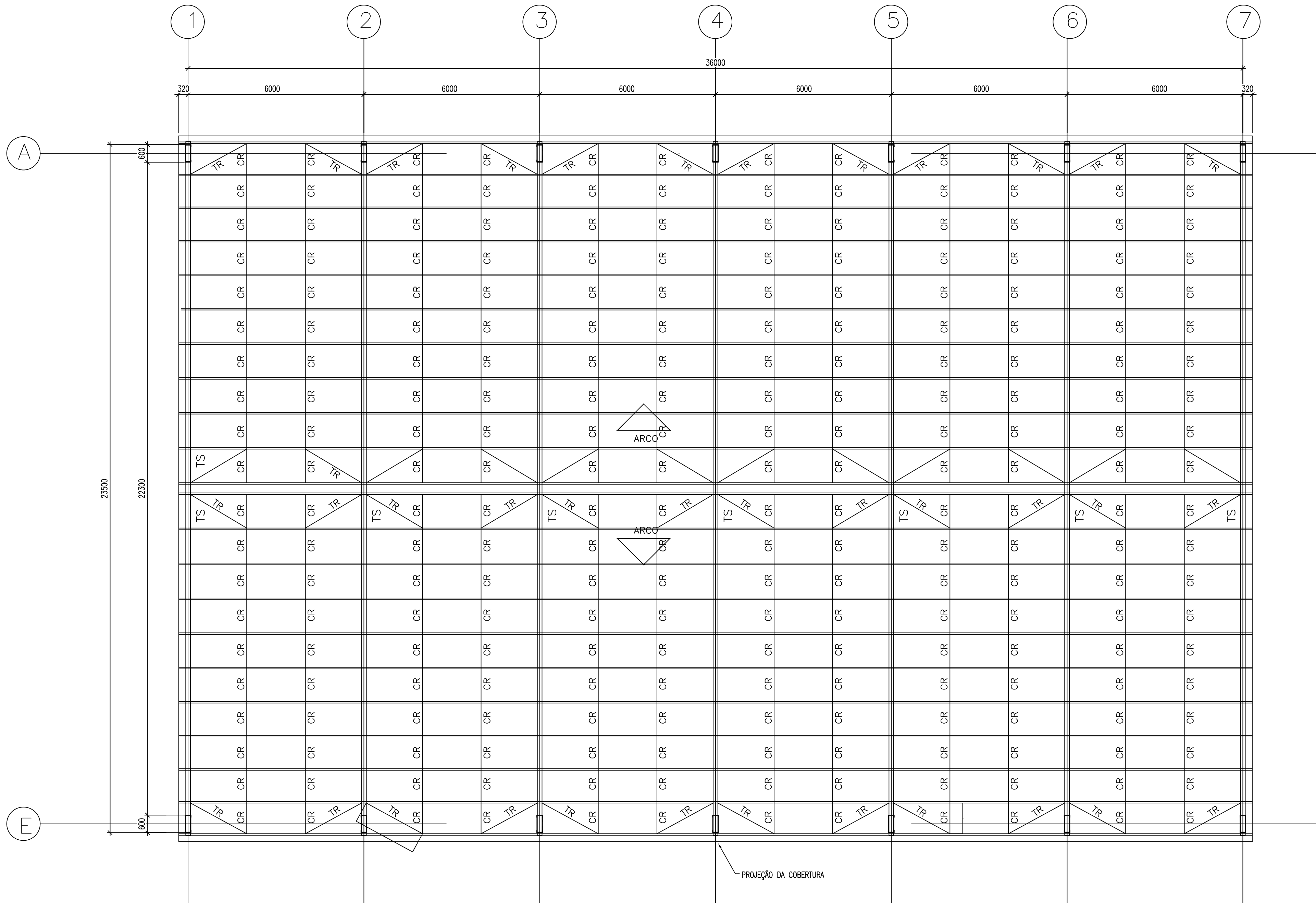
PLANTA – TERÇAS E ACESSÓRIOS DA COBERTURA ESC.:1/125
