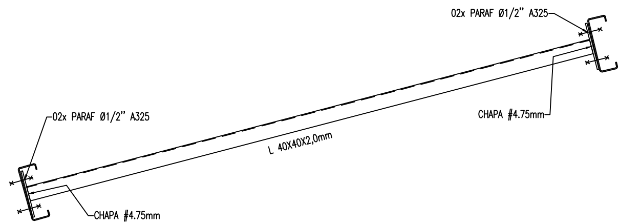
DETALHE TÍPICO DE FIXAÇÃO DAS CORRENTES RÍGIDAS ESC.: 1/10
