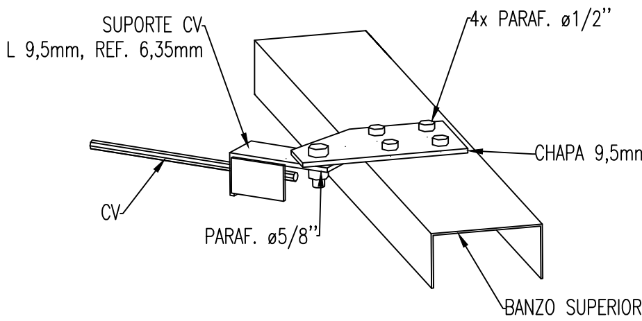
DETALHE FIXAÇÃO CONTRAVENTOS ESC.: 1/10
