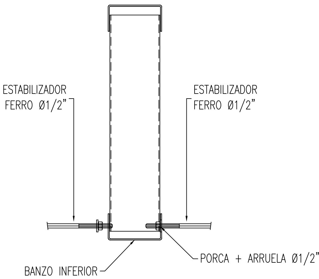
DETALHE ESTABILIZADOR ESC.: 1/10
