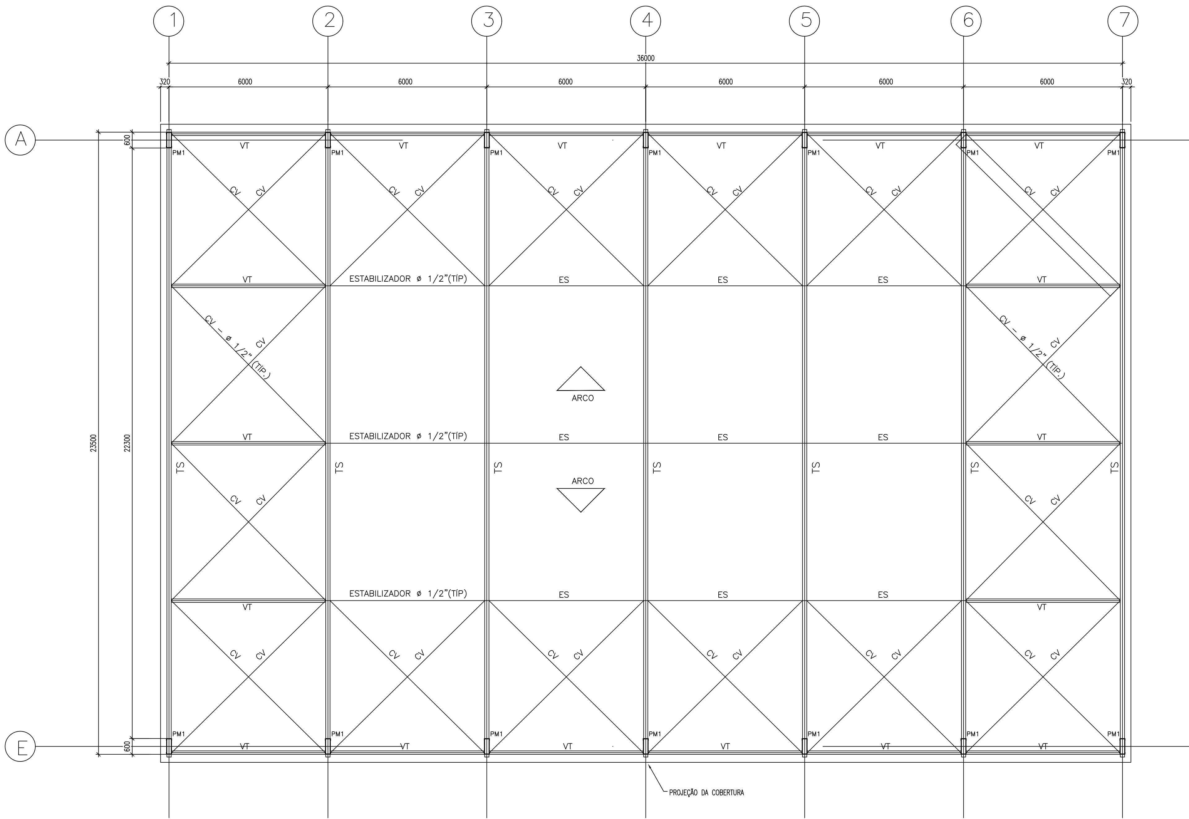
PLANTA – TRAVAMENTO DA COBERTURA ESC.:1/125
