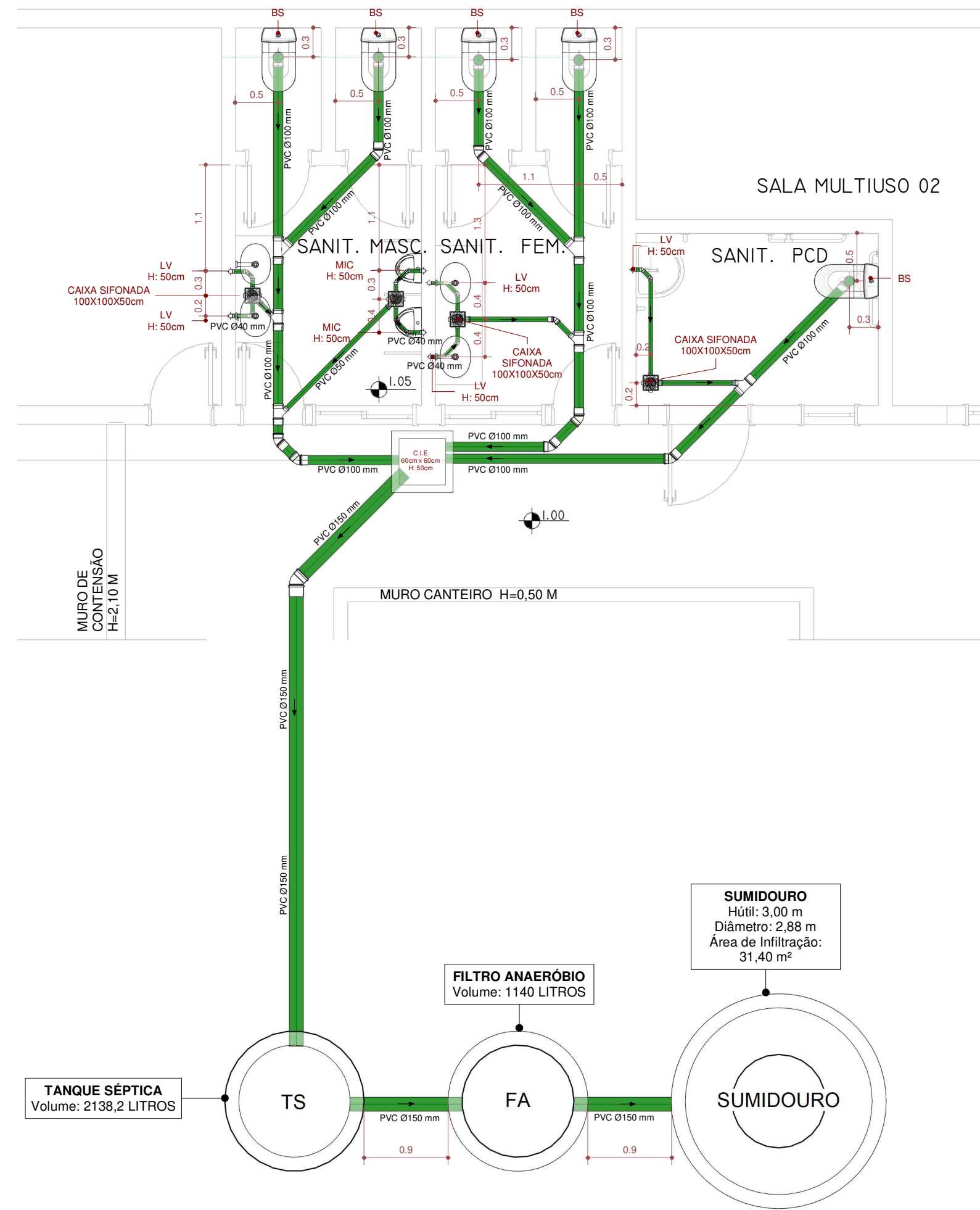
01 Planta Baixa - Quiosque ESCALA: 1 : 50
