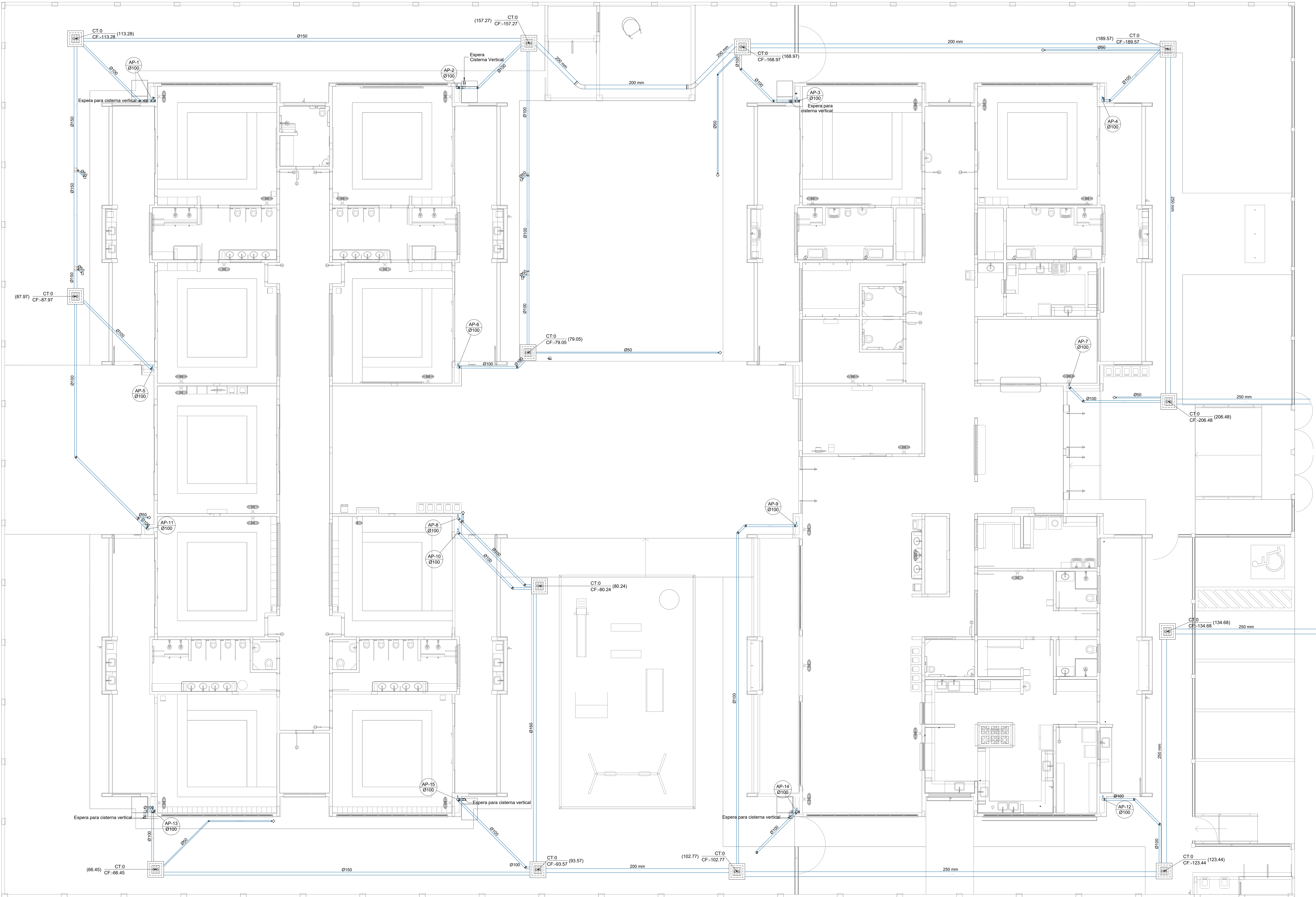
1 PLANTA BAIXA TÉRREO - REDE PLUVIAL ESCALA 1/75
