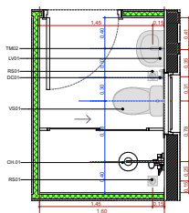
A.M.8 Banh. Func. Masc. Escala 1:25
