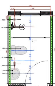
A.M.9 Banh. Func. Fem. Escala 1:25
