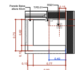
A.M.10 Higienização dos pés Escala 1:25
