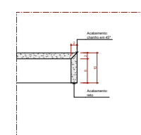
Det. B.7.b Bancada de Plástico Detalhe Lateral Escala 1:5
