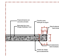
Det. B.1.b Bancada de Inox Detalhe Lateral - Área Molhada Escala 1:5
