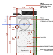
BPC.120e Escala 1:20
