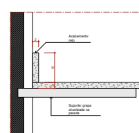
Det. B.7.a Bancada de Plástico Detalhe Frontal Escala 1:5
