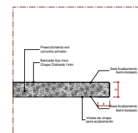
Det. B.1.d Bancada de Inox Detalhe Lateral - Área Seca Escala 1:5
