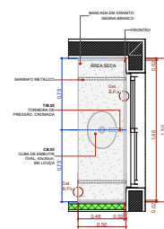
BPC.150de-Escovário Escala 1:20
