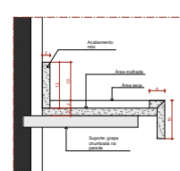
Det. B.7.c Bancada de Plástico Detalhe Lateral - Área Molhada Escala 1:5
