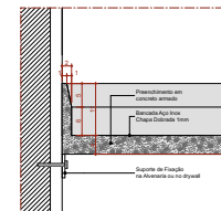
Det. B.1.a Bancada de Inox Detalhe Frontal - Área Molhada Escala 1:5
