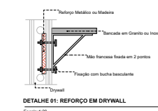
DETALHE 01: REFORÇO EM DRYWALL Escala 1:20
