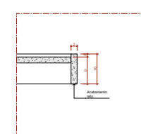
Det. B.7.d Bancada de Plástico Detalhe Lateral - Área Molhada Escala 1:5
