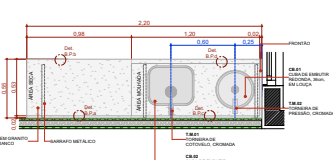
BPC.150de-Escovário Escala 1:20
