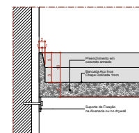
Det. B.1.c Bancada de Inox Detalhe Frontal - Área Seca Escala 1:5
