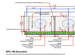
BPC.180-Escovário Escala 1:20
