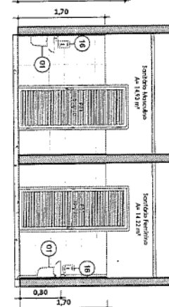
B. Lavatórios - Sanitário Lateral ESCALA 1:50
