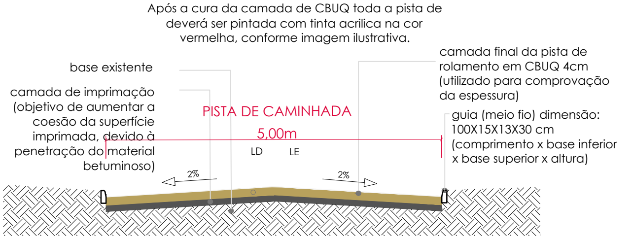
DET 01 | PERFIL DA PISTA DE CAMINHADA
