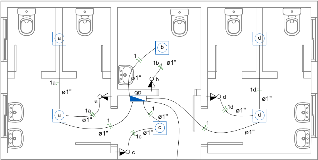
PLANTA ELÉTRICA esc 1:50
