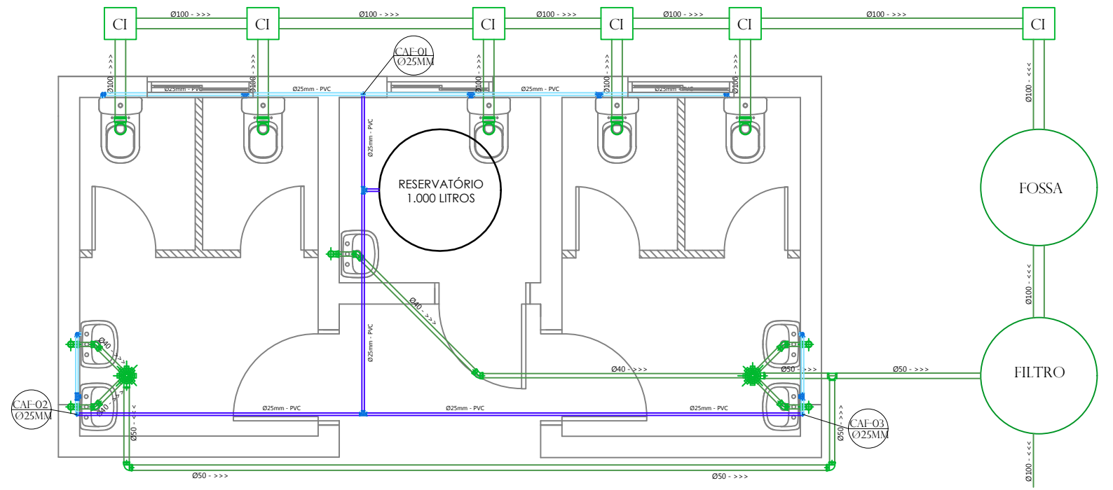
PLANTA BAIXA - INSTALAÇÕES HIDROSSANITÁRIAS esc 1:50
