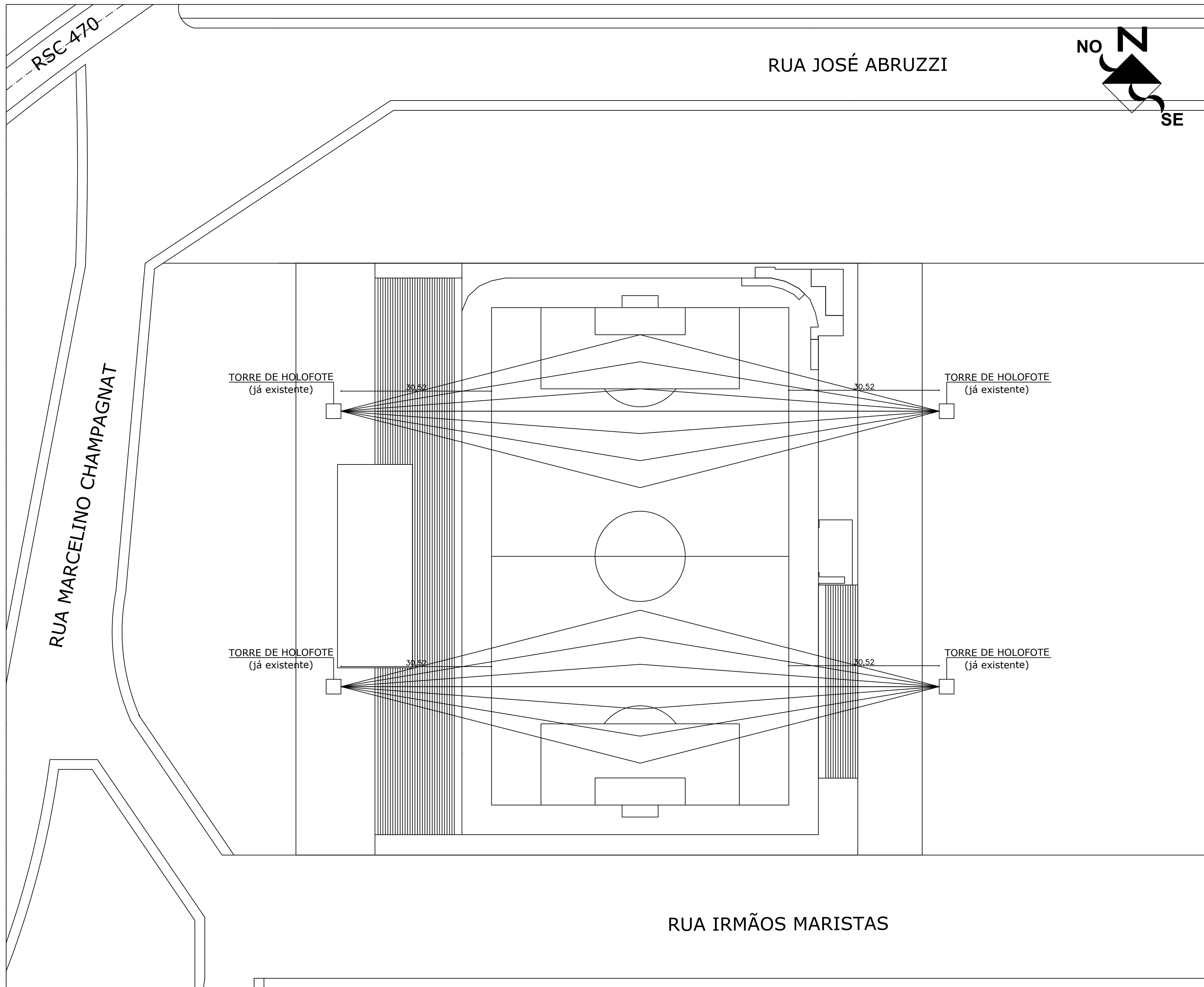
Planta de Localização e Elétrico Escala 1/500
