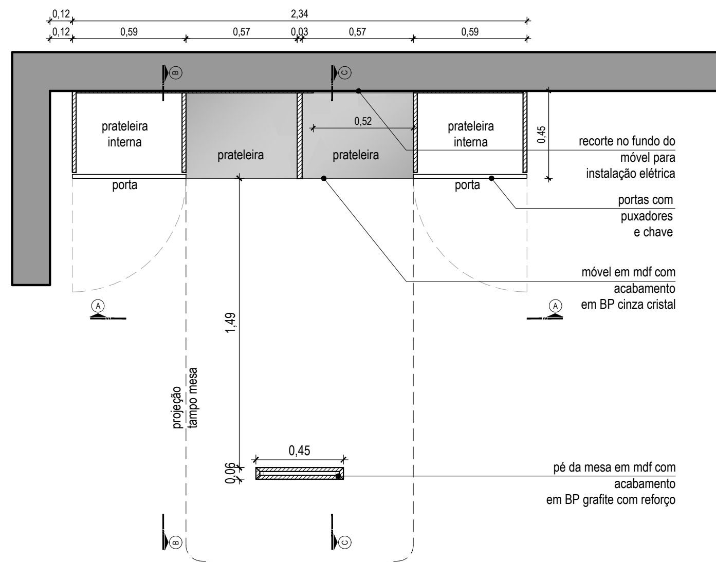
PLANTA BAIXA - ALTURA = 0,60m ESC: 1/20
