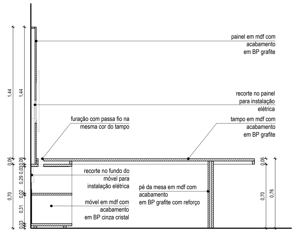
CORTE CC ESC: 1/20
