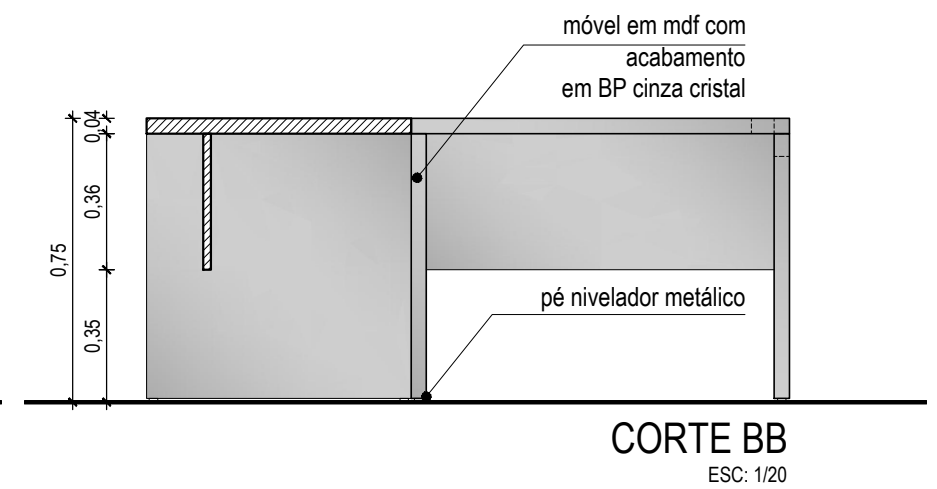
VISTA 2 ESC: 1/20
