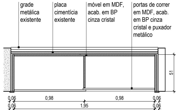
PLANTA BAIXA ESC: 1/25
