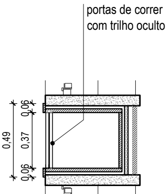
CORTE TRANSVERSAL ESC: 1/25
