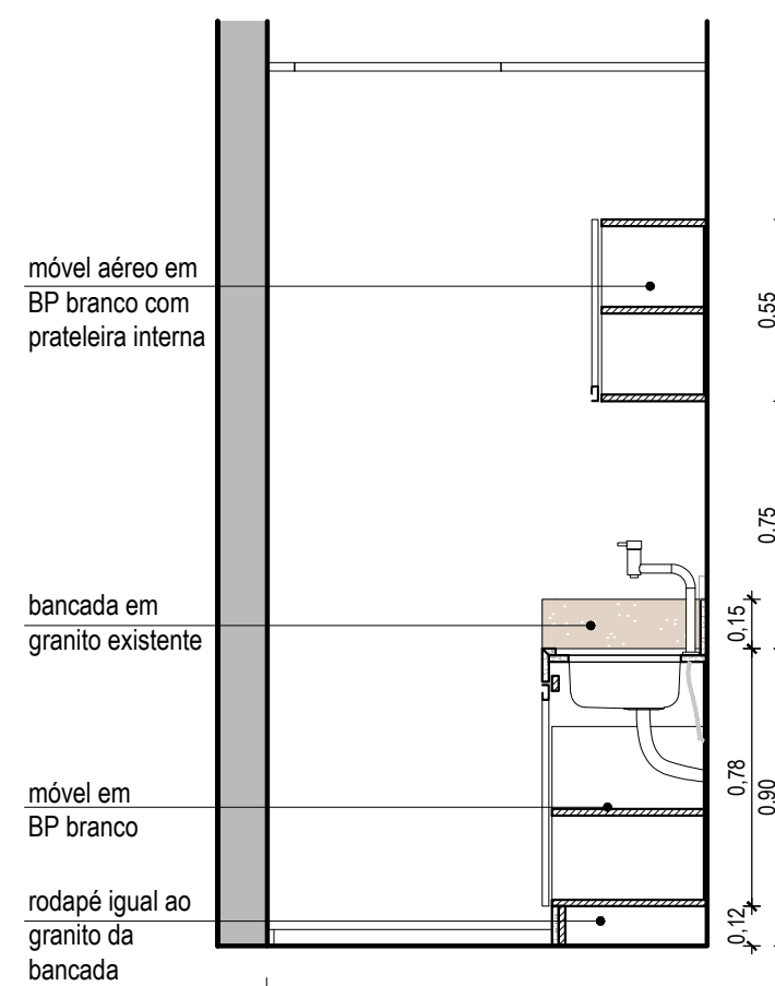
05 CORTE BB ESC: 1/25
