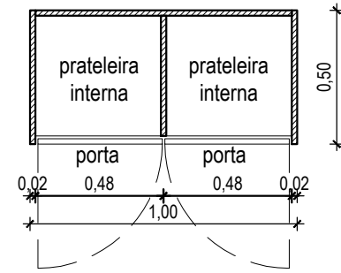
09 PLANTA BAIXA - ALTURA = 100cm ESC: 1/25
