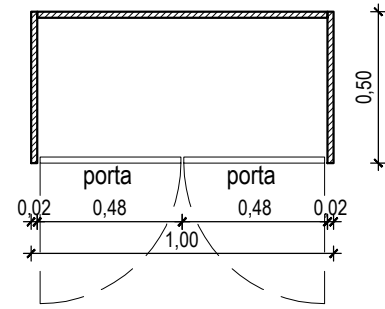
08 PLANTA BAIXA - ALTURA = 50cm ESC: 1/25
