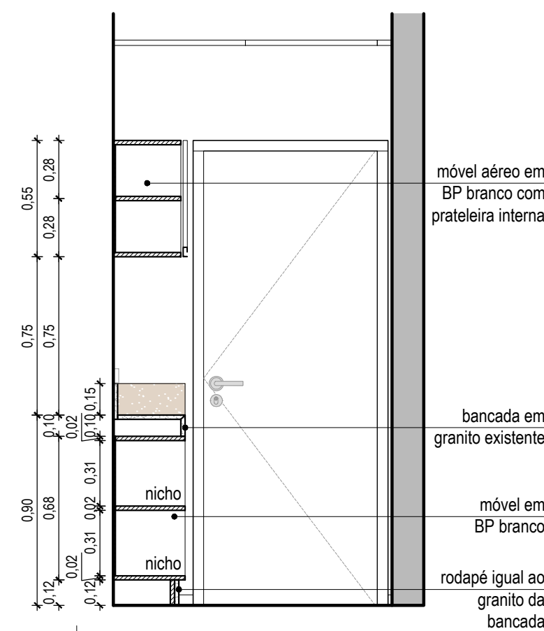
06 CORTE CC ESC: 1/25
