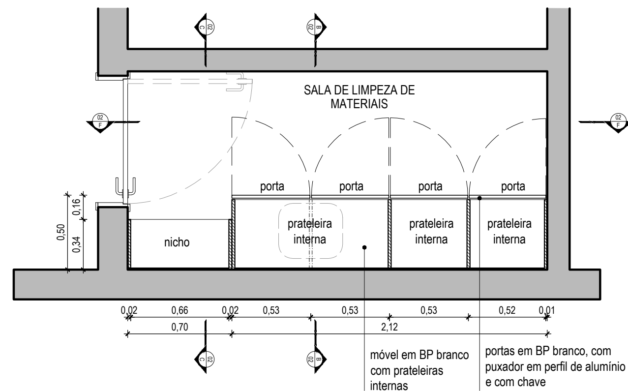
02 PLANTA BAIXA - ALTURA = 60cm ESC: 1/25
