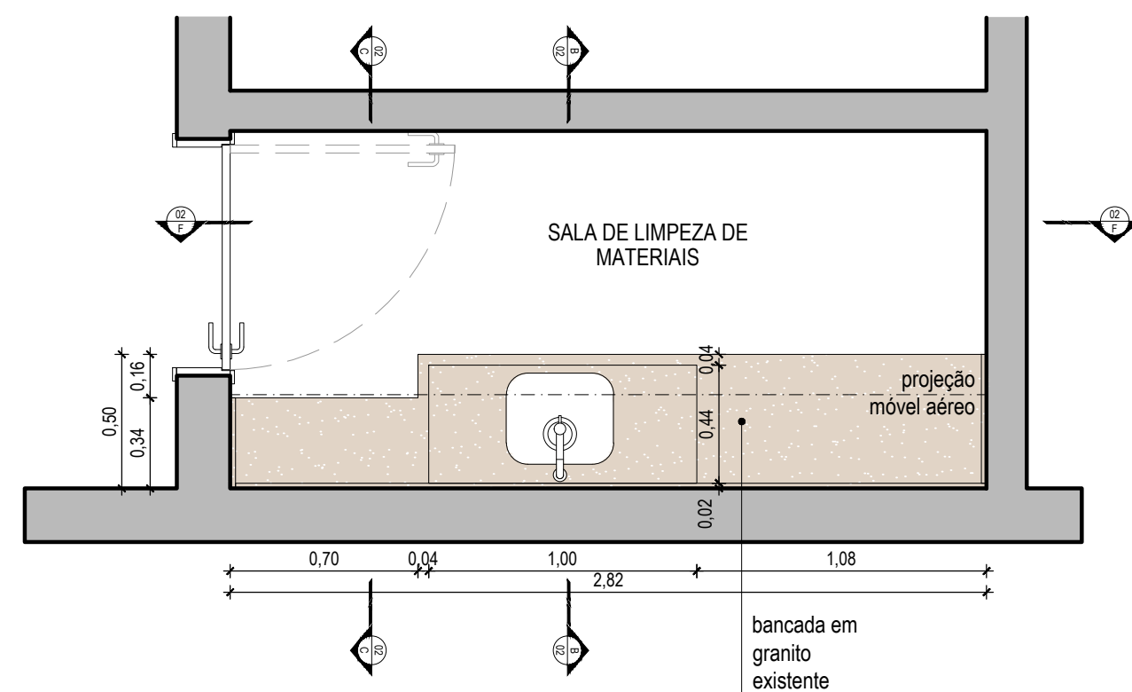
03 PLANTA BAIXA - ALTURA = 120cm ESC: 1/25
