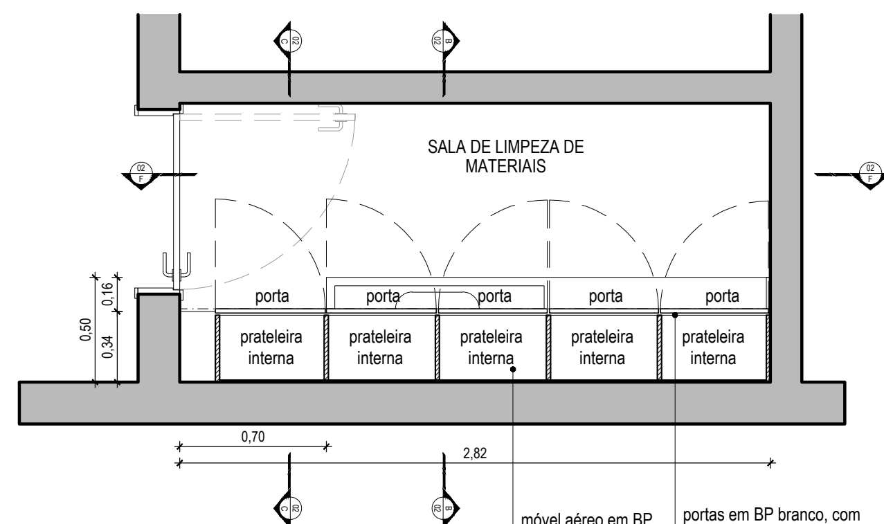
04 PLANTA BAIXA - ALTURA = 180cm ESC: 1/25
