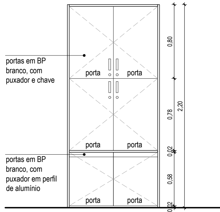
10 VISTA FRONTAL - EXTERNA ESC: 1/25
