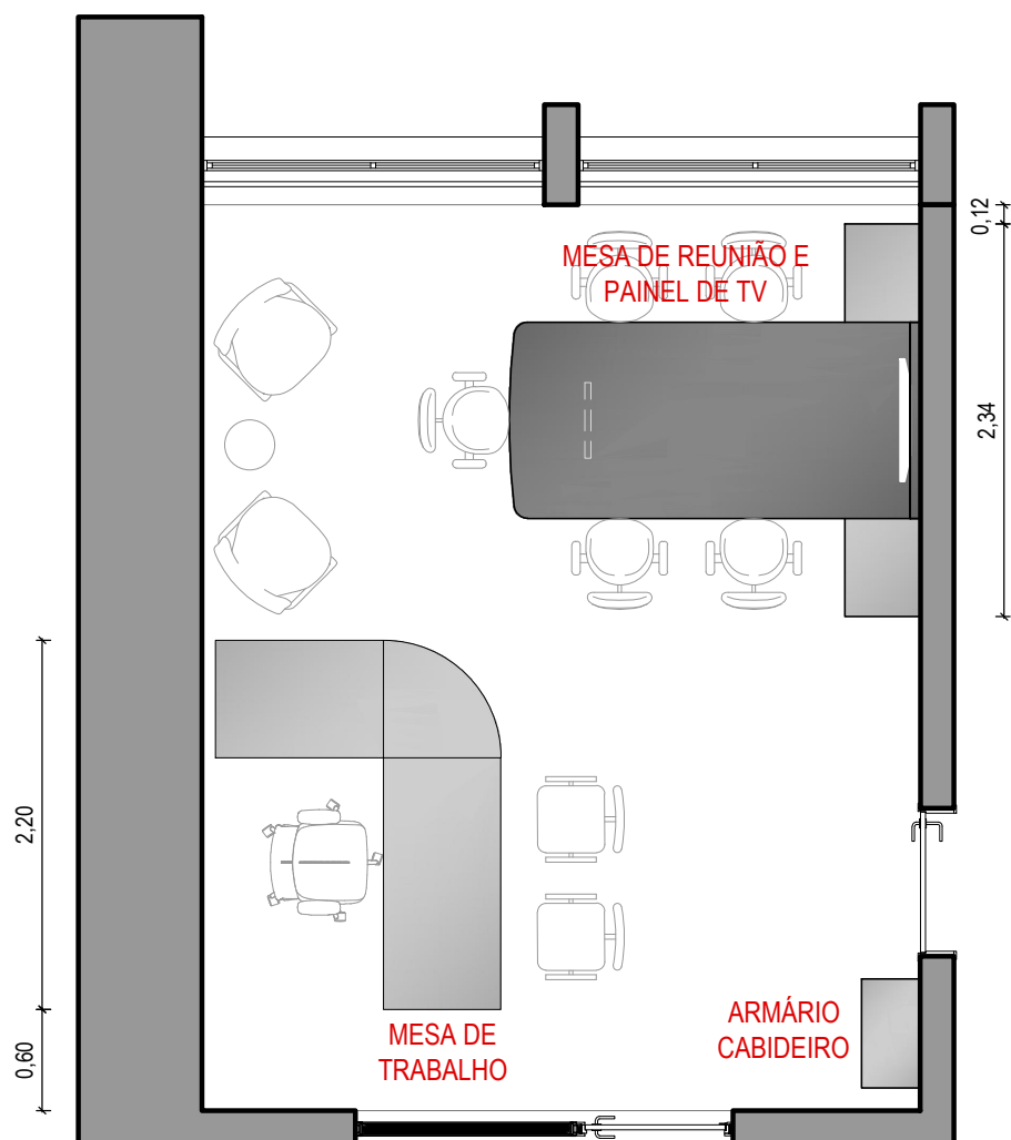
SALA 102 DIRETORIA ADMINISTRATIVA ESC: 1/50
