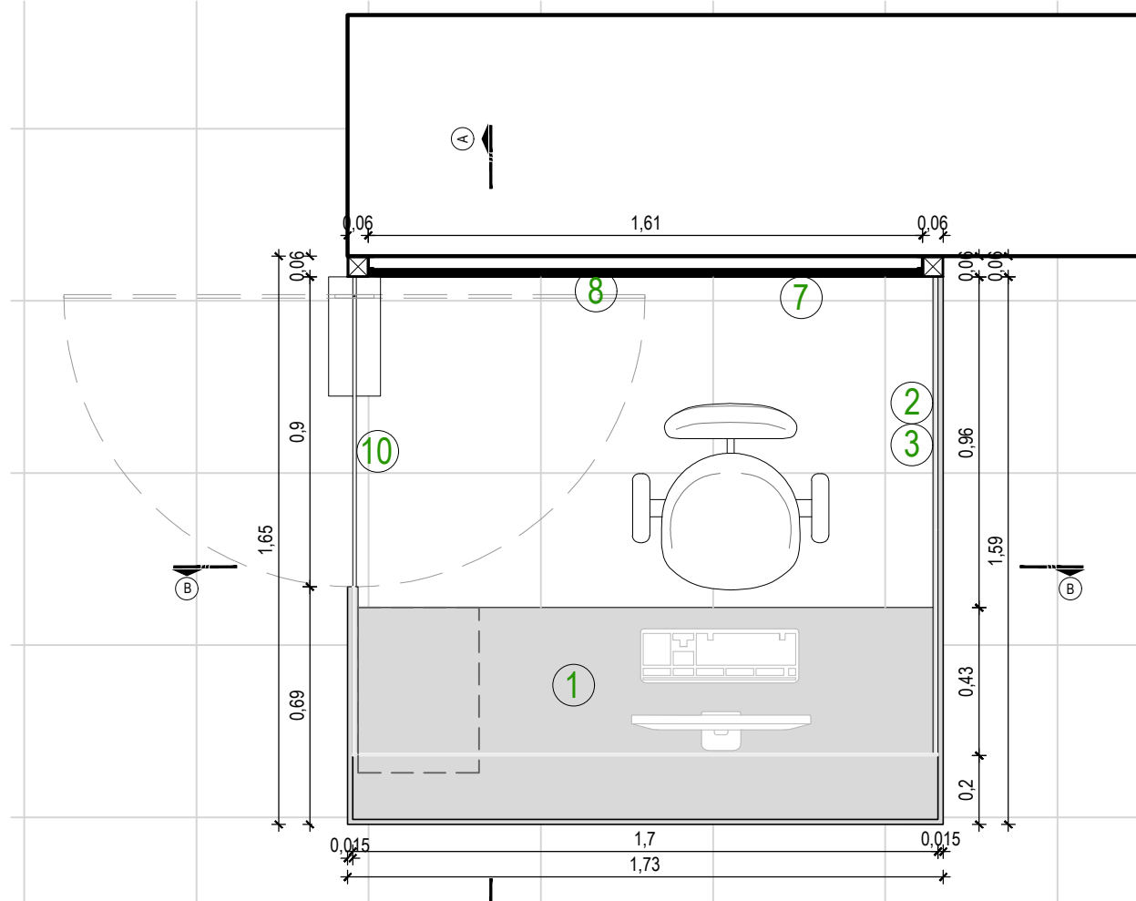
PLANTA BAIXA - 120 cm ESC: 1/20
