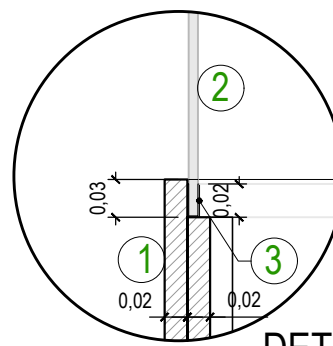
DET. 02 ESC: 1/5
