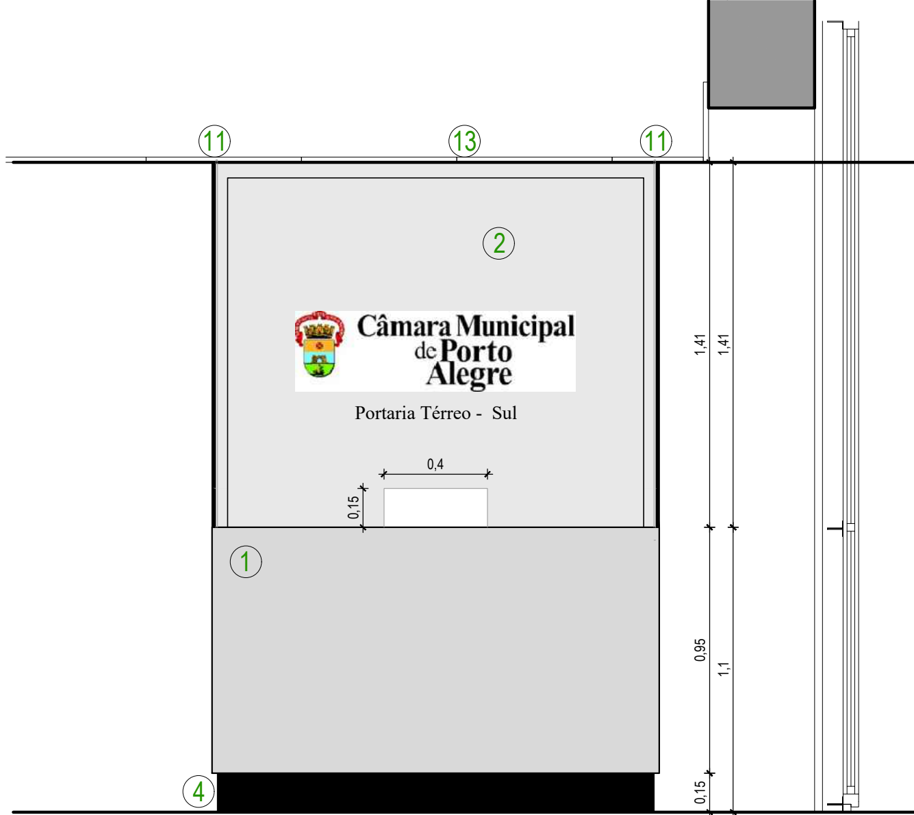
VISTA FRONTAL ESC: 1/20
