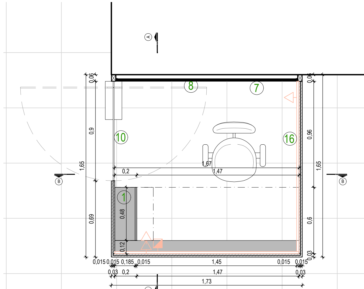
PLANTA BAIXA - 40 cm ESC: 1/20
