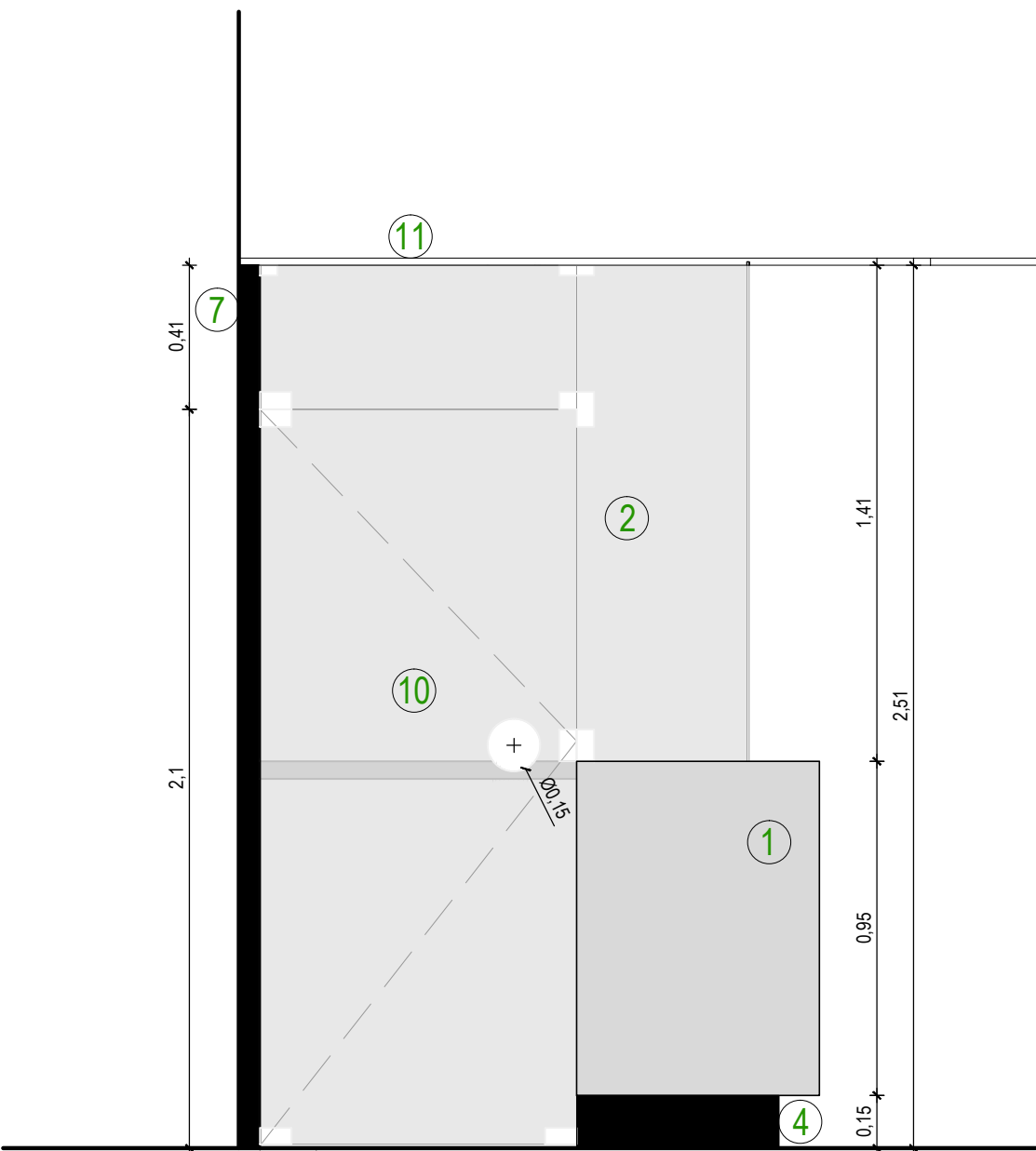
VISTA LATERAL ESC: 1/20
