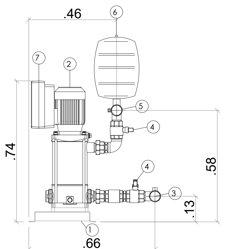
CORTE A
