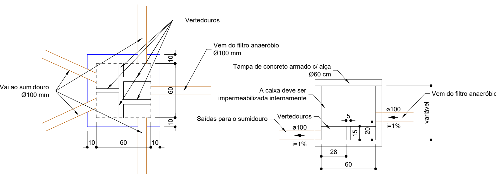
Planta Baixa
