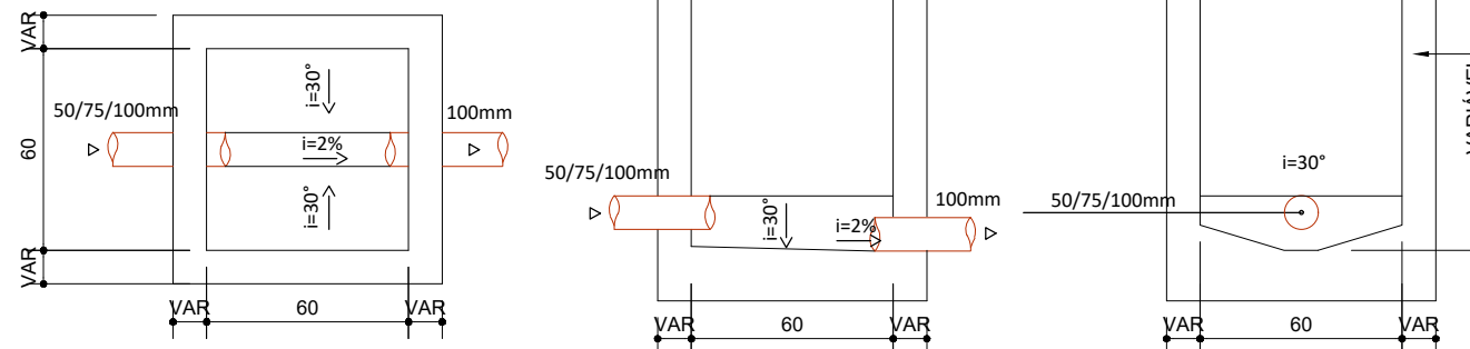
PLANTA BAIXA
