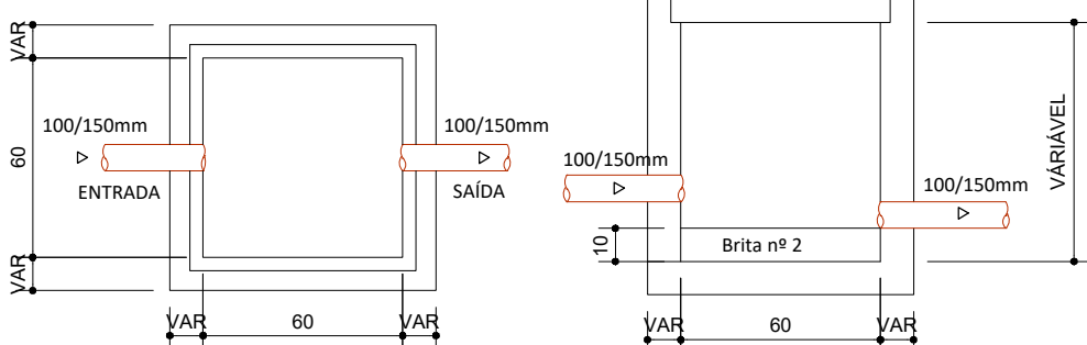
PLANTA BAIXA
