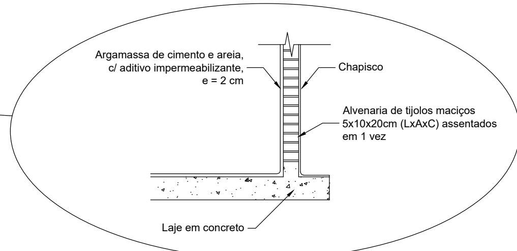
Detalhe de impermeabilização do tanque séptico e do filtro anaeróbio
