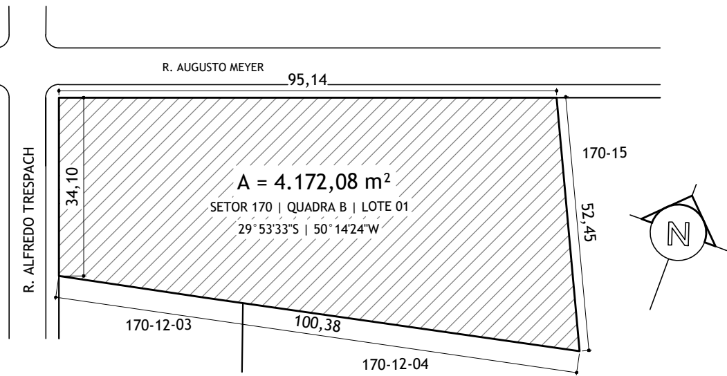
1 SITUAÇÃO 1:1000
