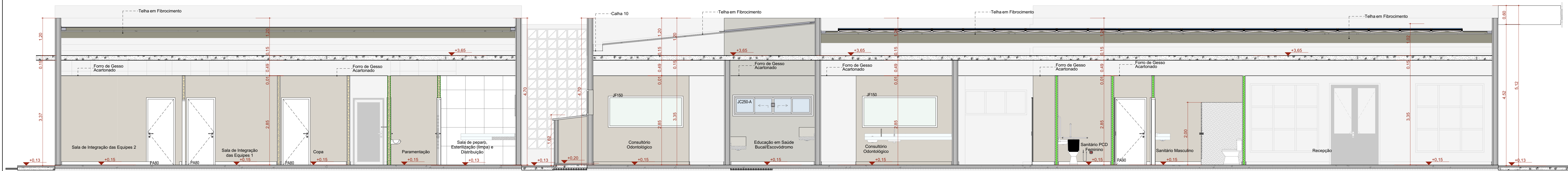
E Corte EE
