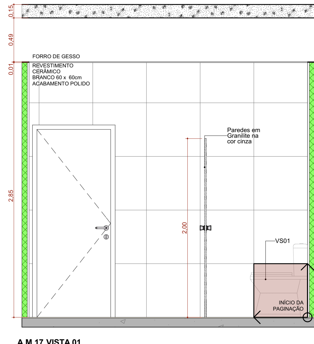
A.M.17 VISTA 01 Escala: 1:25
