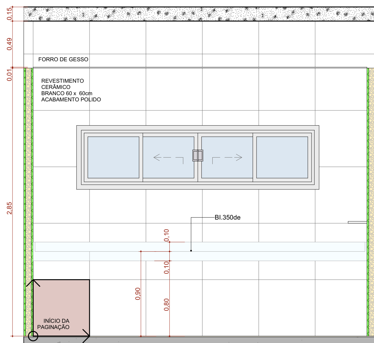
A.M.15 VISTA 04 Escala: 1:25
