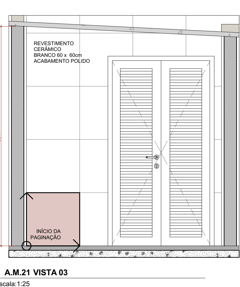
A.M.21 VISTA 03 Escala:1:25
