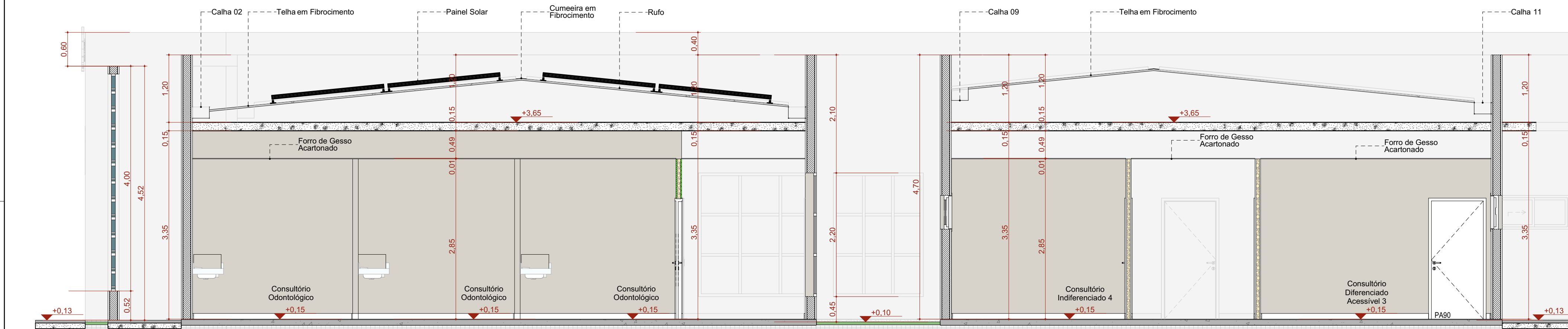
B Corte BB
