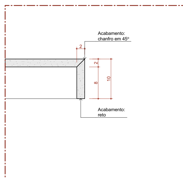
Det. B.P.b Bancada de Pedra Detalhe Sala Escala: 1:5
