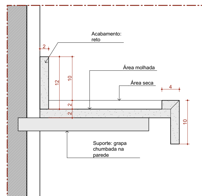
Det. B.P.c Bancada de Pedra Detalhe área molhada Escala: 1:5
