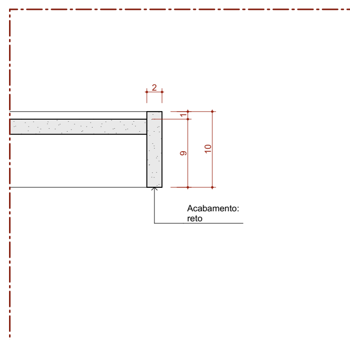
Det. B.P.d Bancada de Pedra Detalhe área molhada Escala: 1:5
