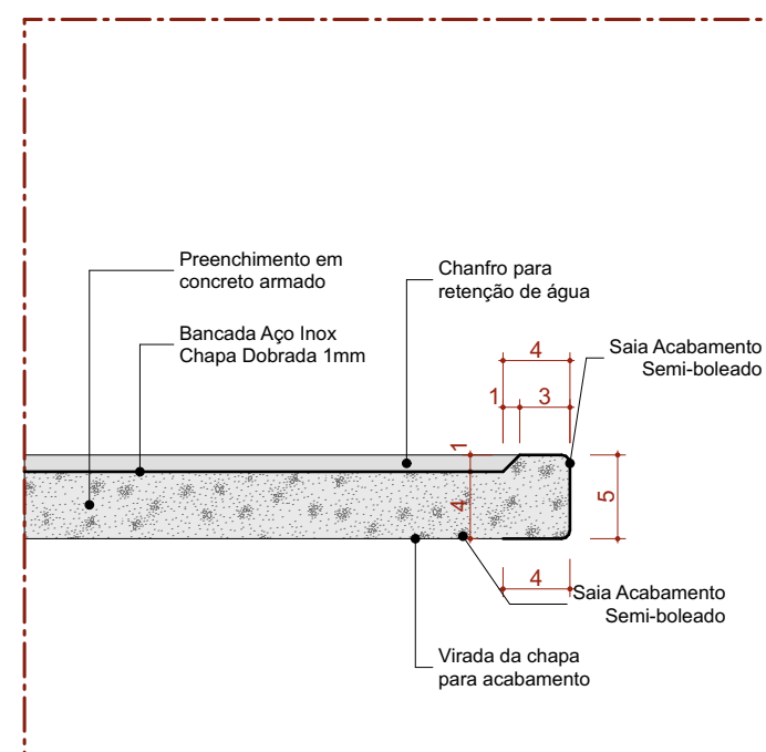
Det. B.I.b Bancada de Inox Detalhe Sala - Área Molhada Escala: 1:5
