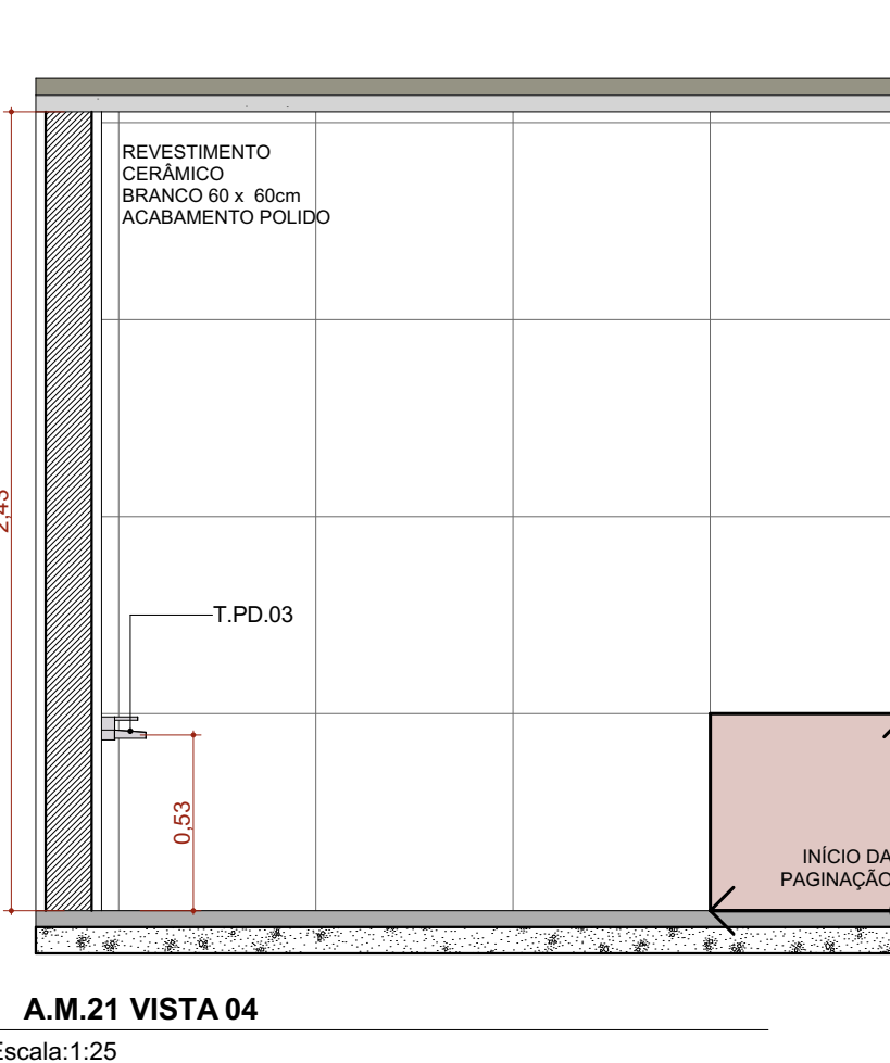
A.M.21 VISTA 04 Escala:1:25
