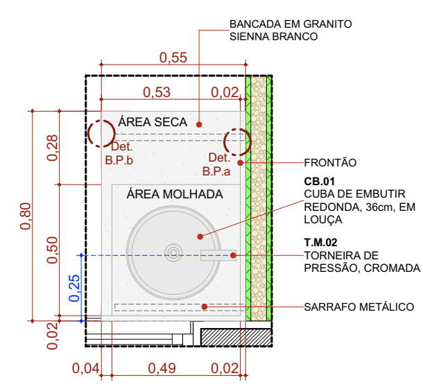
BPC.80d Escala: 1:20
