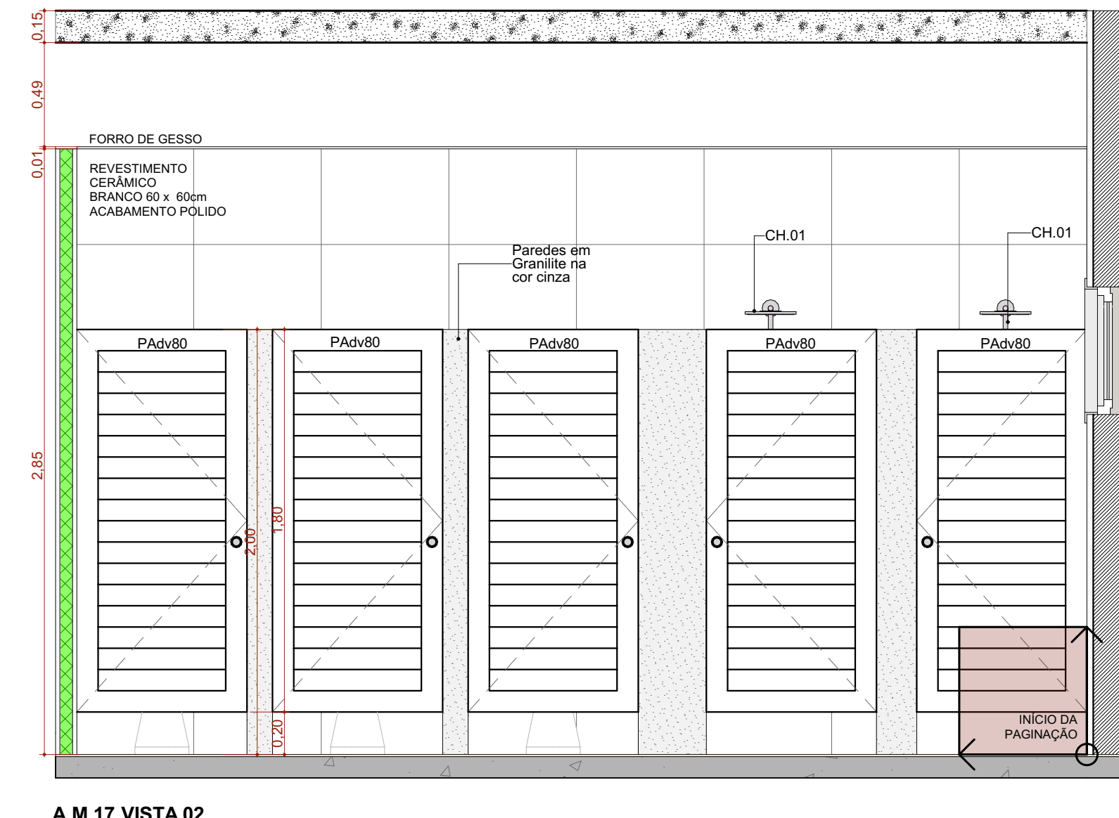
A.M.17 VISTA 02 Escala: 1:25
