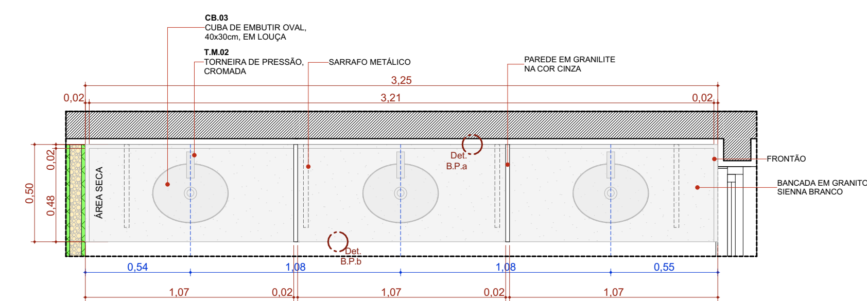
BPC.325de-Escovodromo Escala: 1:20
