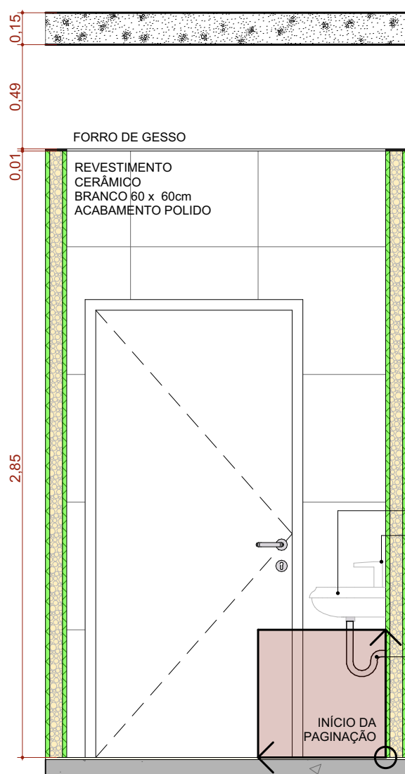
A.M.14 VISTA 02 Escala: 1:25
