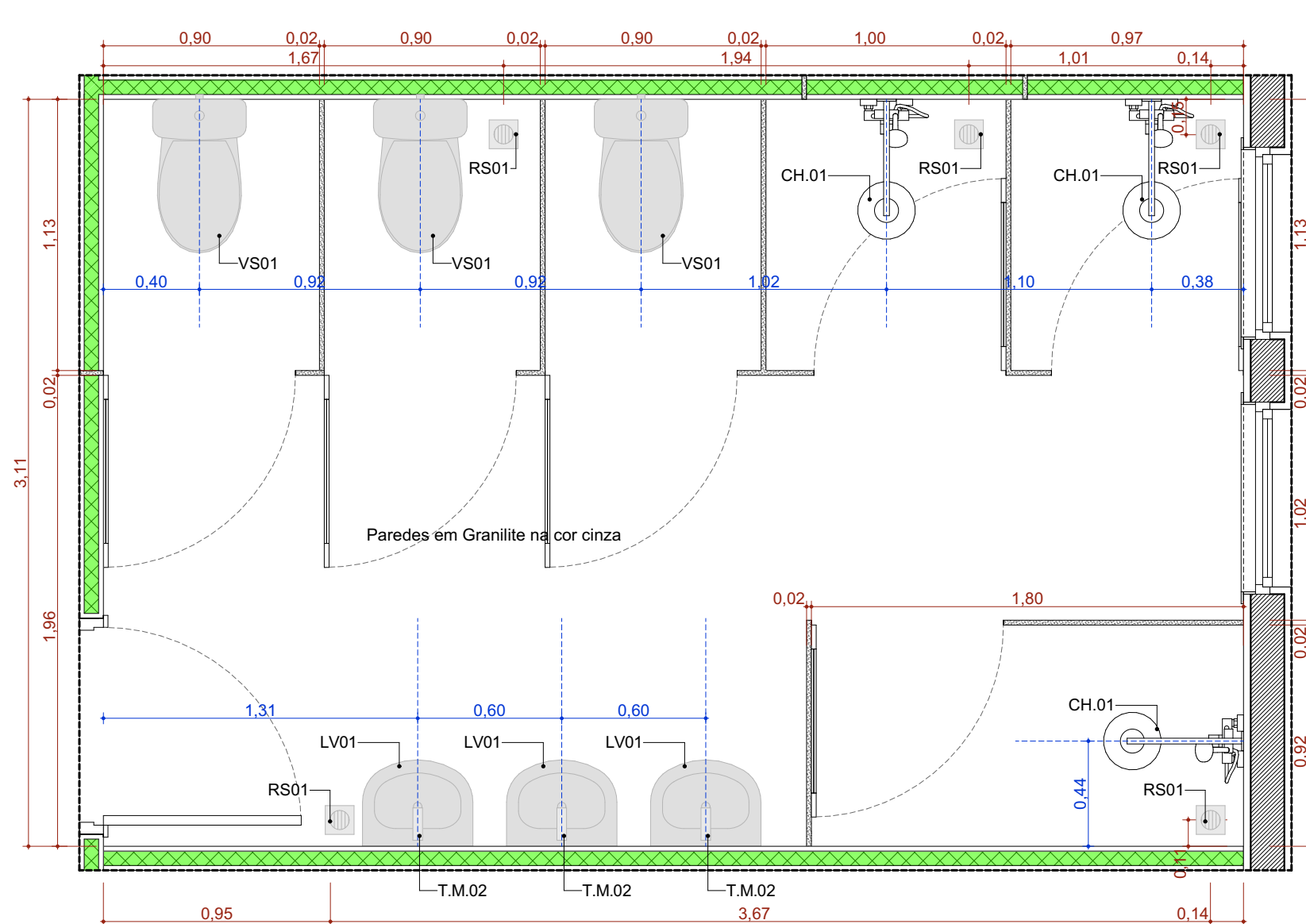
A.M.17 Banheiro de Funcionários Feminino Escala: 1:25
