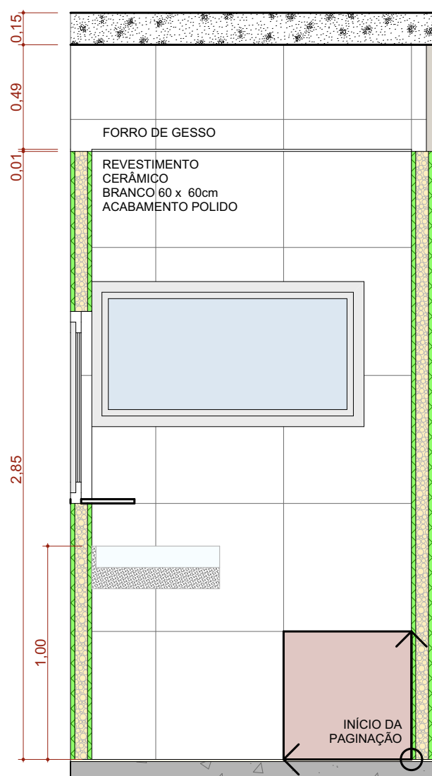
A.M.14 VISTA 04 Escala: 1:25
