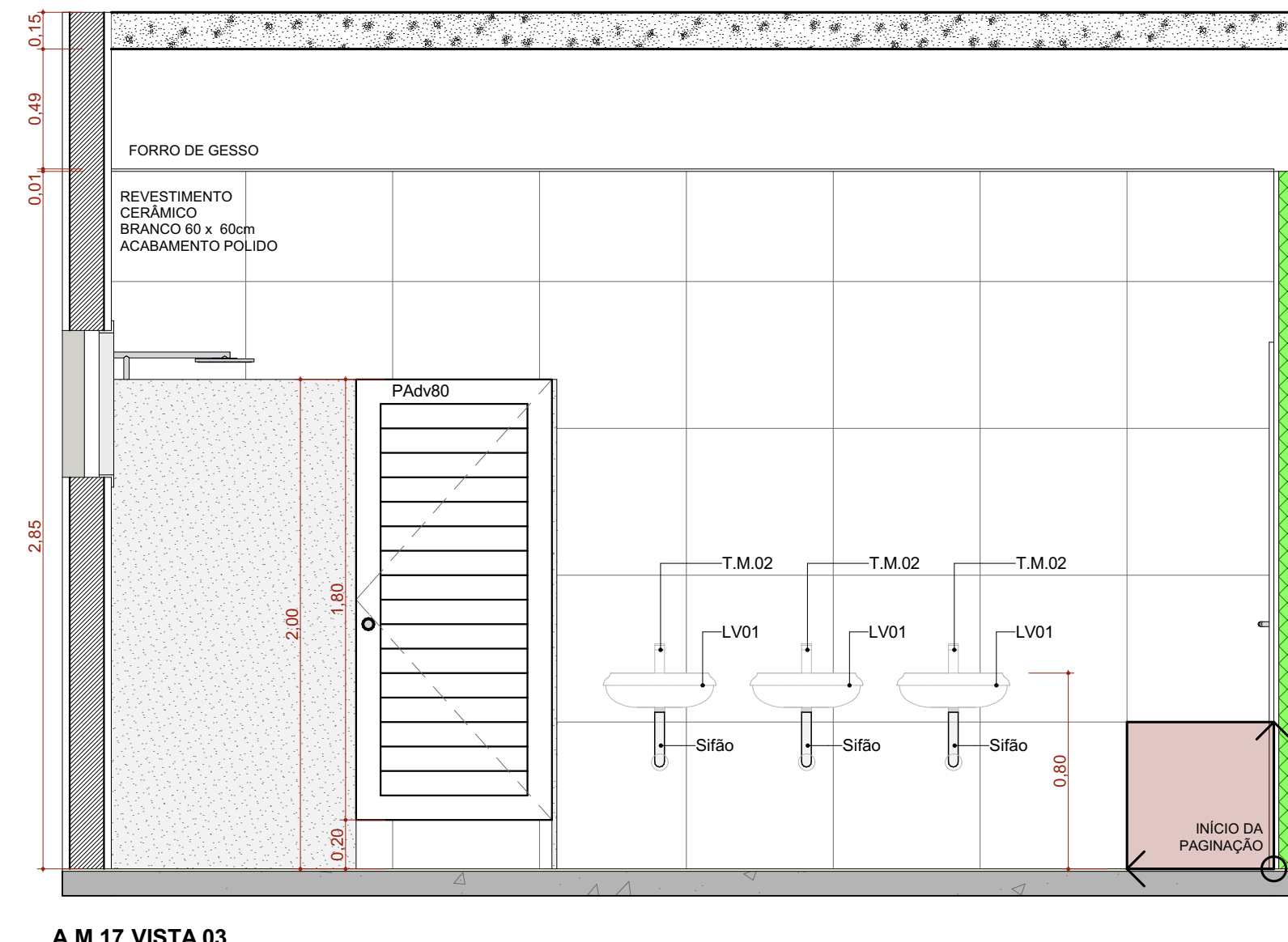
A.M.17 VISTA 03 Escala: 1:25
