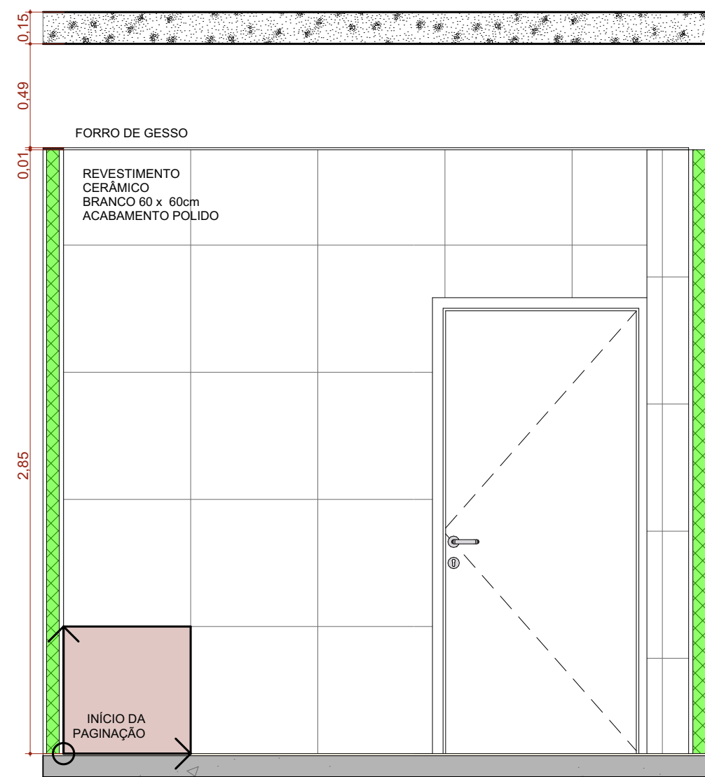
A.M.19 VISTA 01 Escala:1:25
