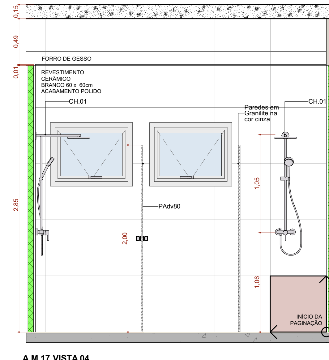
A.M.17 VISTA 04 Escala: 1:25
