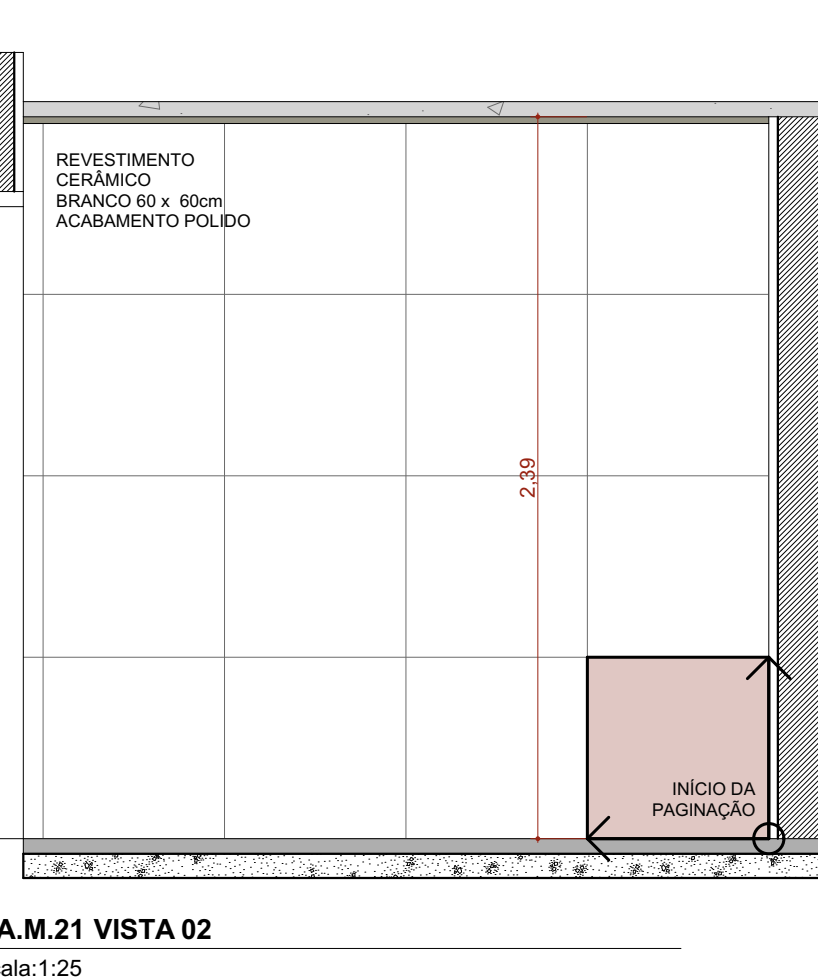
A.M.21 VISTA 02 Escala:1:25
