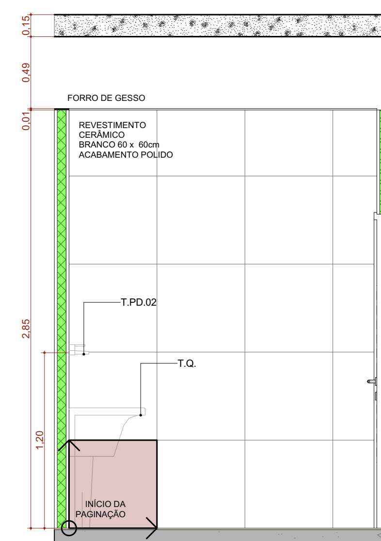
A.M.16 VISTA 03 Escala: 1:25
