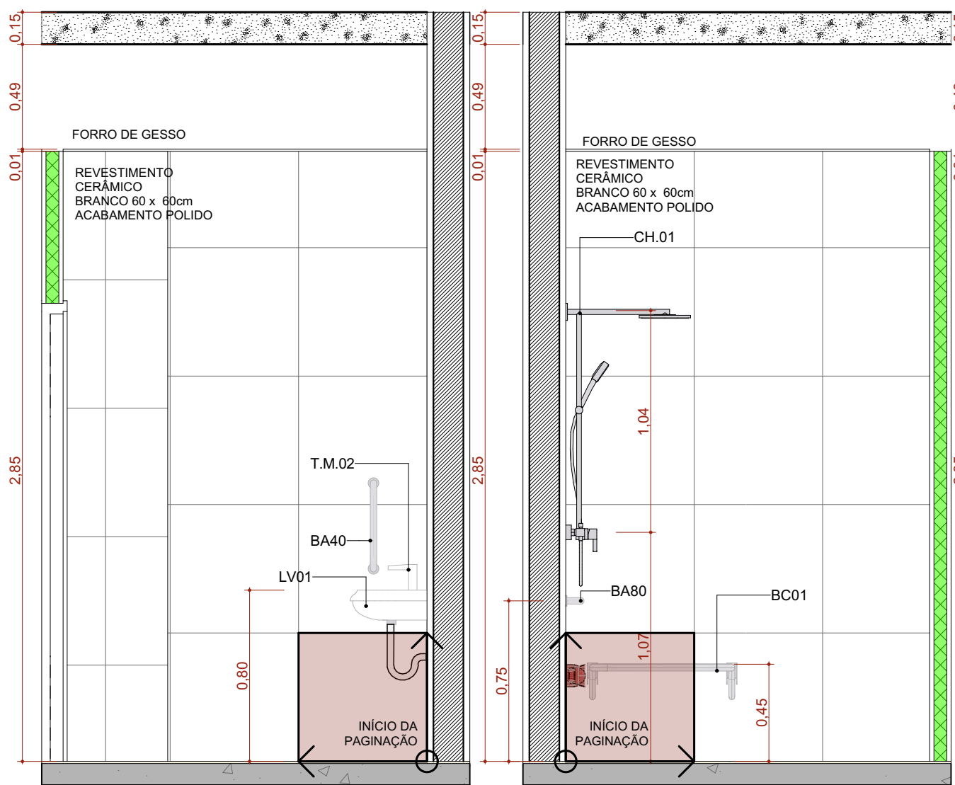
A.M.19 VISTA 02 Escala:1:25
