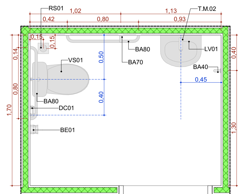
A.M.07 Sanitário PCD Feminino
