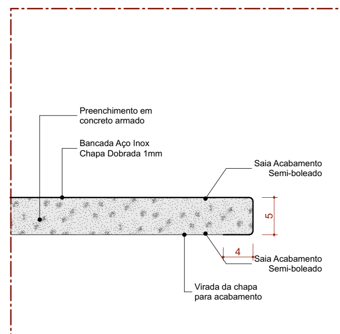
Det. B.I.d Bancada de Inox Detalhe Sala - Área seca Escala: 1:5
