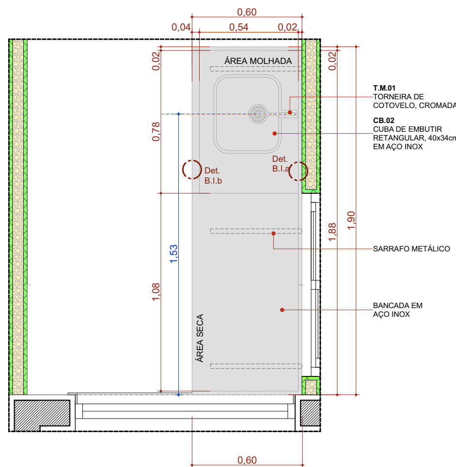
BIC.190d Escala: 1:20
