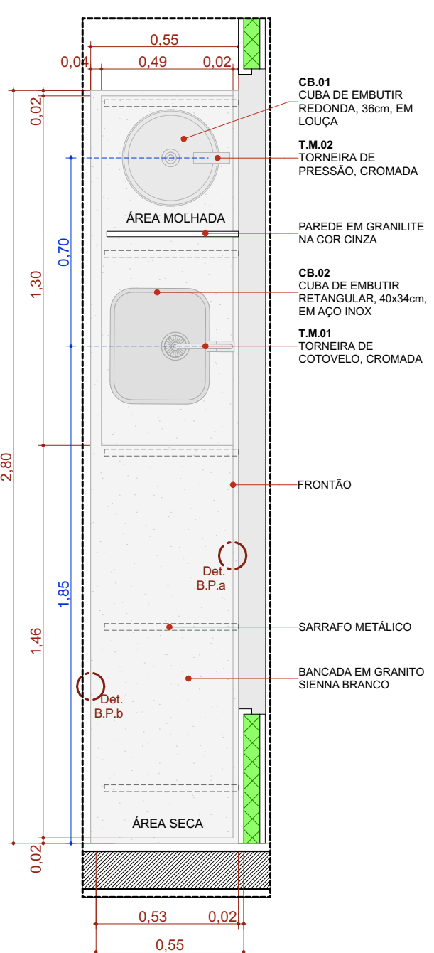
BPC.280d Escala: 1:20
