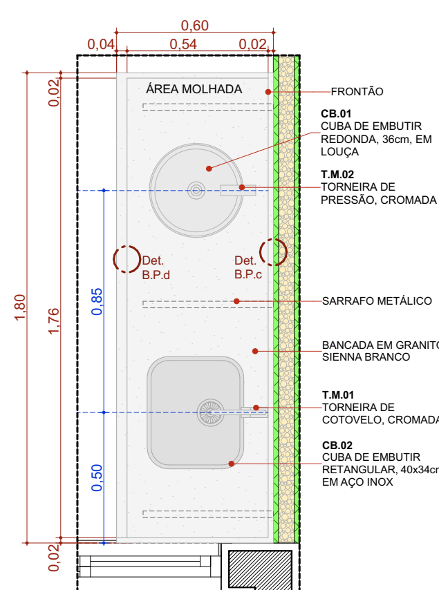
BPC2.180d Escala: 1:20
