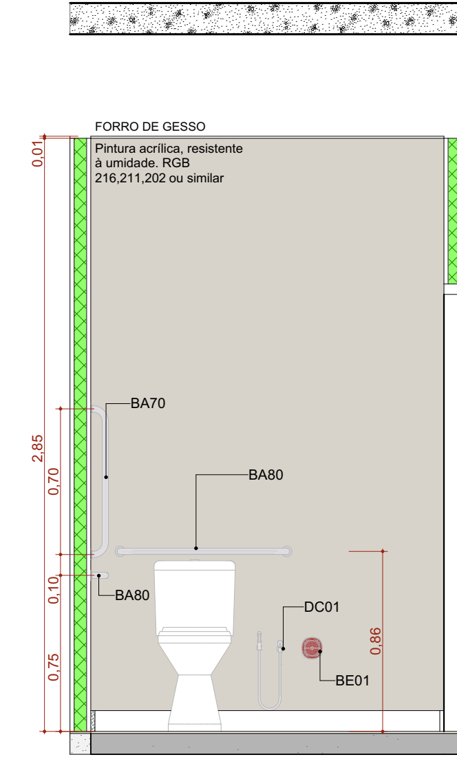
A.M.06 VISTA 04 Escala: 1:25
