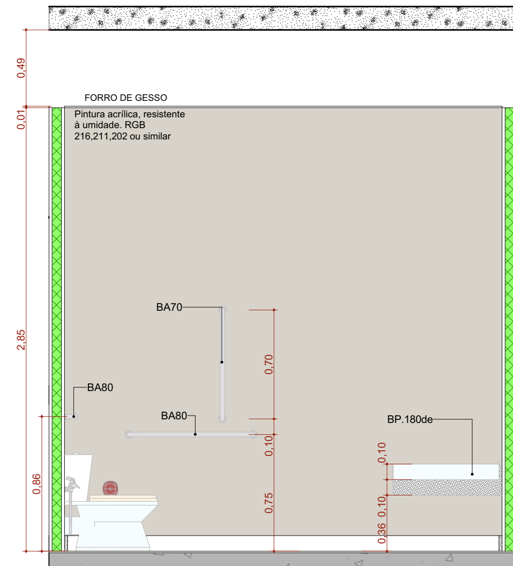
A.M.01 VISTA 04 Escala: 1:25
