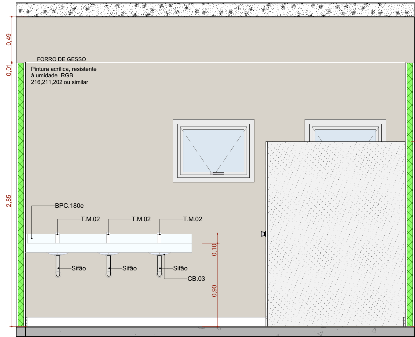
A.M.03 VISTA 02 Escala: 1:25
