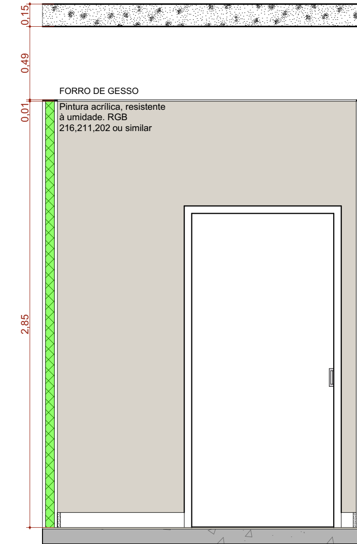
A.M.06 VISTA 03 Escala: 1:25
