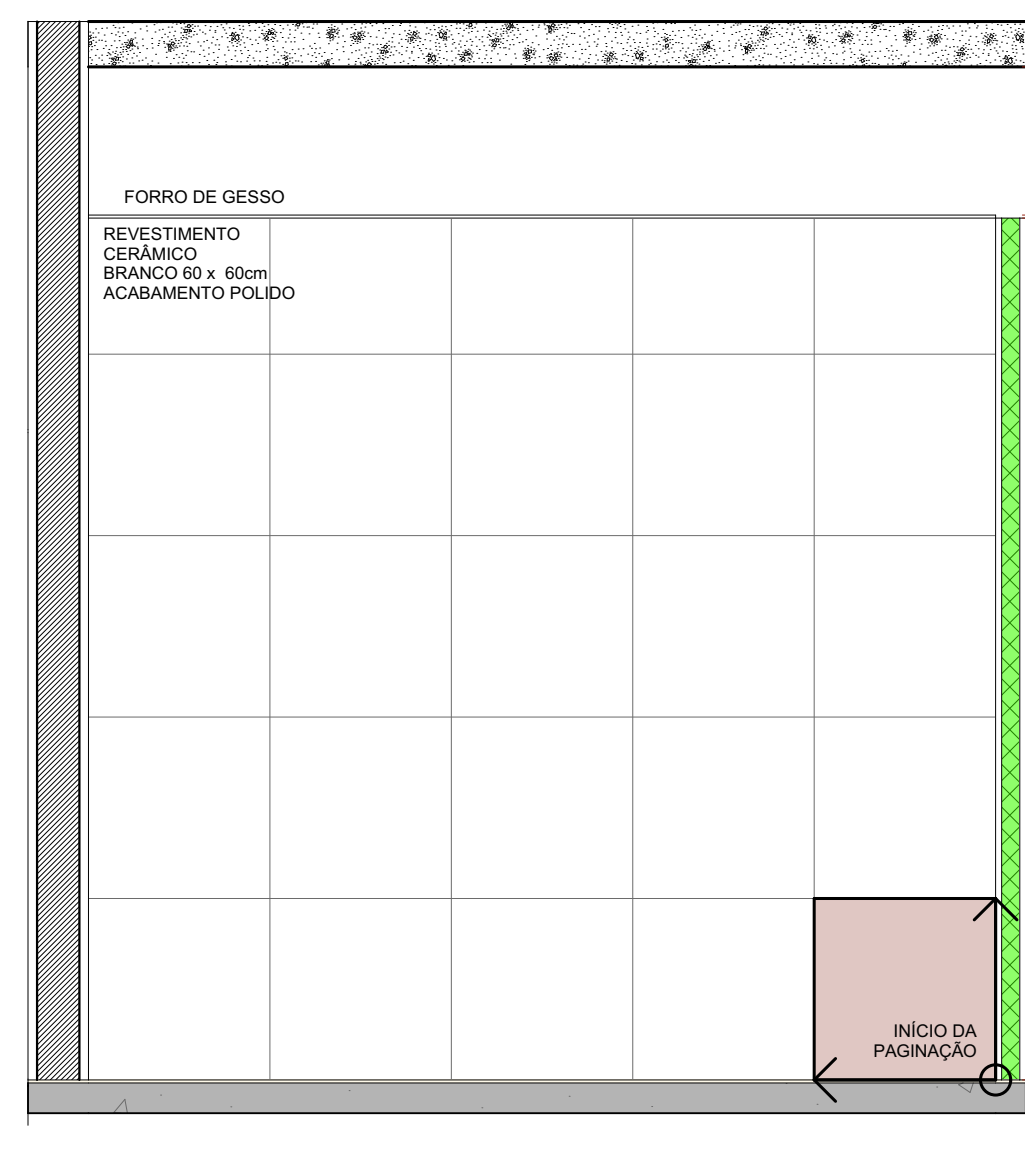
A.M.04 VISTA 02 Escala: 1:25
