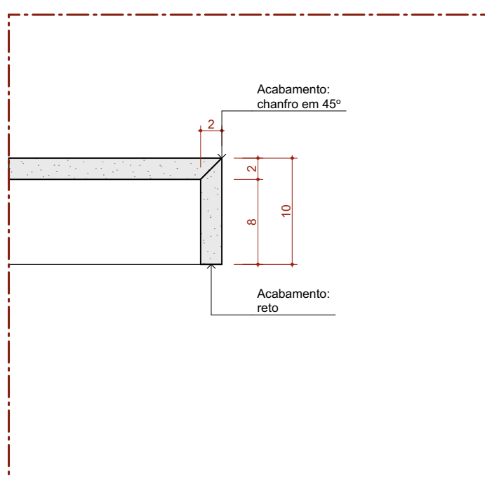
Det. B.P.b Bancada de Pedra Detalhe Sala Escala 1:5
