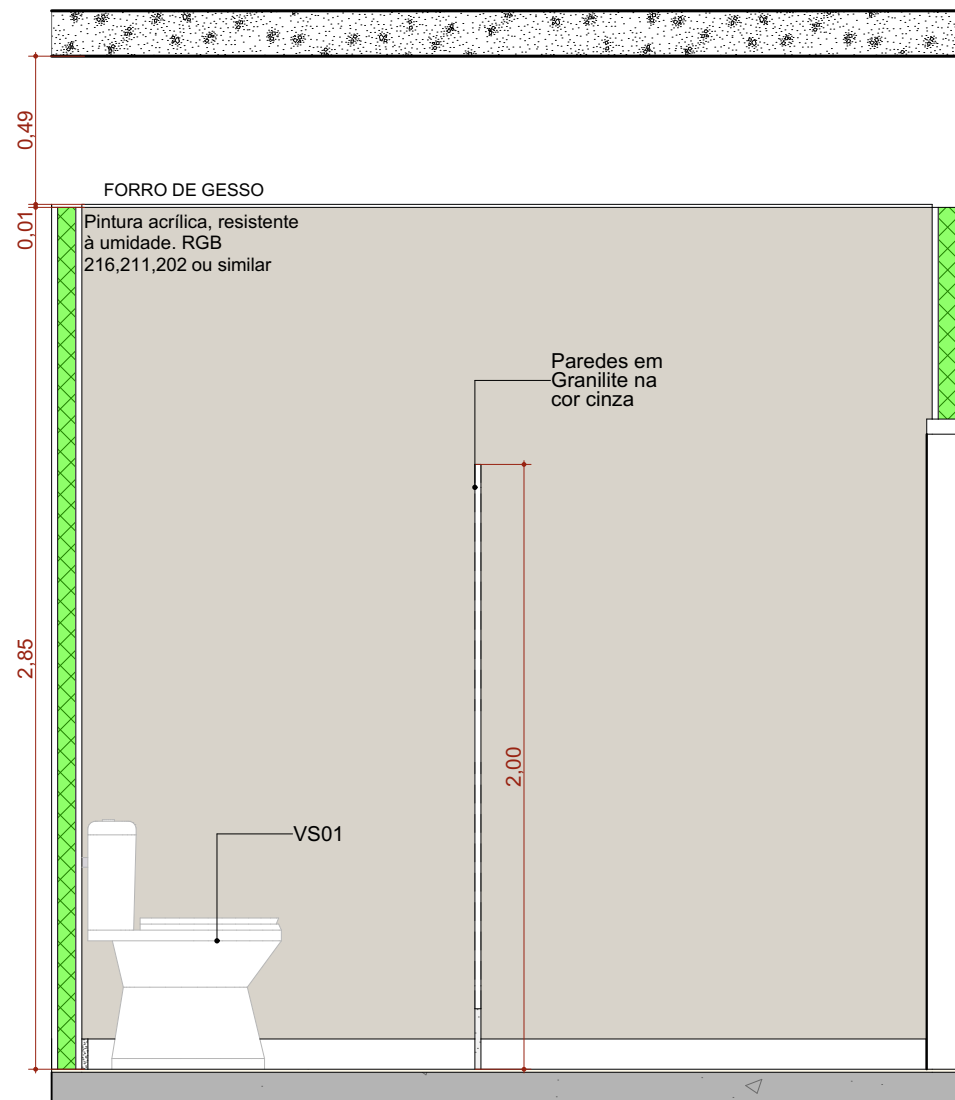
A.M.02 VISTA 02 Escala: 1:25
