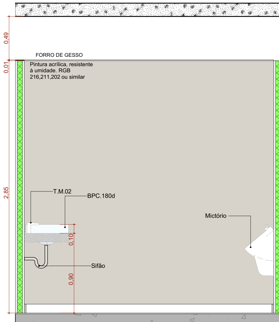
A.M.02 VISTA 01 Escala: 1:25
