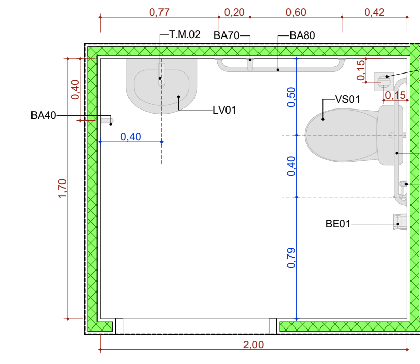
A.M.06 Sanitário PCD Masculino Escala: 1:25
