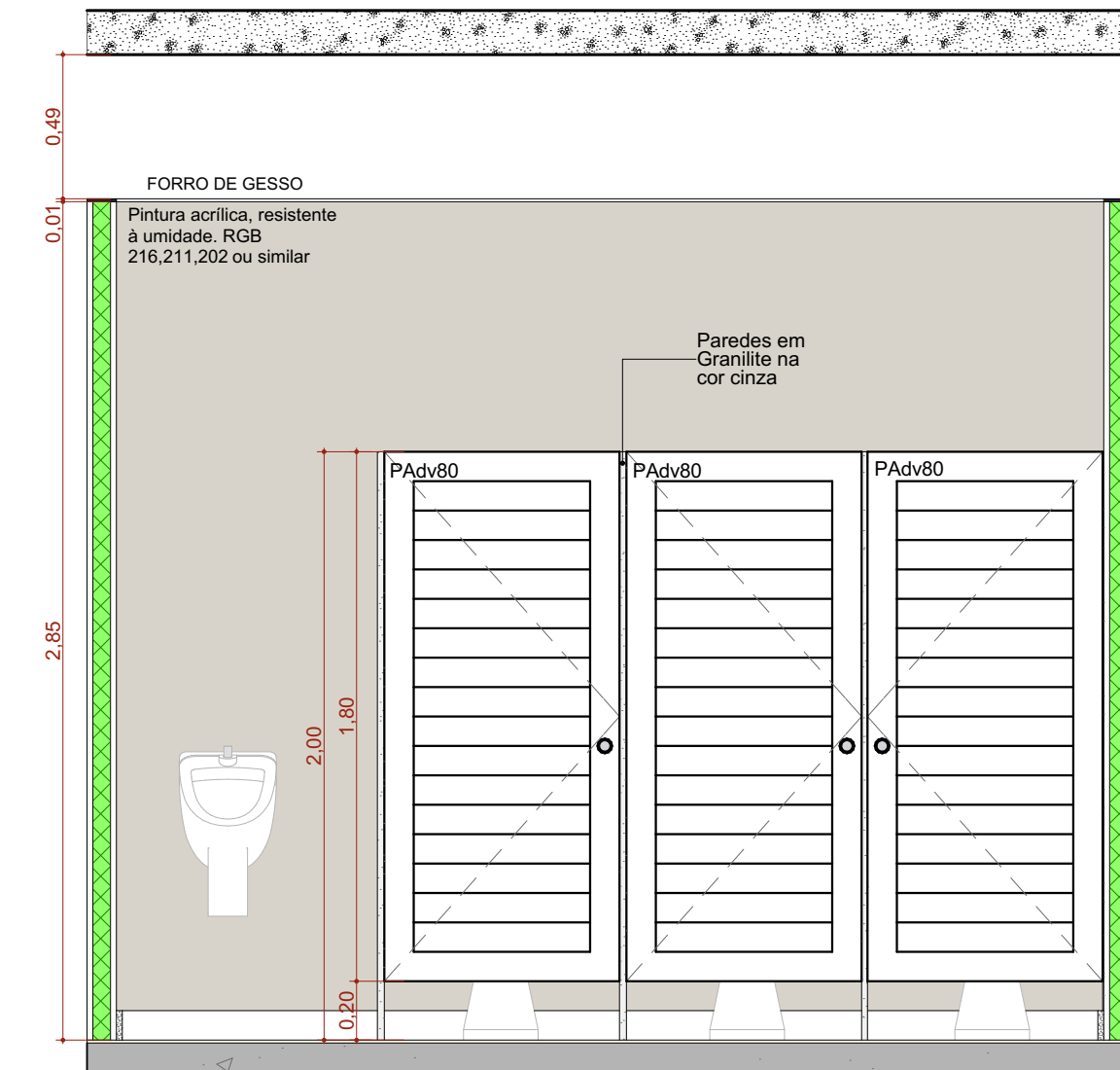
A.M.02 VISTA 04 Escala: 1:25
