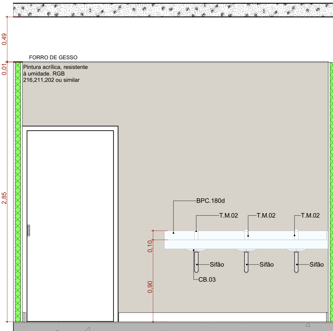
A.M.02 VISTA 03 Escala: 1:25
