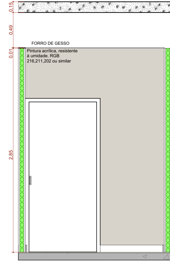
A.M.05 VISTA 04 Escala: 1:25
