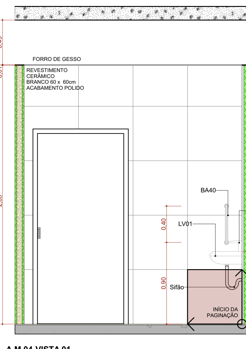
A.M.04 VISTA 01 Escala: 1:25
