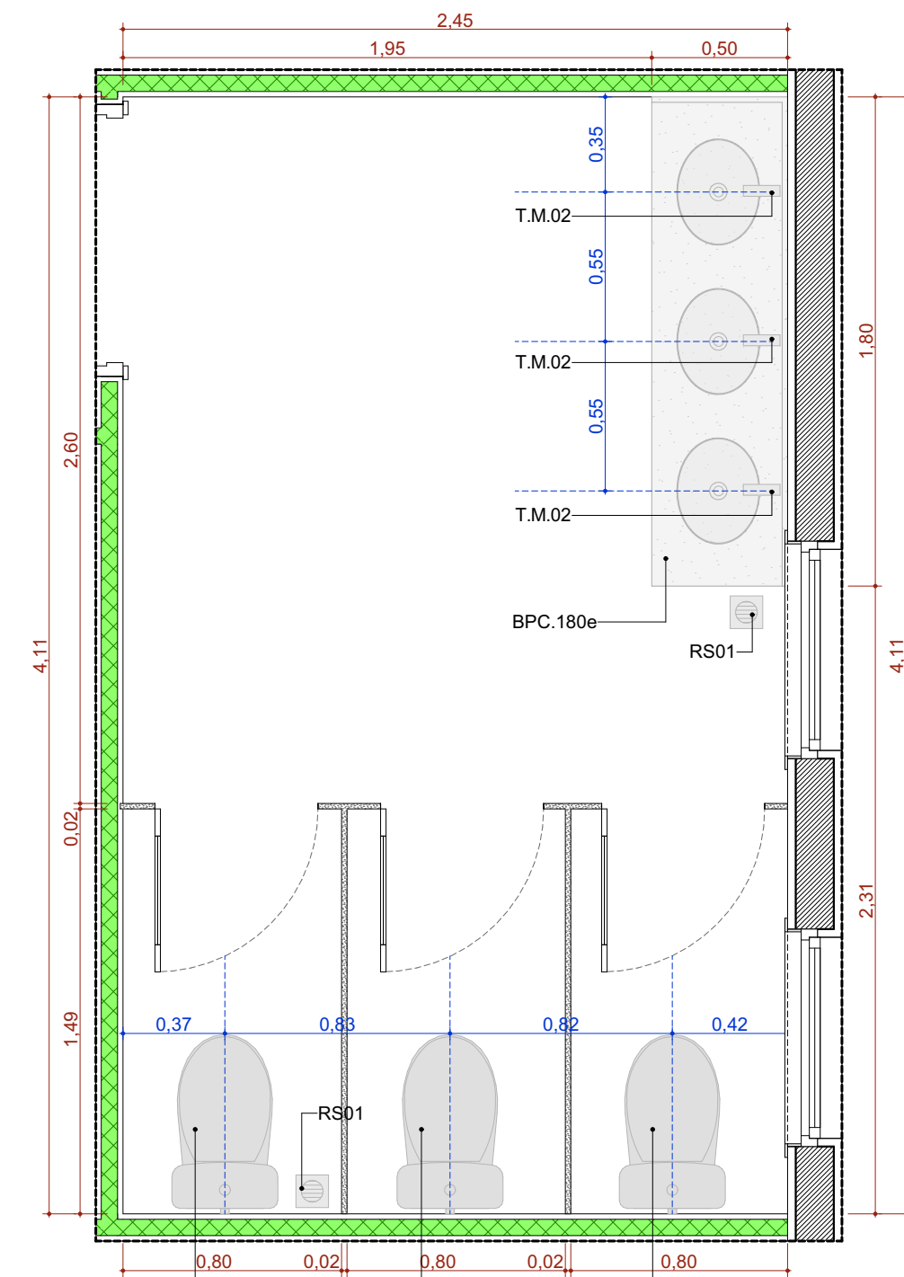
A.M.03 Sanitário Feminino Escala: 1:25
