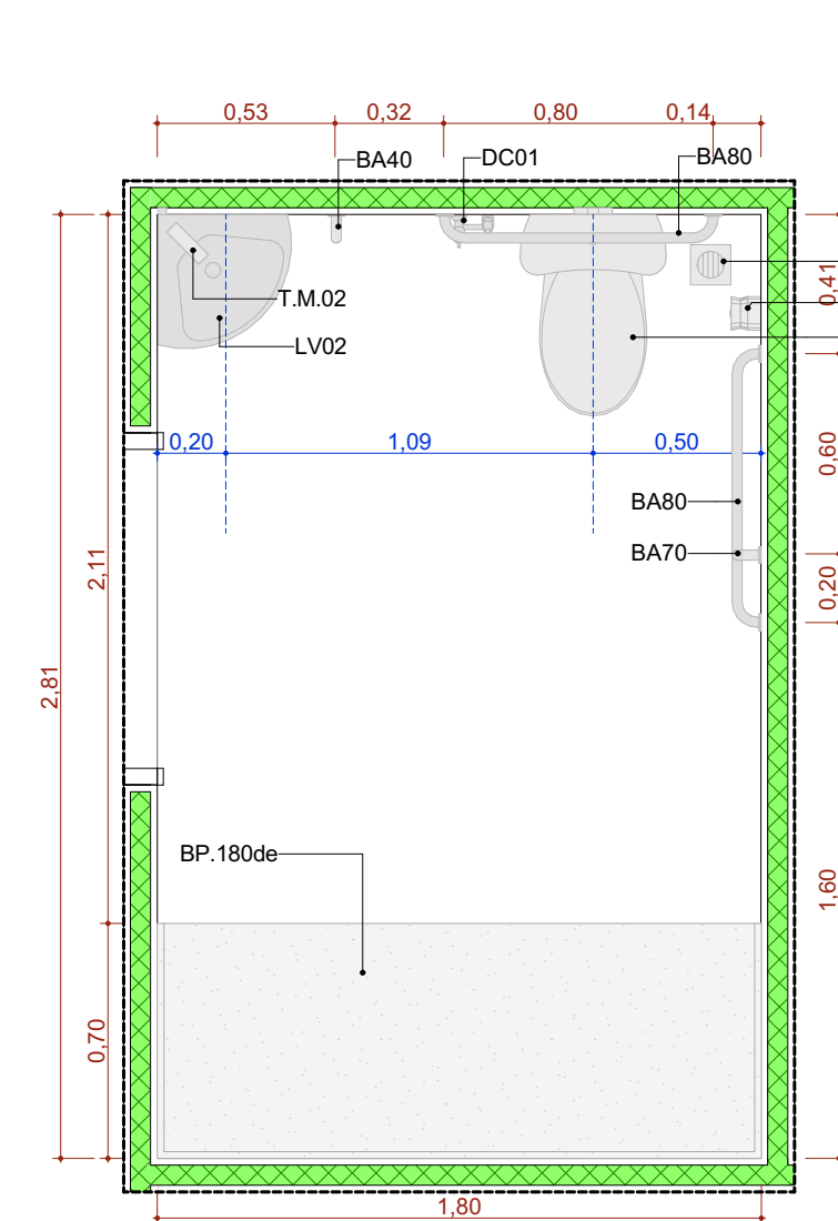
A.M.01 Sanitário Família Escala: 1:25
