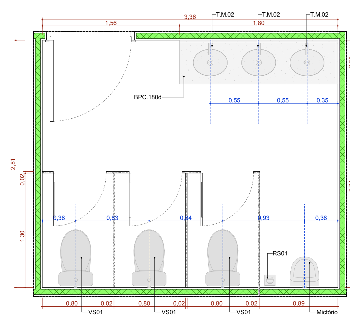
A.M.02 Sanitário Masculino Escala: 1:25
