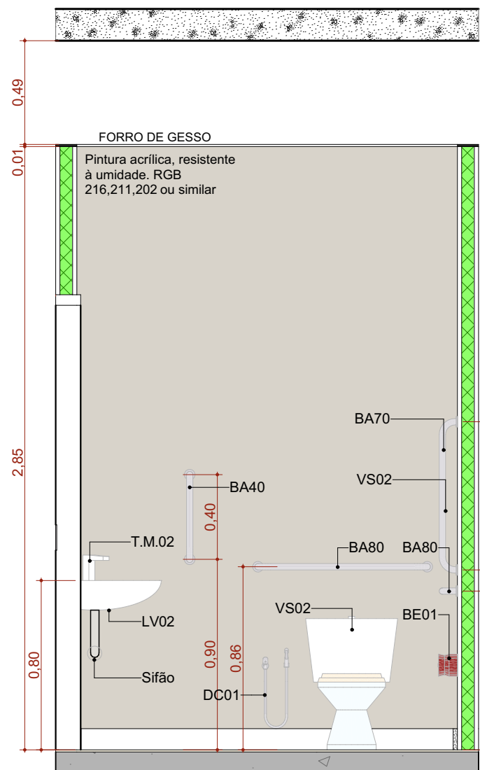
A.M.01 VISTA 01 Escala: 1:25
