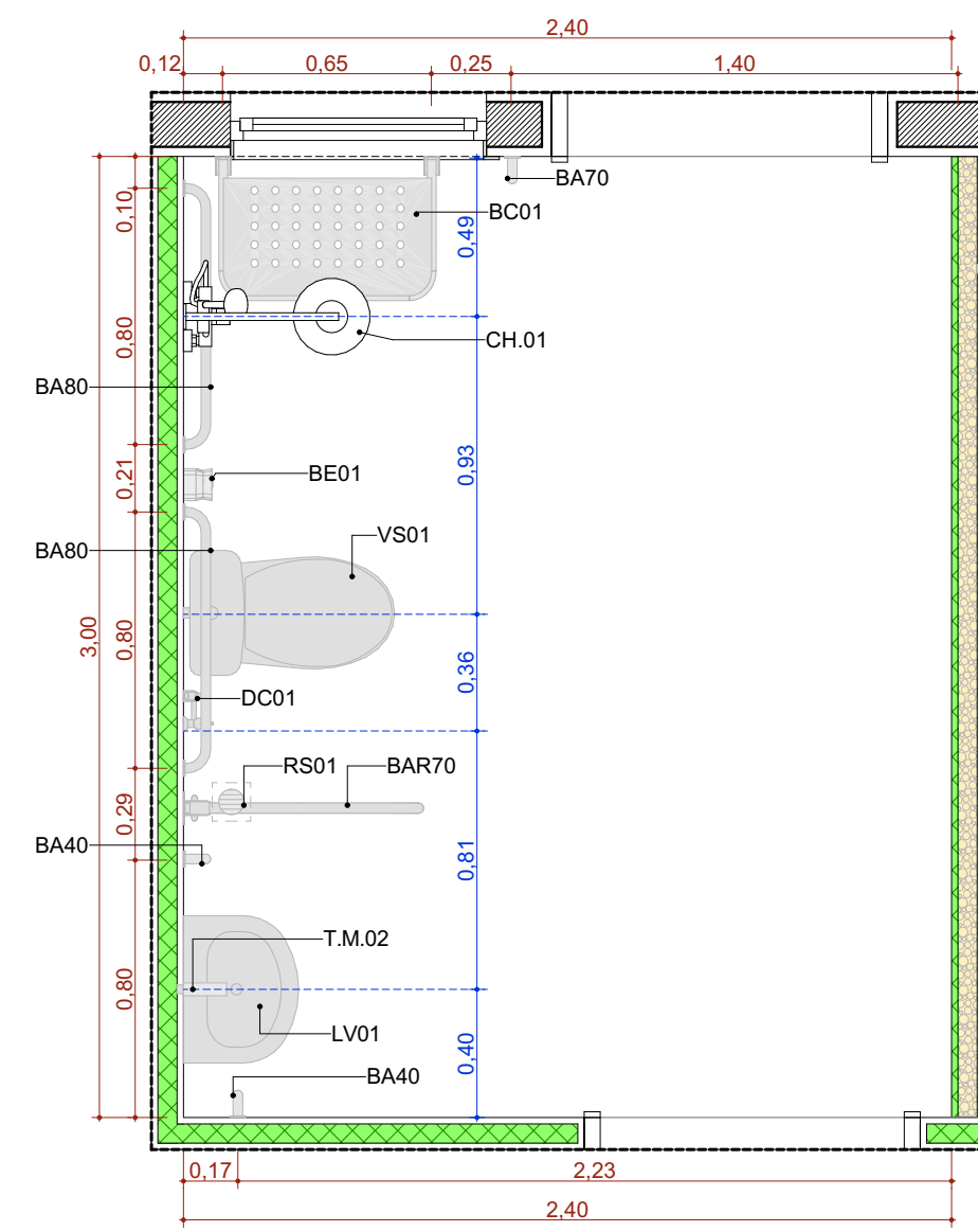
A.M.04 Banheiro PCD Práticas Escala: 1:25
