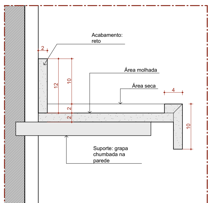
Det. B.P.b Bancada de Pedra Detalhe área molhada Escala 1:5
