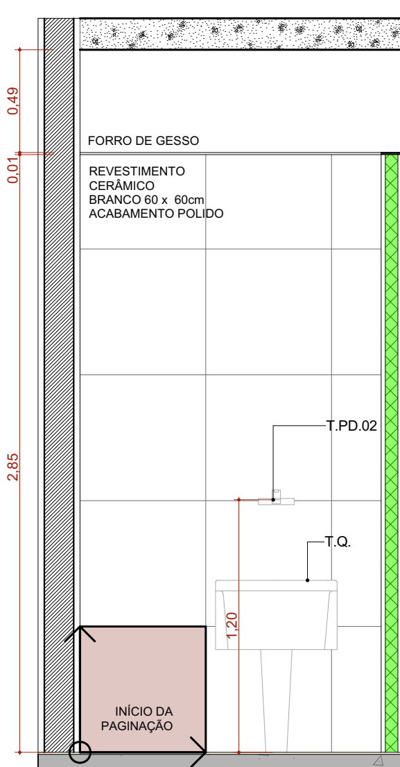
A.M.16 VISTA 02 Escala: 1:25
