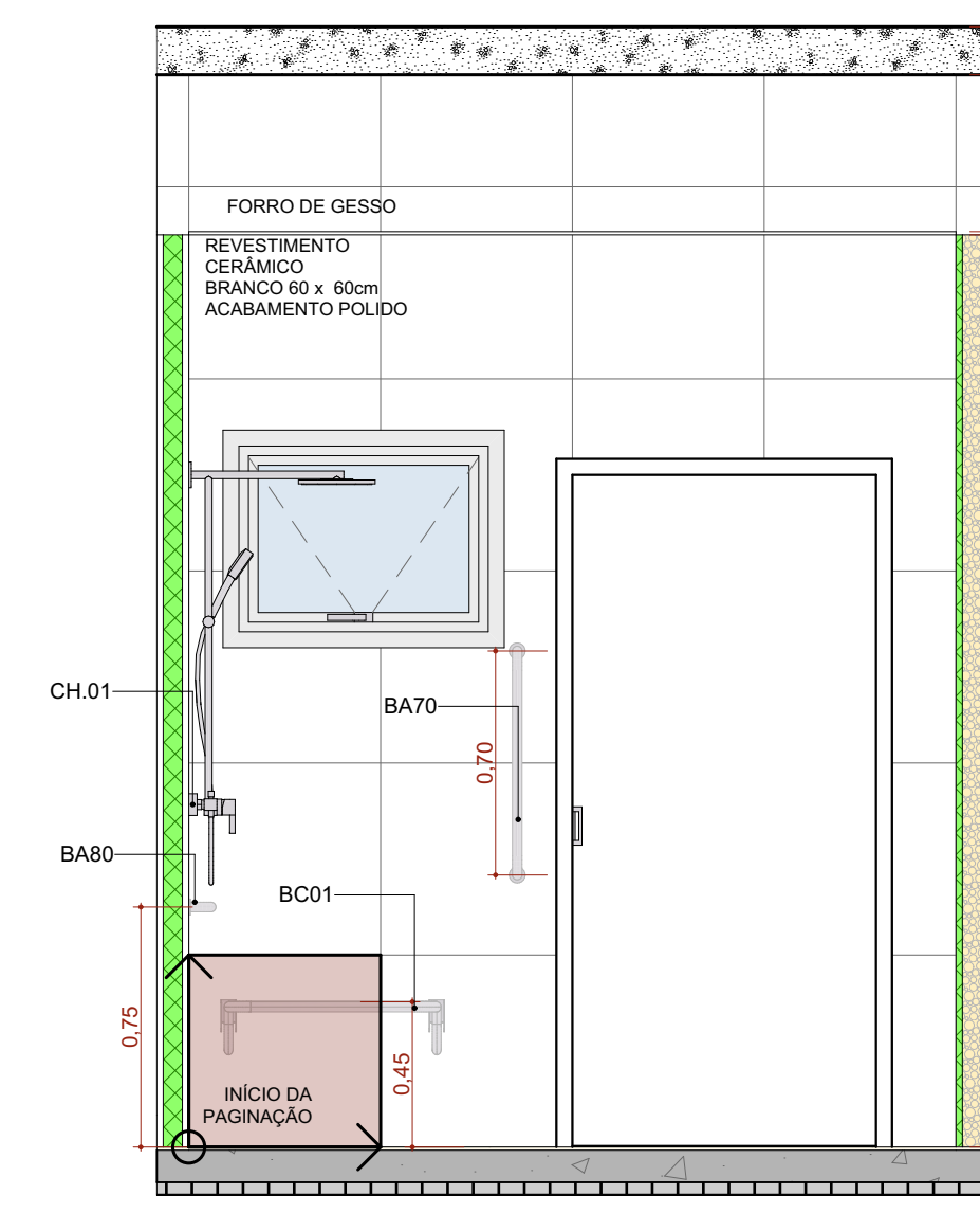
A.M.04 VISTA 03 Escala: 1:25
