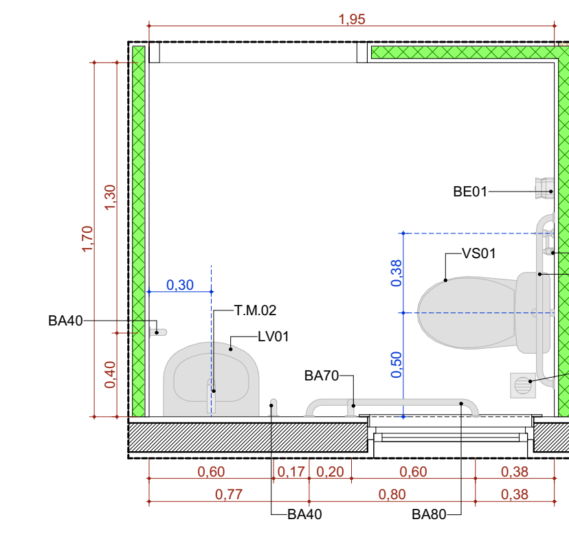
A.M.05 Sanitário PCD Gine.1 Escala: 1:25
