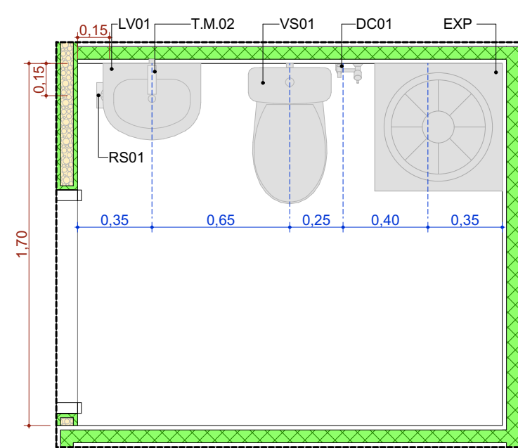
A.M.08 Sanitário Ostimizado
