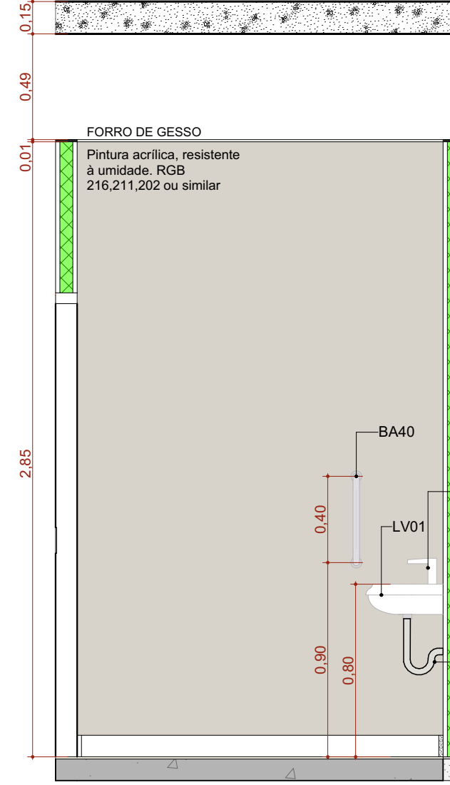
A.M.06 VISTA 01 Escala: 1:25
