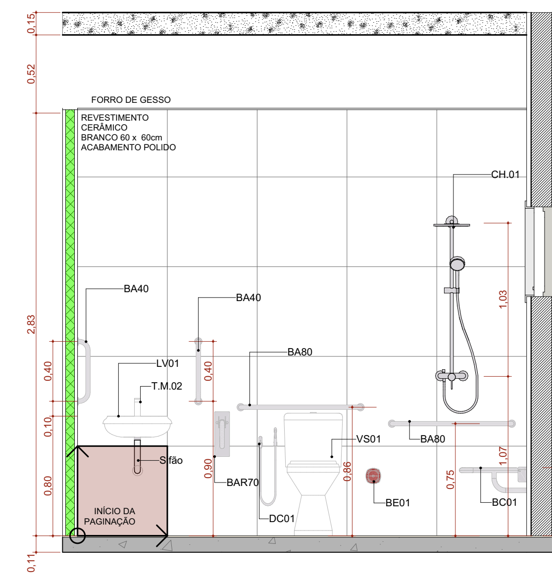
A.M.04 VISTA 04 Escala: 1:25
