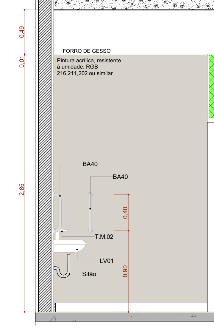
A.M.05 VISTA 02 Escala: 1:25
