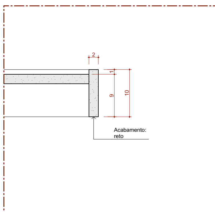
Det. B.P.d Bancada de Pedra Detalhe área molhada Escala 1:5
