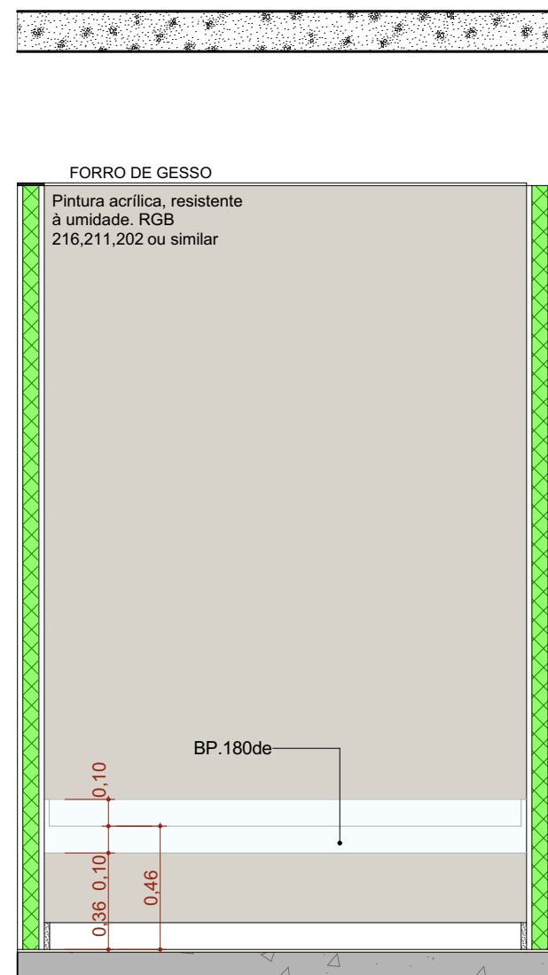
A.M.01 VISTA 02 Escala: 1:25
