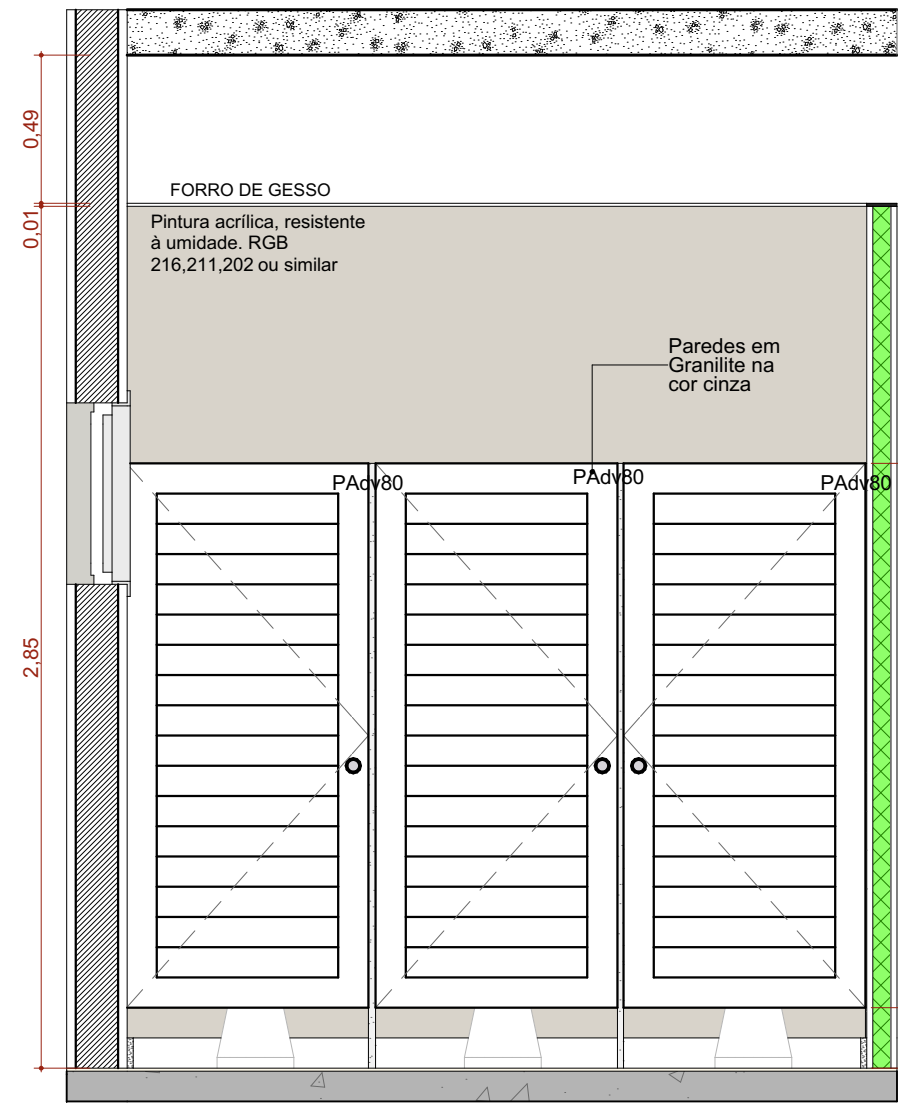
A.M.03 VISTA 01 Escala: 1:25
