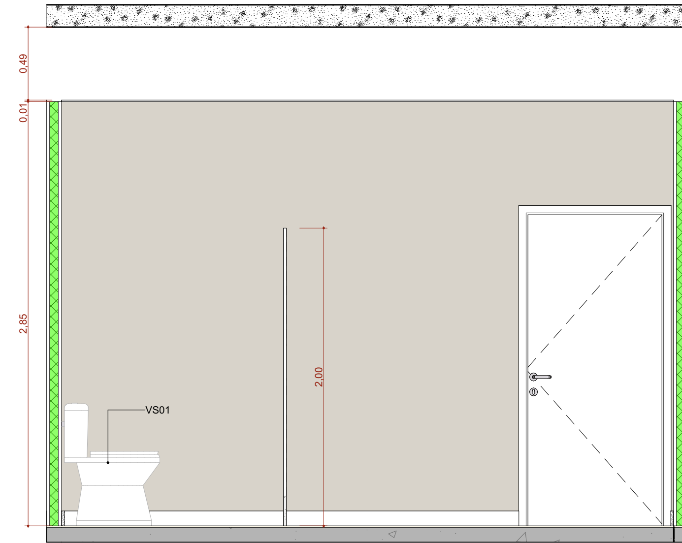
A.M.03 VISTA 04 Escala: 1:25
