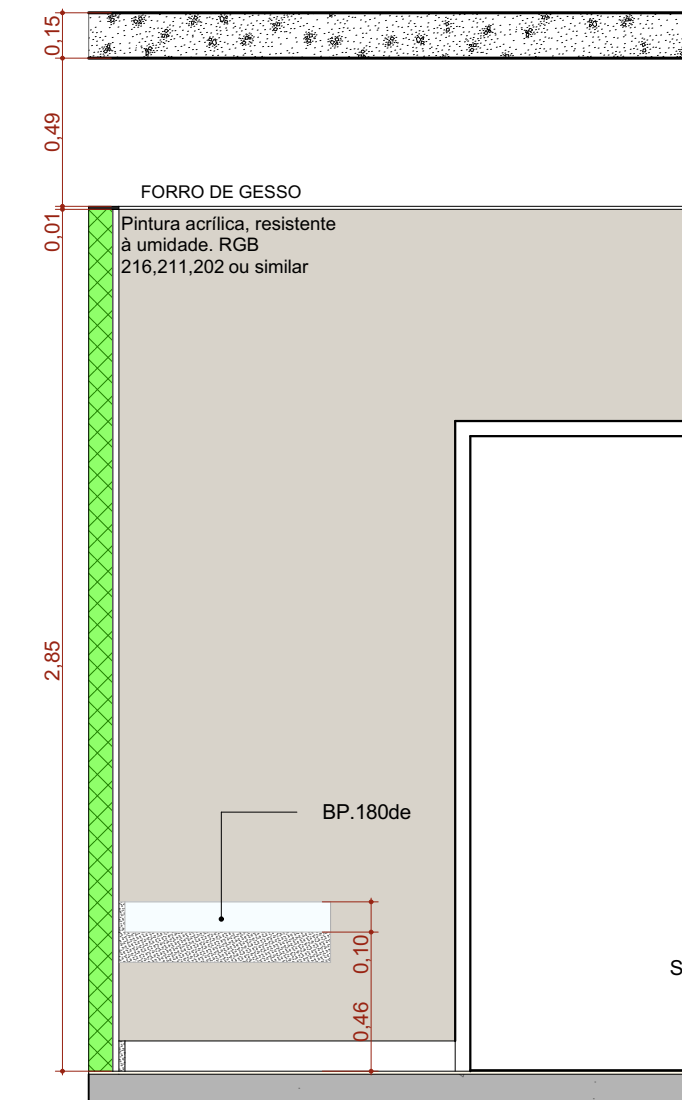
A.M.01 VISTA 03 Escala: 1:25
