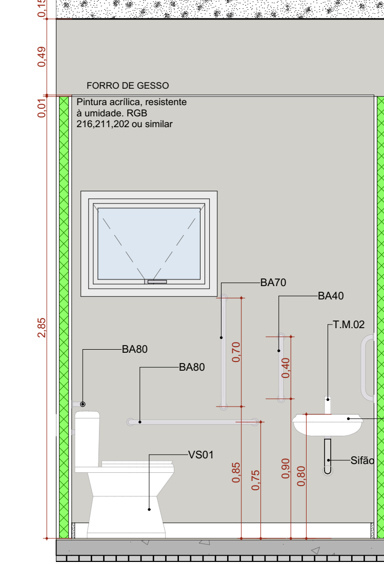
A.M.05 VISTA 01 Escala: 1:25
