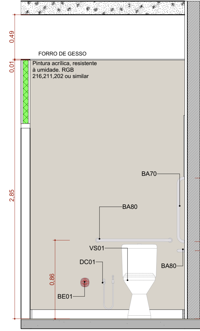
A.M.05 VISTA 03 Escala: 1:25
