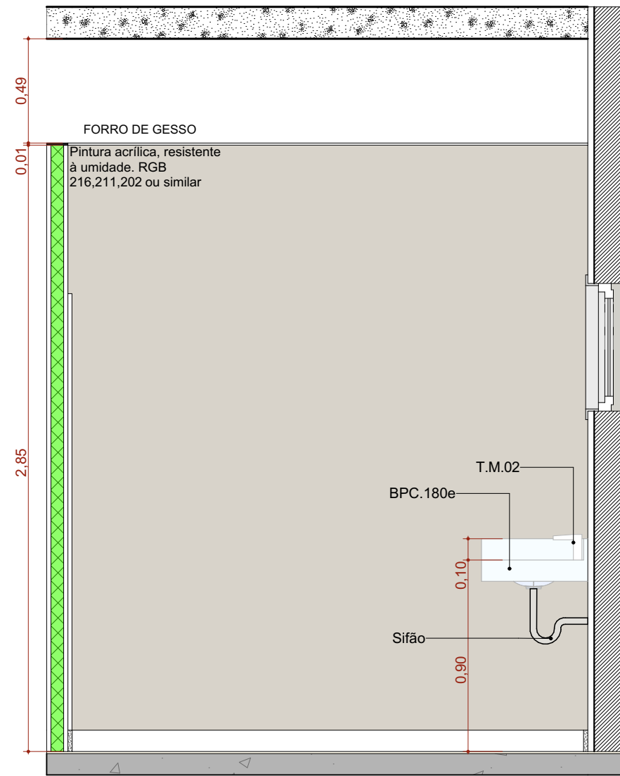
A.M.03 VISTA 03 Escala: 1:25
