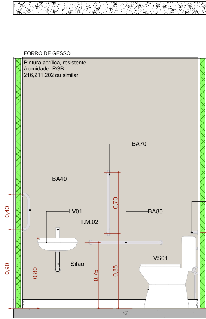
A.M.06 VISTA 02 Escala: 1:25
