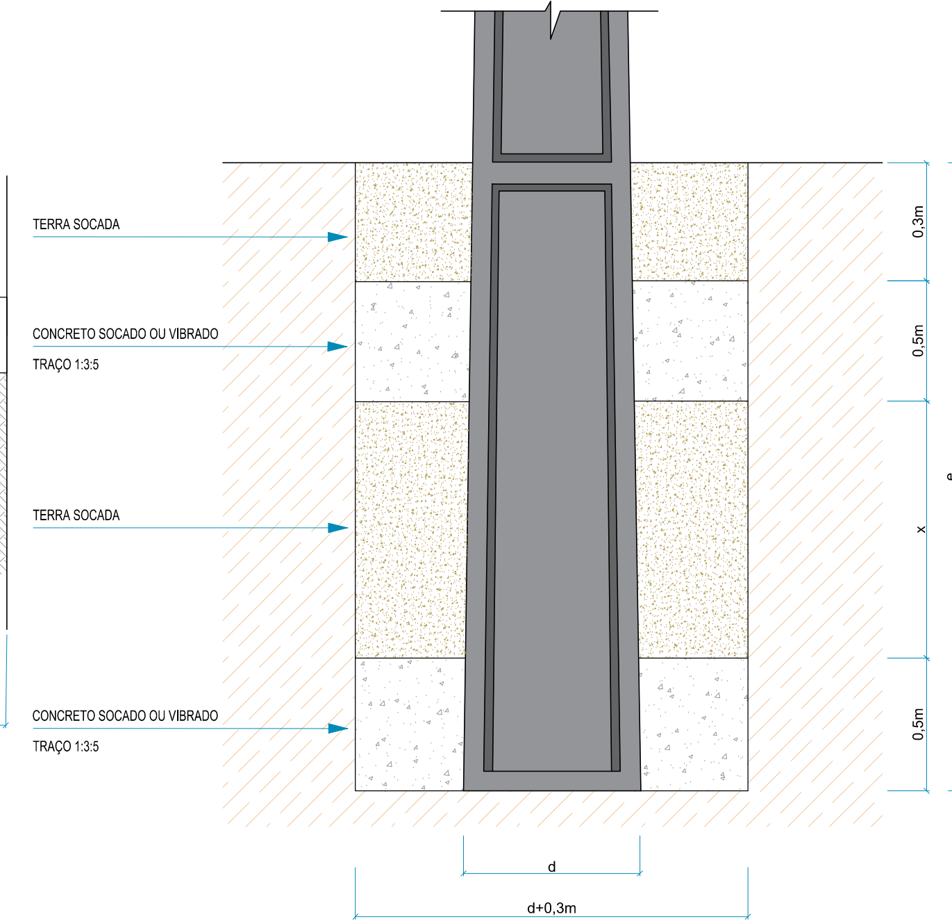
DETALHE ENGASTAMENTO esc 1:20
