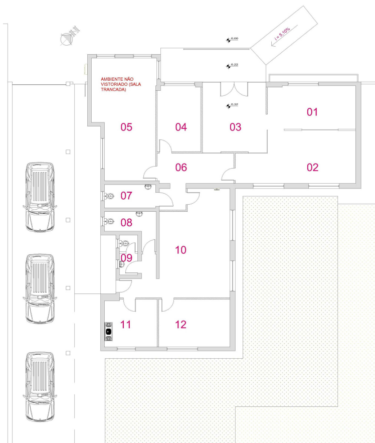
Imagem 01: Planta baixa do imóvel
