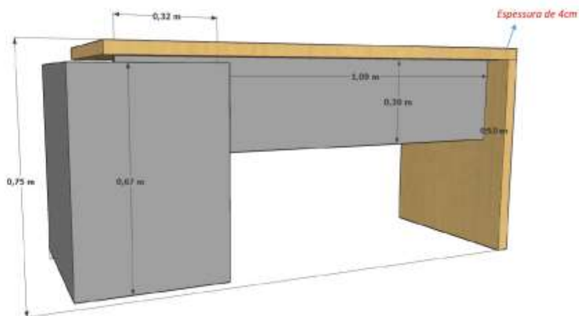
PERSPECTIVA EXTERNA
