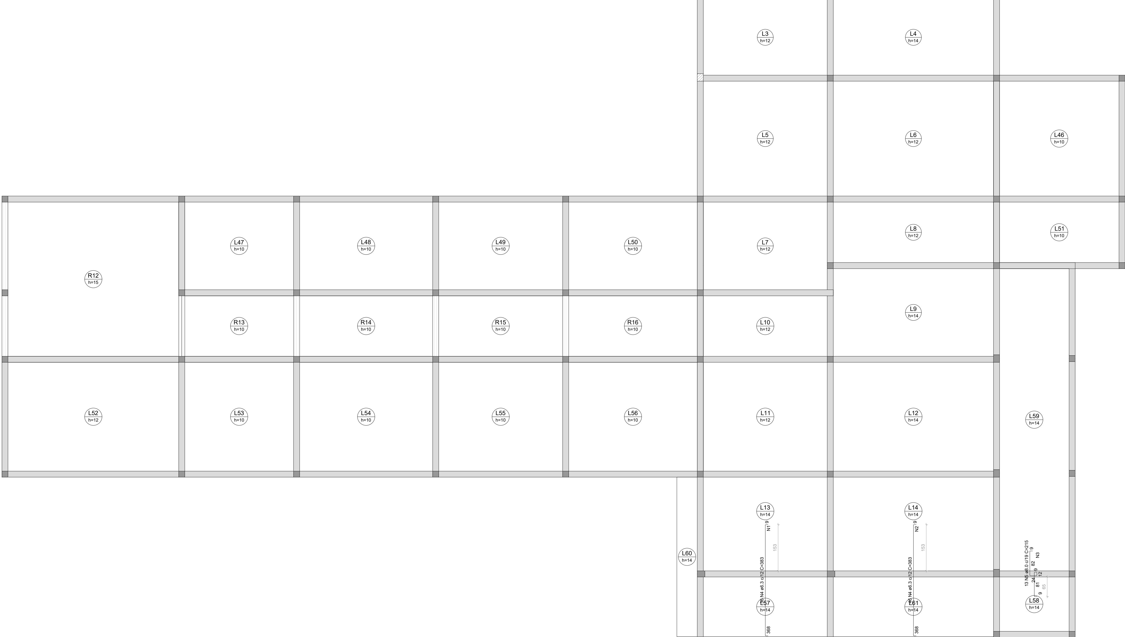
Armação Negativa das Lajes do Pav. Cobertura (Eixo Y) escala 1:50
