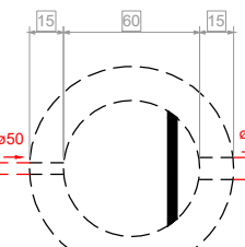
Caixa de gordura - TÉRREO Planta baixa - ESC. 1:25
