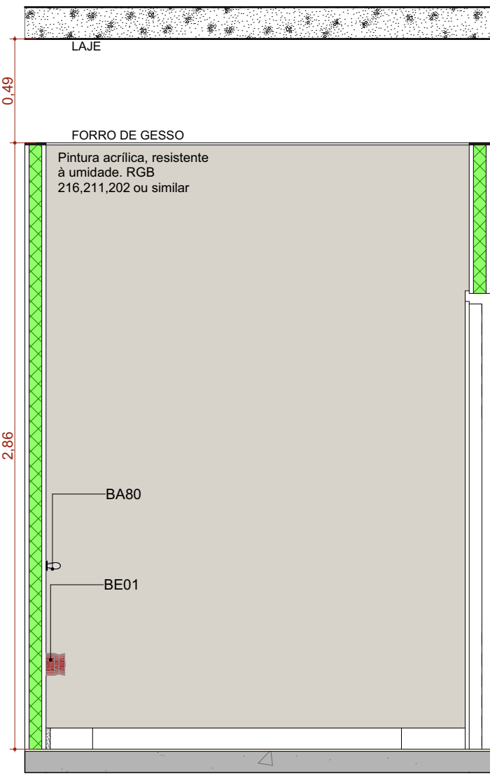
A.M.11 VISTA 01 Escala: 1:25
