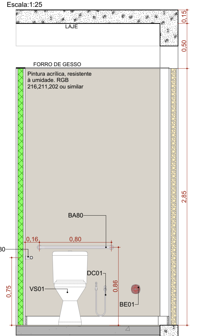
A.M.11 VISTA 04 Escala: 1:25
