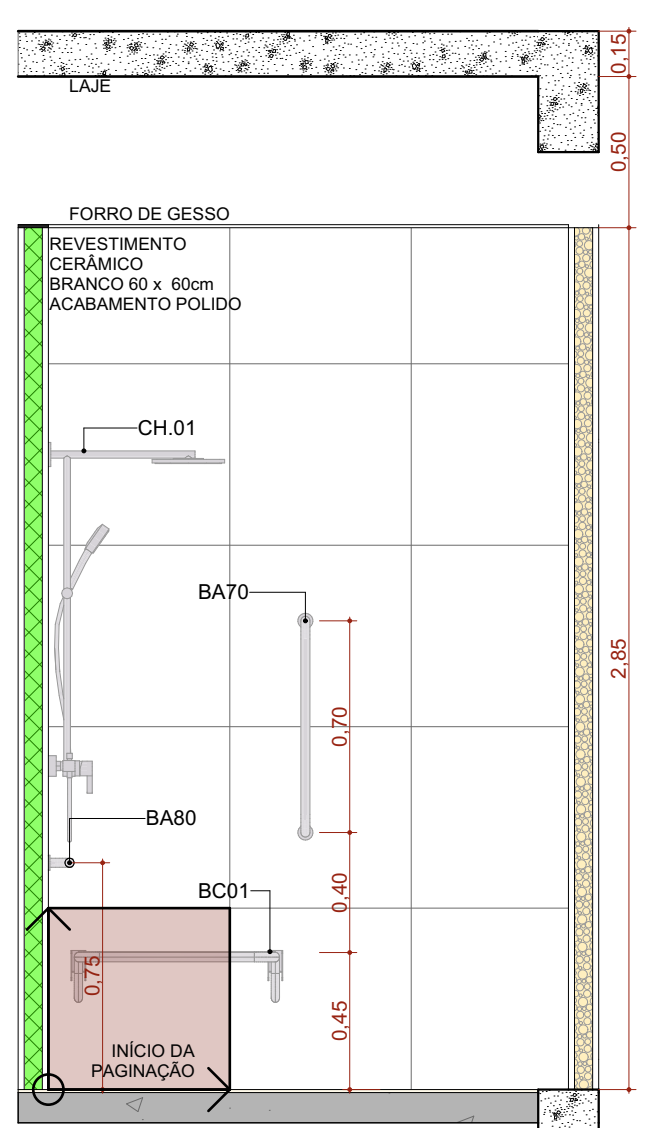
A.M.08 VISTA 02 Escala: 1:25
