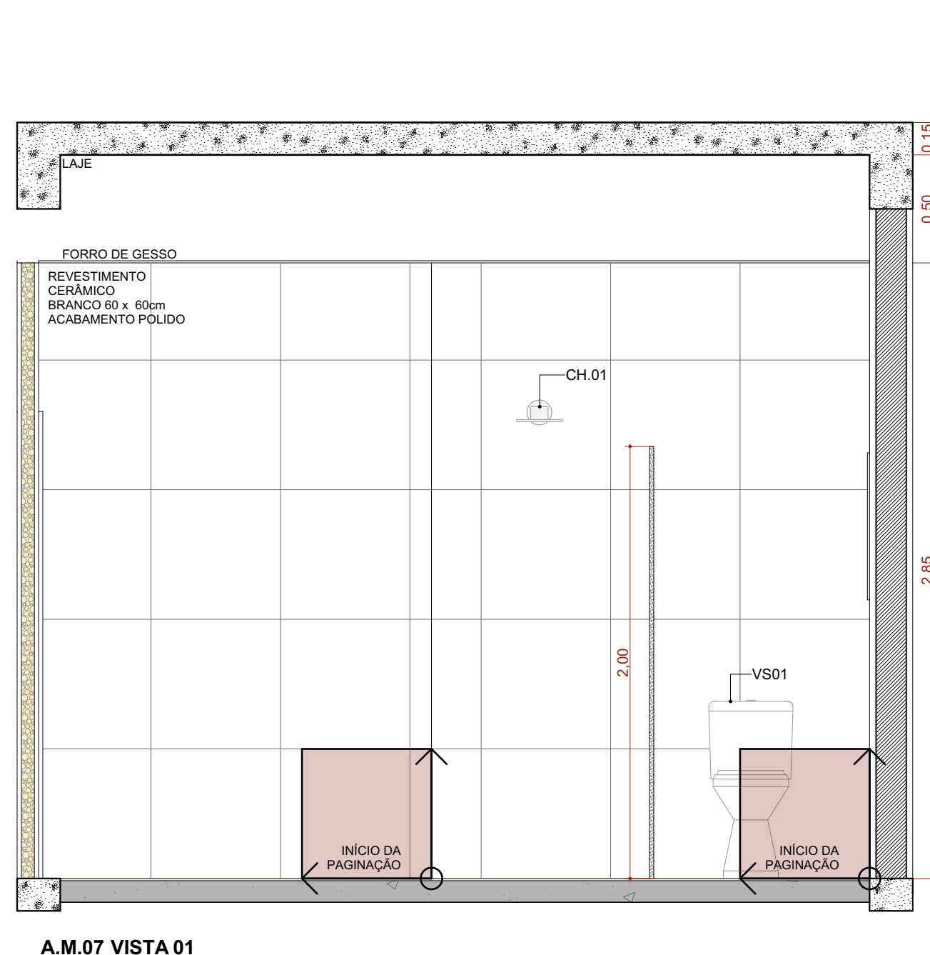
A.M.07 VISTA 01 Escala: 1:25
