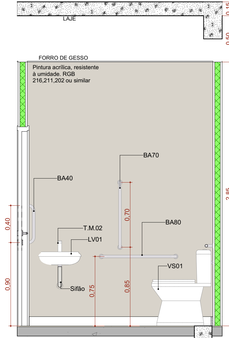
A.M.11 VISTA 02 Escala: 1:25
