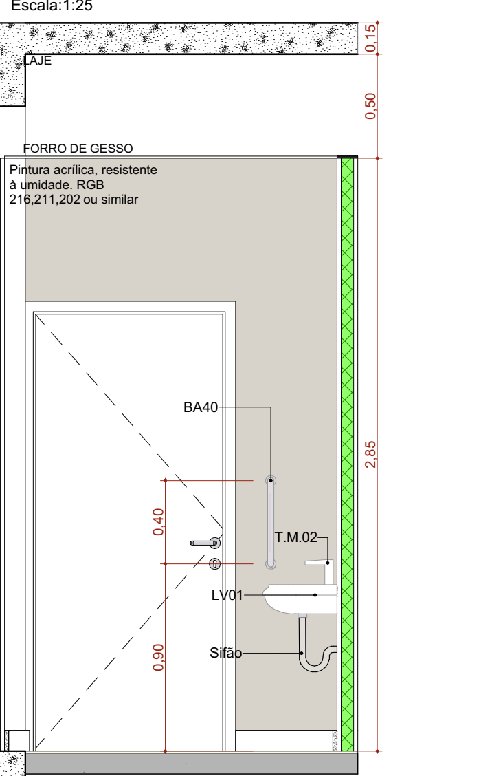
A.M.11 VISTA 03 Escala: 1:25
