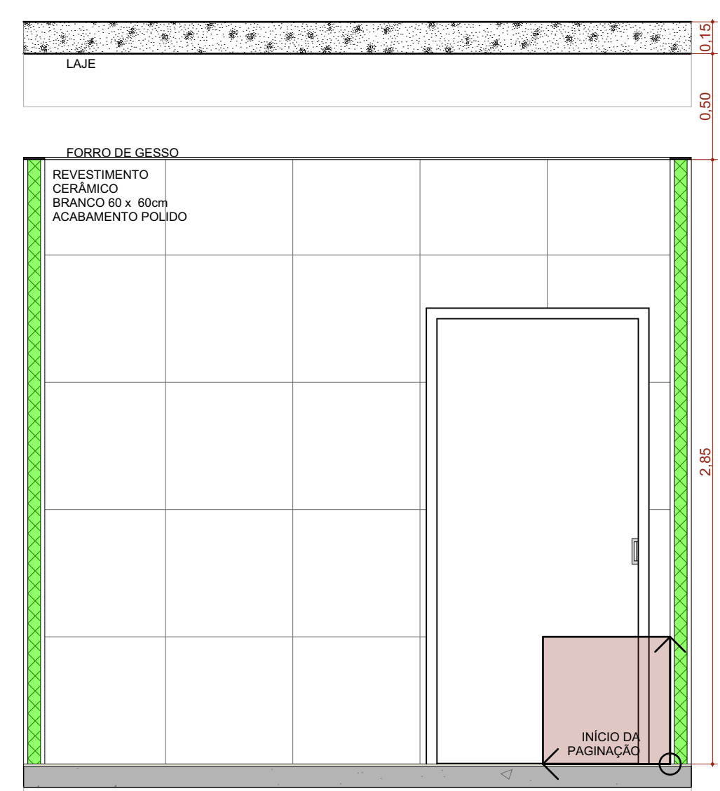
A.M.08 VISTA 04 Escala: 1:25
