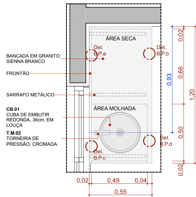
BPC.120d Escala: 1:20
