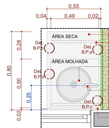
BPC.80d Escala: 1:20
