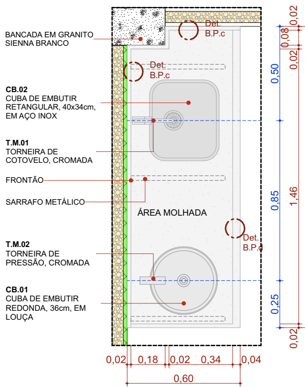
BPC.160d Escala: 1:20
