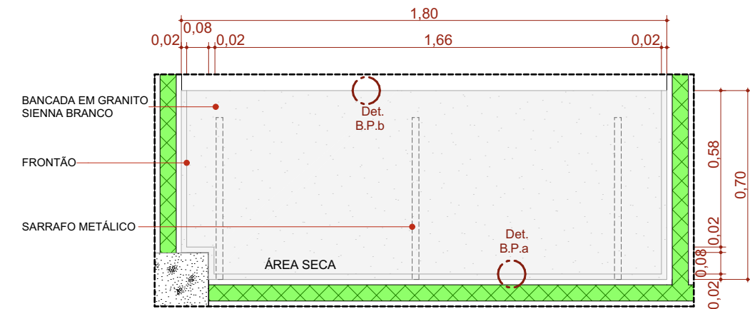
BP.180de Escala: 1:20
