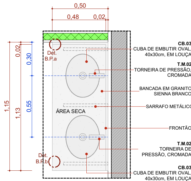
BPC.115e Escala: 1:20
