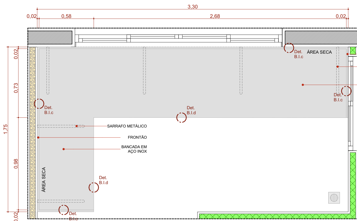
BI.330de Escala: 1:20
