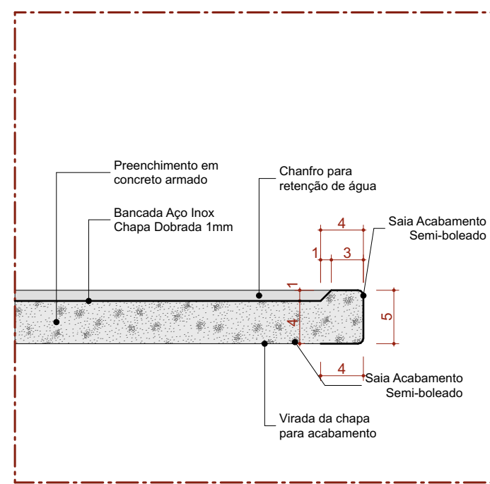
Det. B.I.b Bancada de Inox Detalhe Saia - Área Molhada Escala: 1:5
