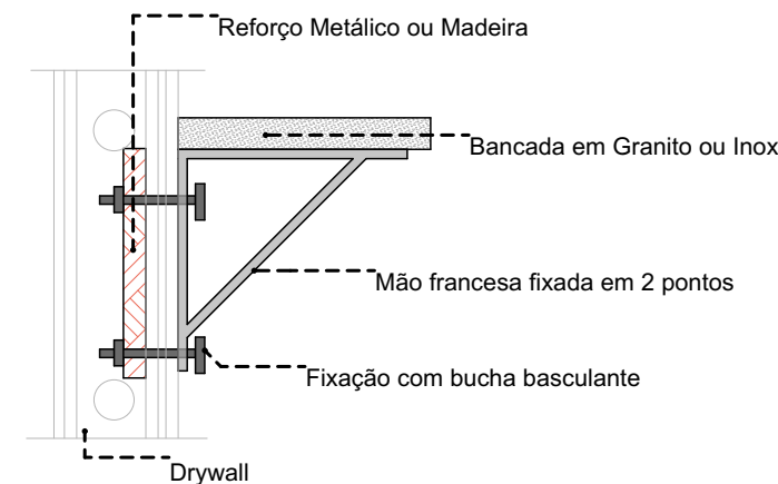
DETALHE 01: REFORÇO EM DRYWALL Escala: 1:20
