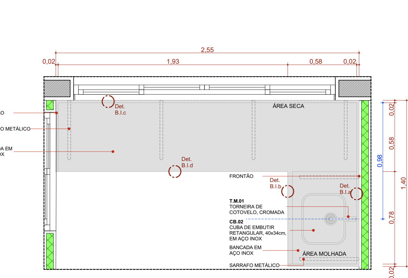
BI.255de Escala: 1:20
