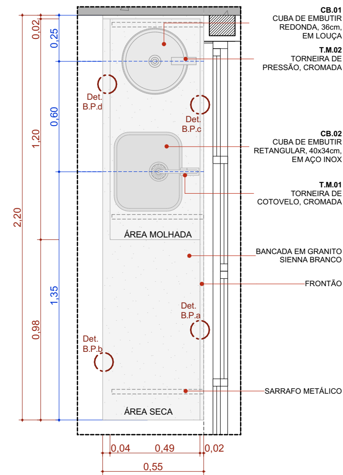
BPC.220e Escala: 1:20
