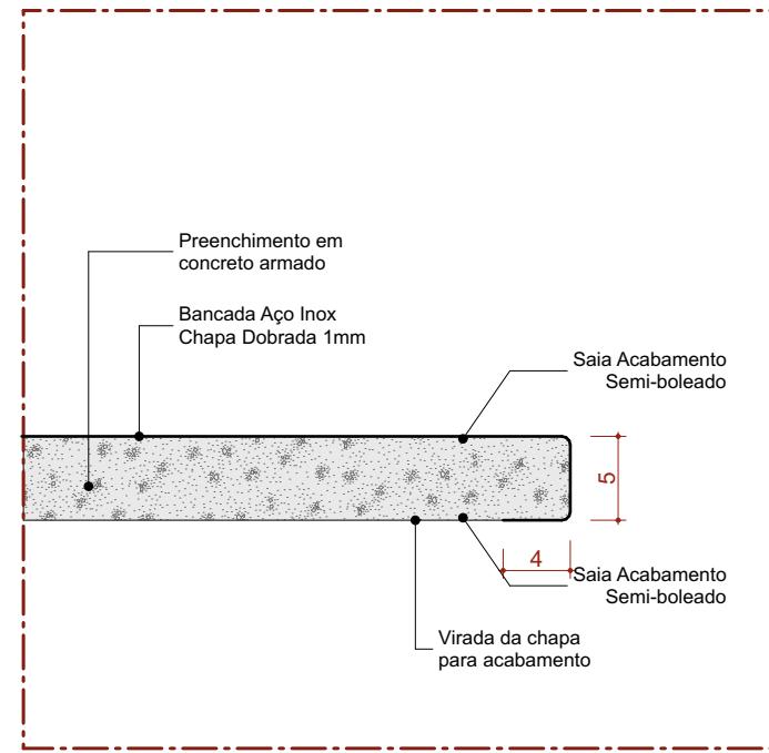
Det. B.I.d Bancada de Inox Detalhe Saia - Área seca Escala: 1:5
