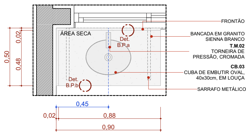
BPC.90e-Escovodromo Escala: 1:20
