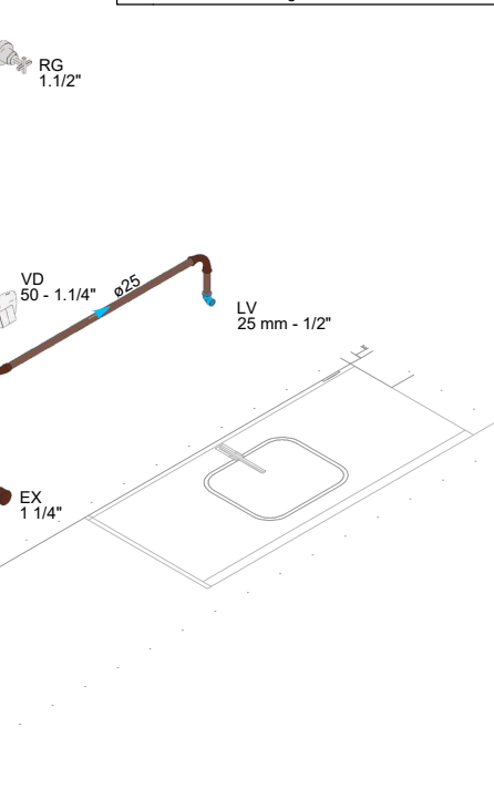
DETALHE HID-8 1:25
