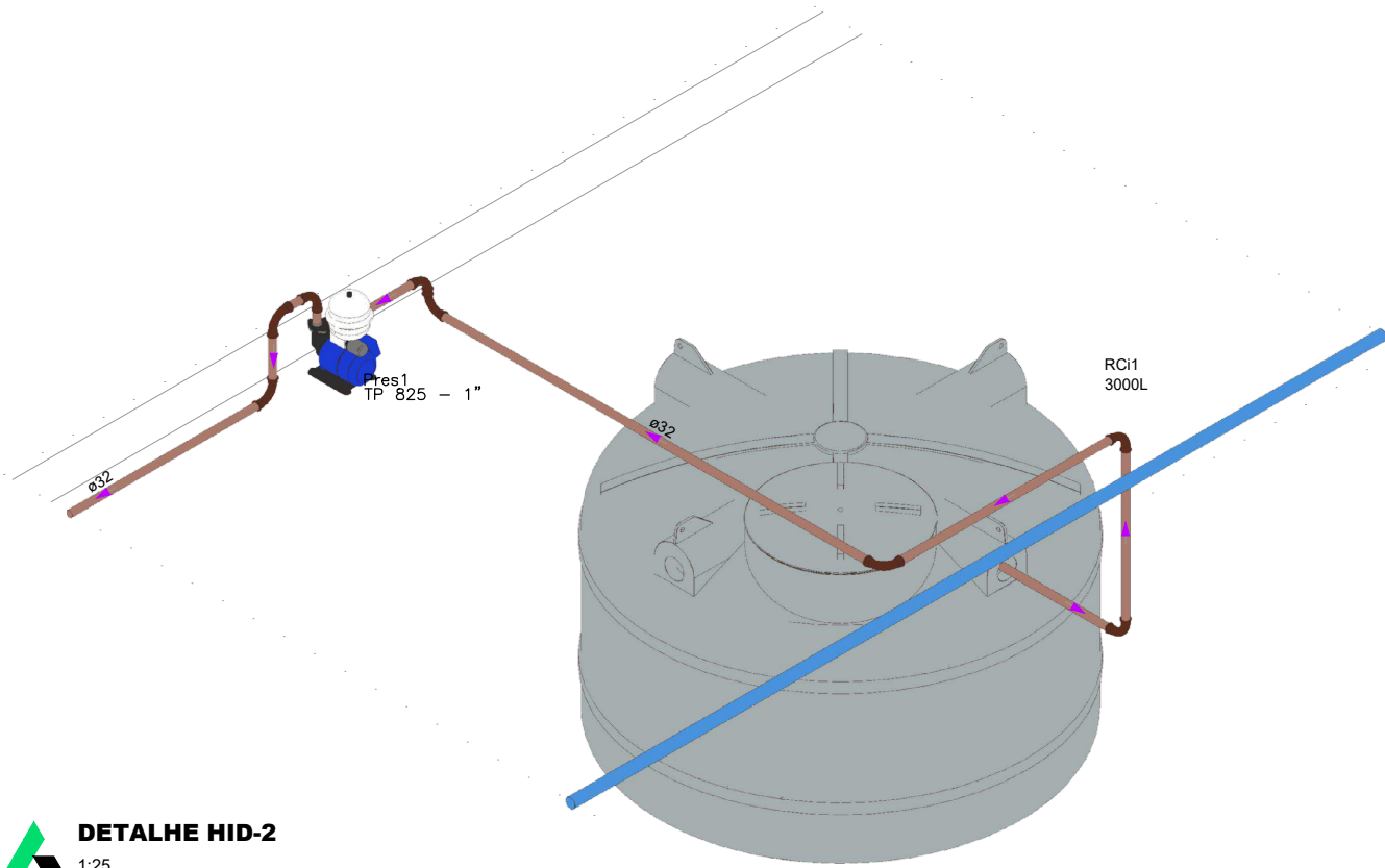
DETALHE HID-2 1:25
