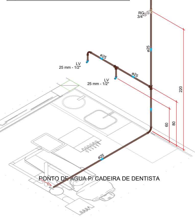
DETALHE HID-13 1:25
