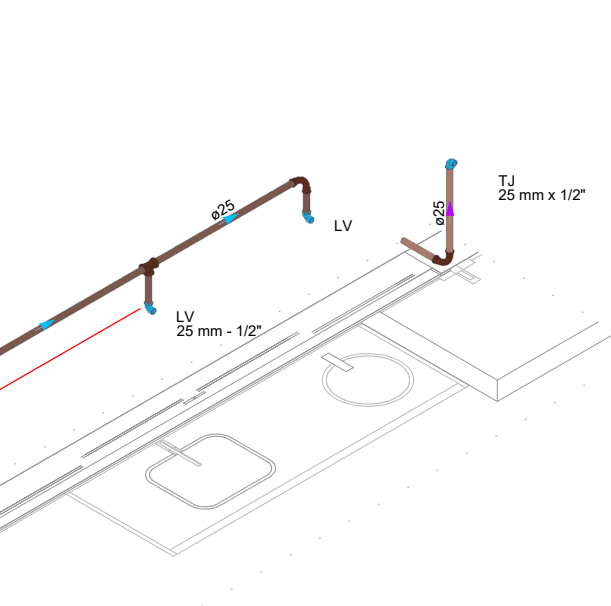
DETALHE HID-11 1:25
