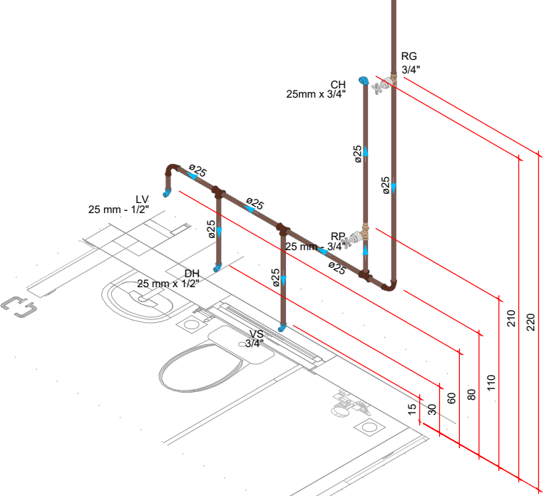
DETALHE HID-5 1:25
