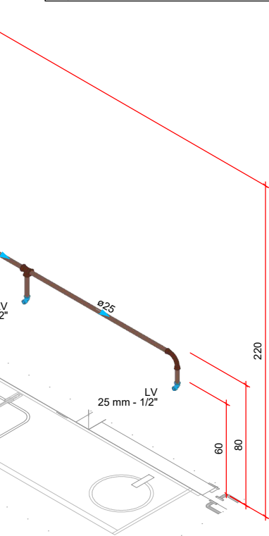
DETALHE HID-10 1:25
