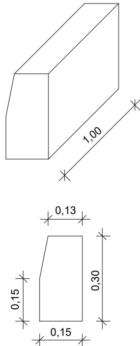
DETALHE MEIO-FIO
