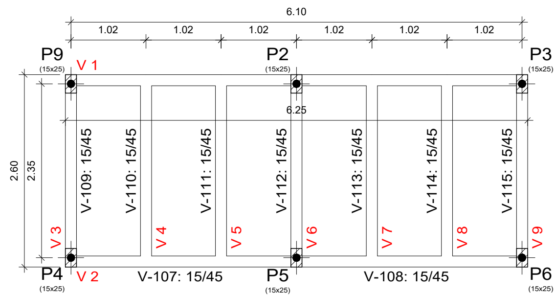
2 Planta de Formas Esc.1/50
