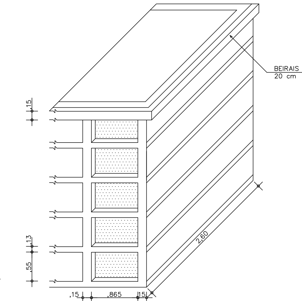
5 Detalhe gavetas S/ Escala
