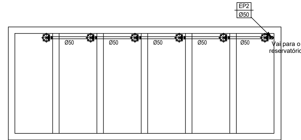
9 Projeto Sanitário Esc.1/50
