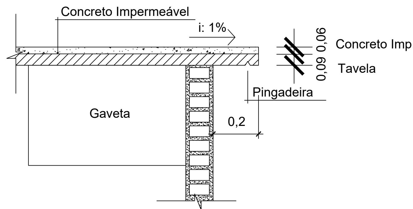
7 Detalhe Pingadeira S/ Escala
