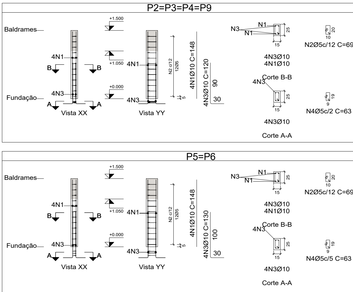
6 Detalhamento Pilaretes Esc.1/50
