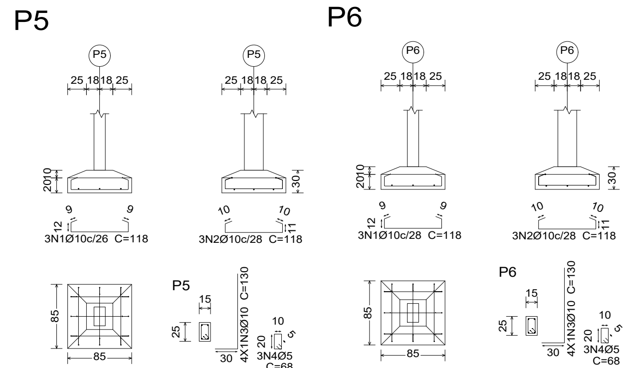
8 Detalhe Sapatas Esc.1/50
