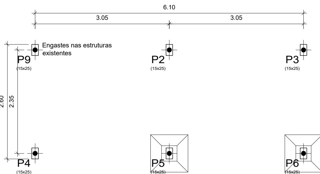
3 Locação Fundações Esc.1/50
