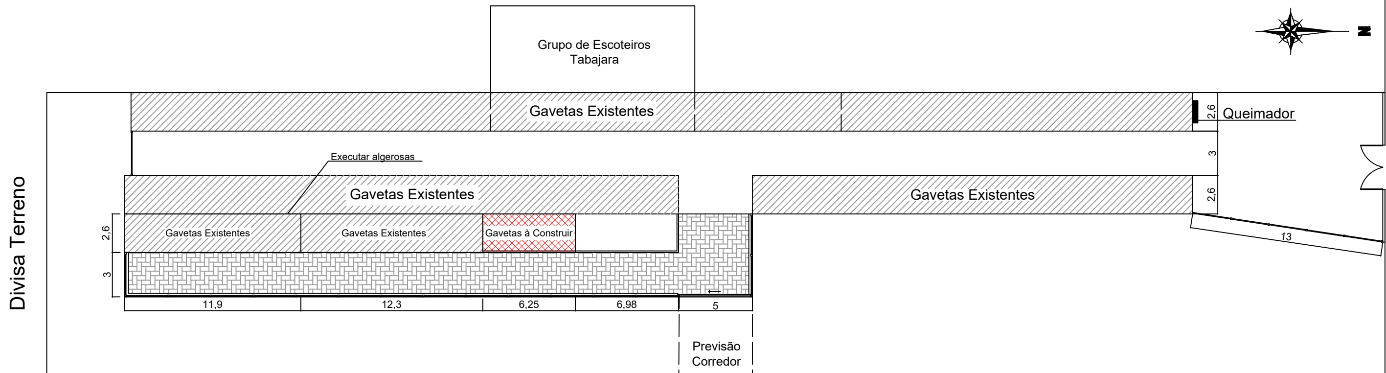
1 Planta Baixa Esc.1/250
