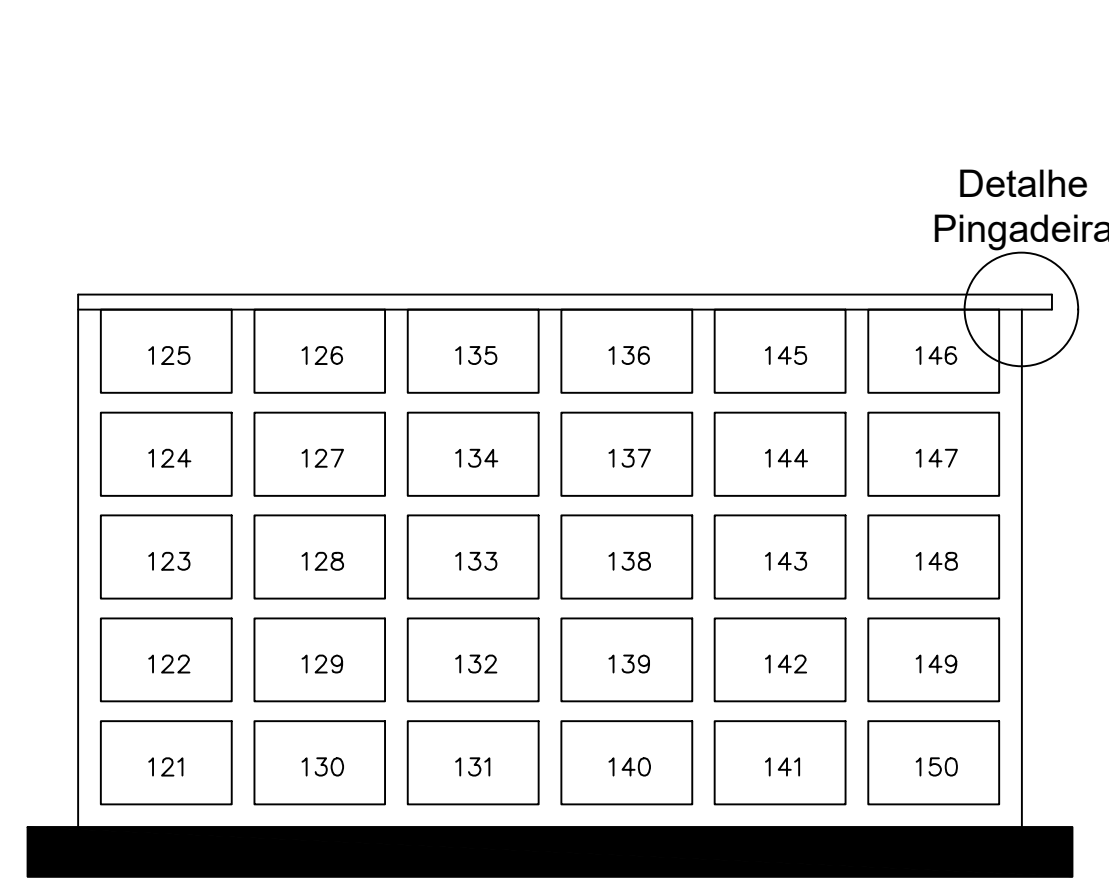
5 Detalhe gavetas S/ Escala
