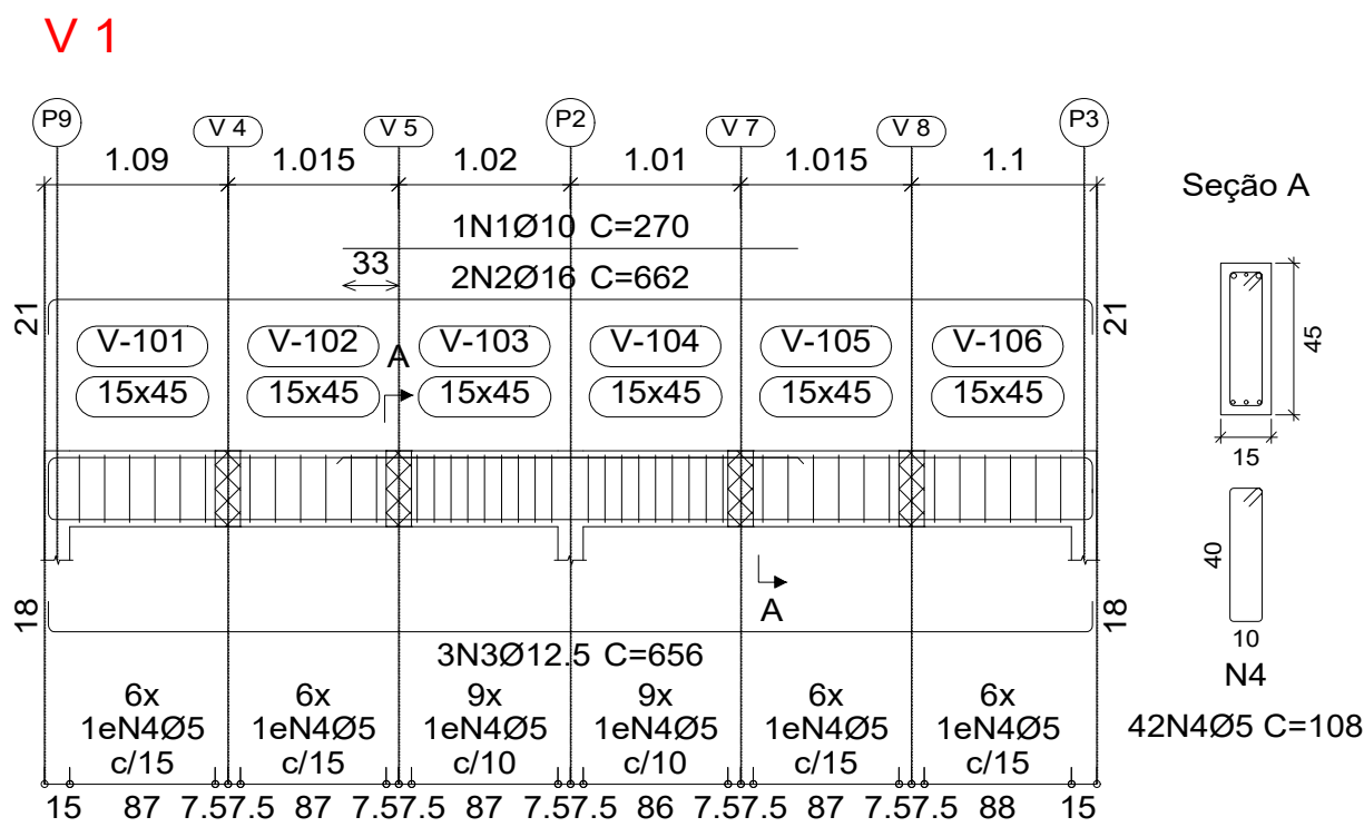
4 Detalhamento Vigas Esc.1/50 Corte 1/25
