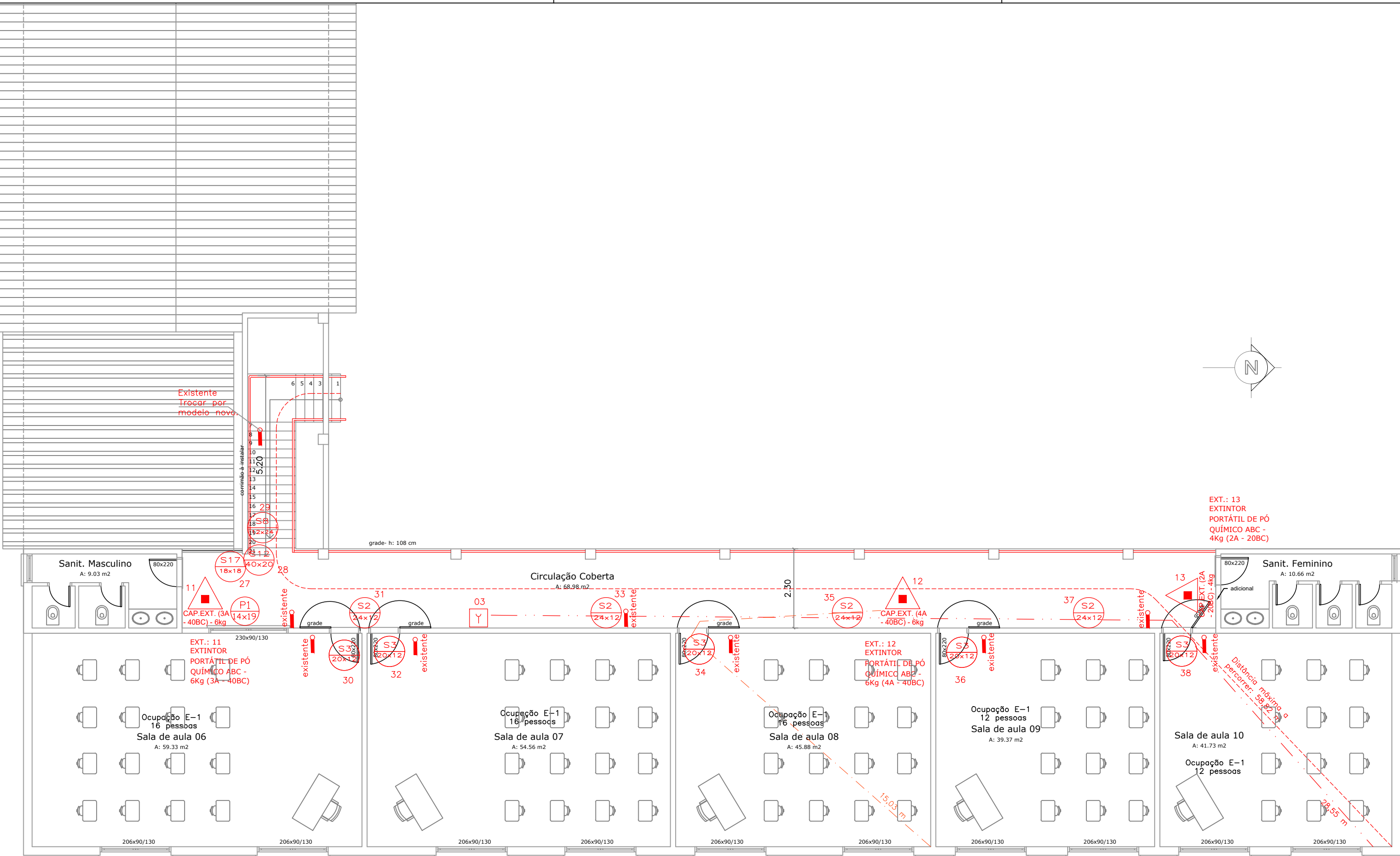
PLANTA DE BAIXA - SUPERIOR
