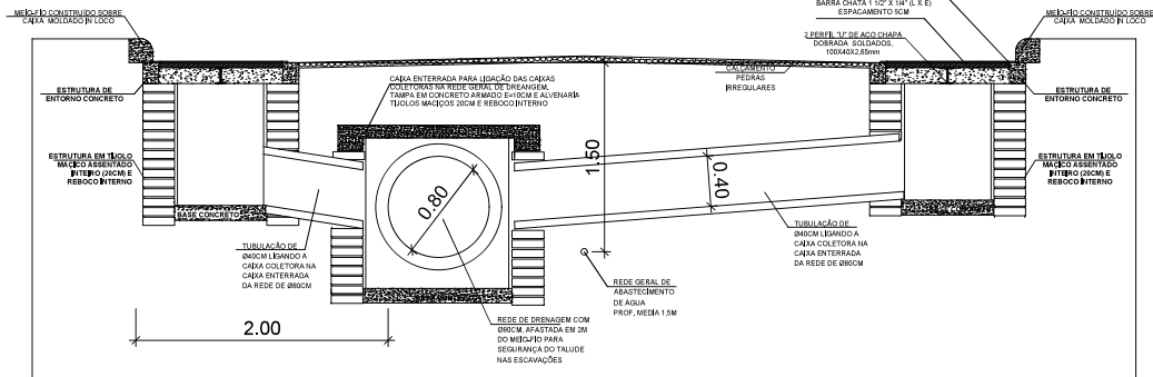
SEÇÃO TRANSVERSAL CAIXA ENTERRADA RUA EGBERTO S. DE MORAES ESC: S/ ESC
