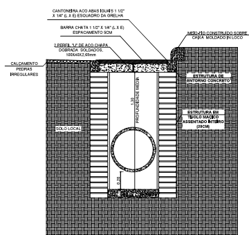
SEÇÃO TRANSVERSAL CAIXA ESC: S/ ESC
