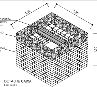
CAIXA COLETORA ESC: S/ ESC
