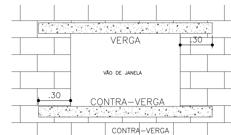
ESQUEMA DE MONTAGEM VERGA E CONTRA-VERGA SEM ESCALA
