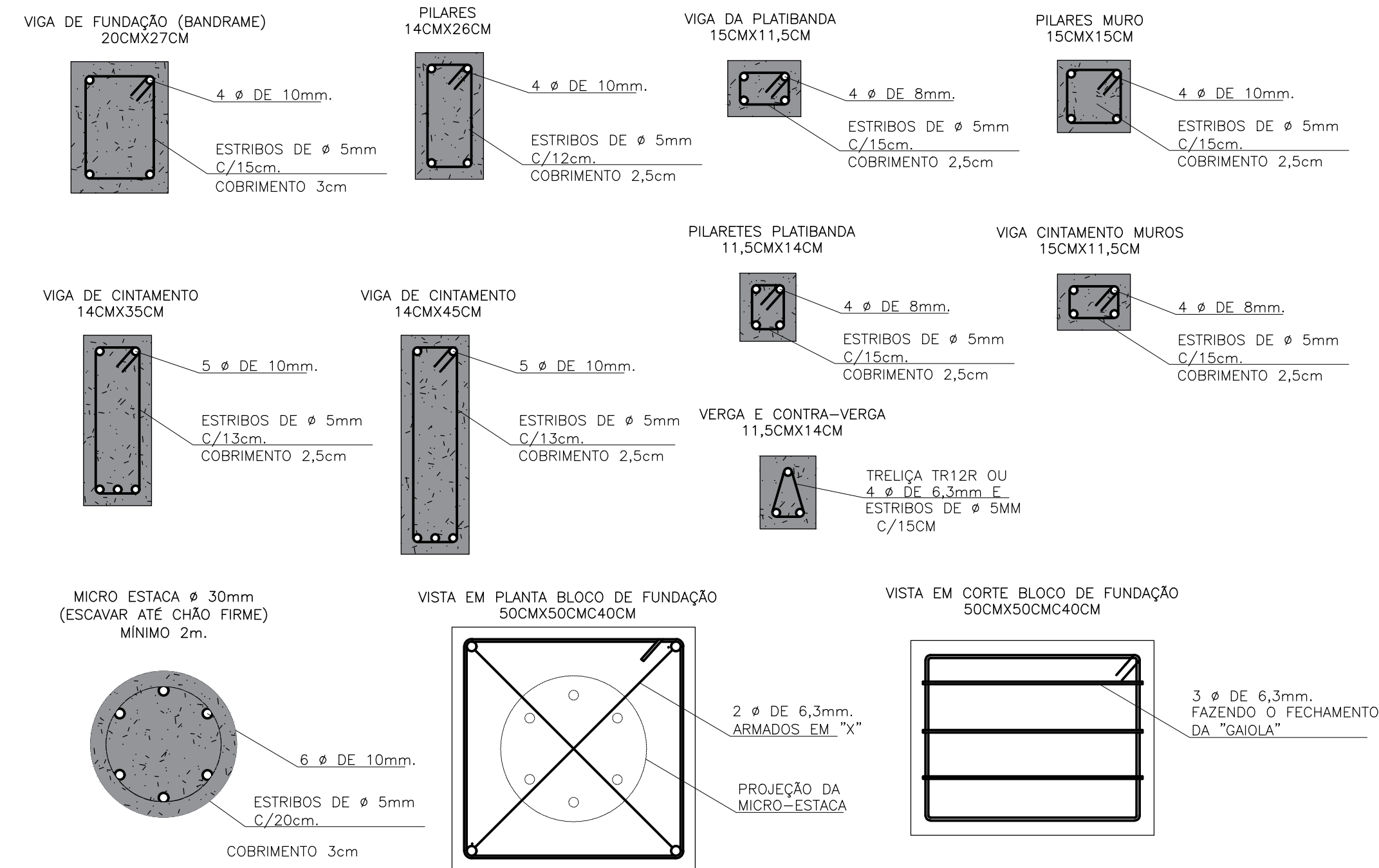
DETALHAMENTO PILARES – VIGAS E ESTACAS SEM ESCALA
